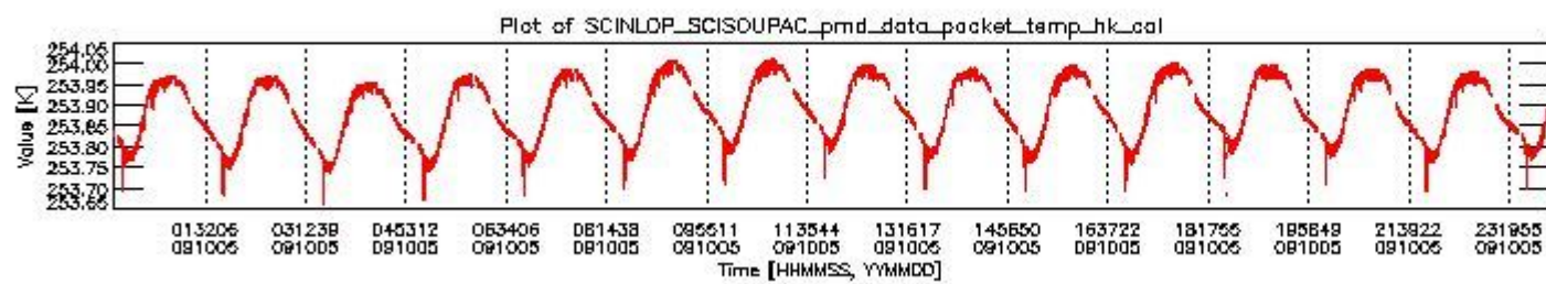
sciamachy_daily_report_level0_KSPT_L0_4303_N_20091005_3.PNG
