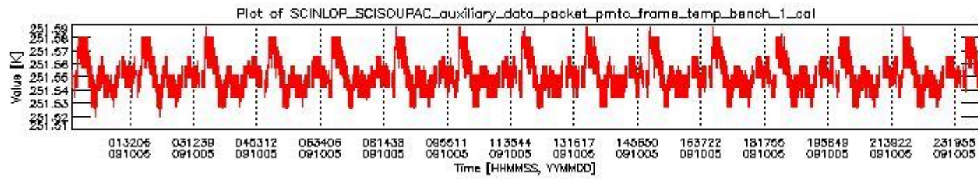
sciamachy_daily_report_level0_KSPT_L0_4303_N_20091005_0.PNG
