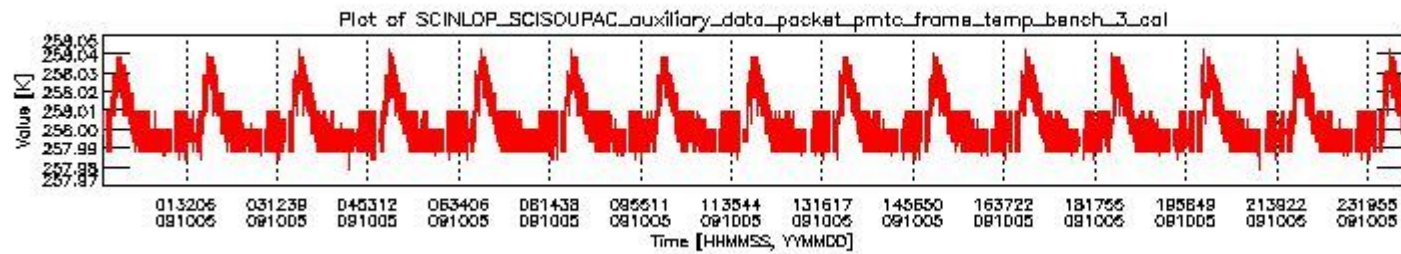
sciamachy_daily_report_level0_KSPT_L0_4303_N_20091005_2.PNG
