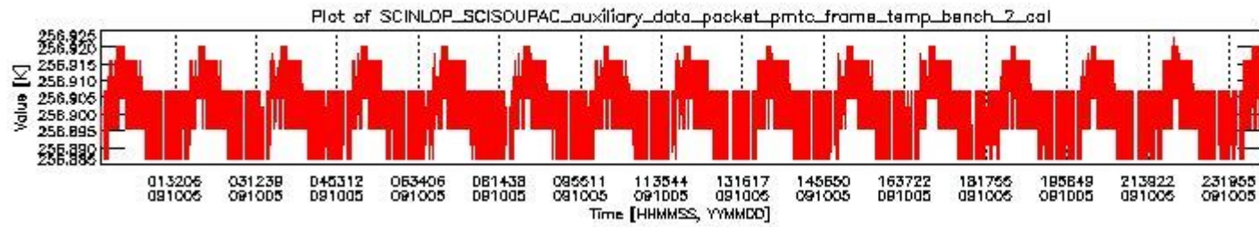
sciamachy_daily_report_level0_KSPT_L0_4303_N_20091005_1.PNG
