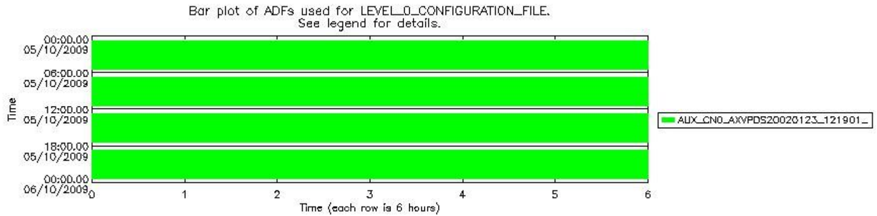
sciamachy_daily_report_level0_KSPT_L0_4303_N_20091005_6.PNG
