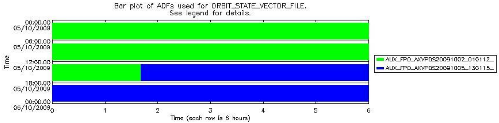
sciamachy_daily_report_level0_KSPT_L0_4303_N_20091005_7.PNG
