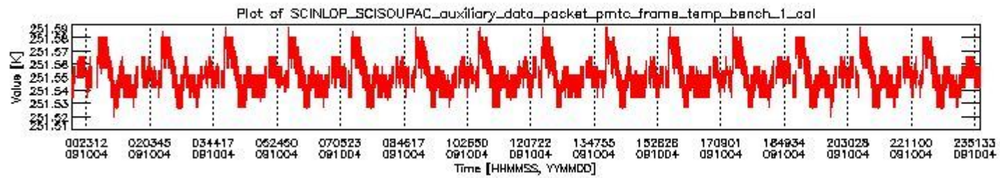
sciamachy_daily_report_level0_KSPT_L0_4303_N_20091004_0.PNG
