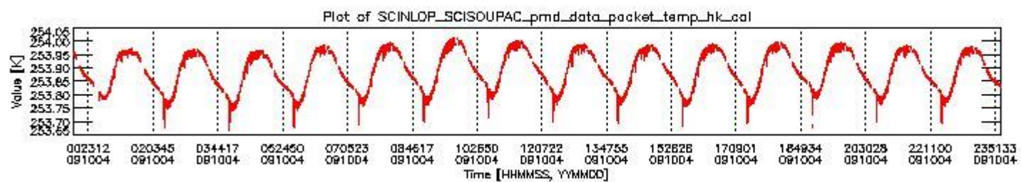
sciamachy_daily_report_level0_KSPT_L0_4303_N_20091004_3.PNG
