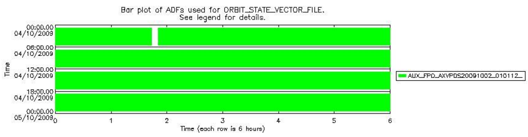
sciamachy_daily_report_level0_KSPT_L0_4303_N_20091004_7.PNG
