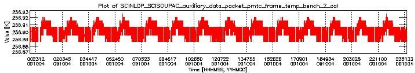
sciamachy_daily_report_level0_KSPT_L0_4303_N_20091004_1.PNG
