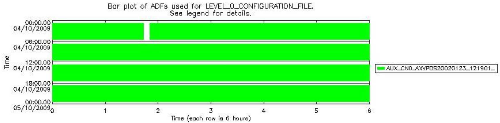
sciamachy_daily_report_level0_KSPT_L0_4303_N_20091004_6.PNG
