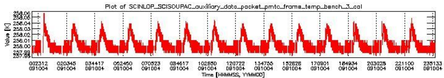
sciamachy_daily_report_level0_KSPT_L0_4303_N_20091004_2.PNG
