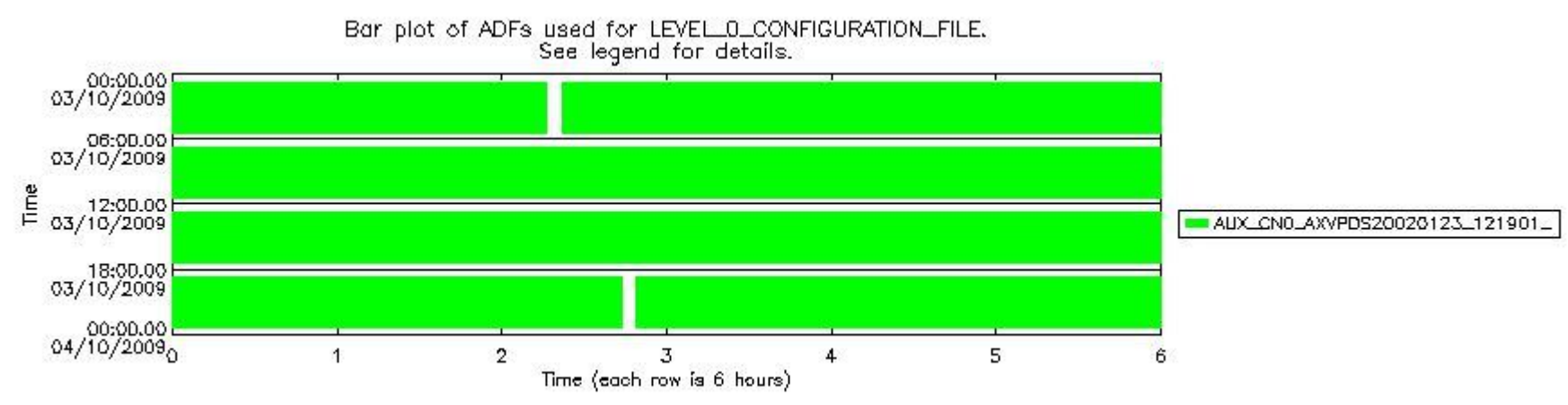
sciamachy_daily_report_level0_KSPT_L0_4303_N_20091003_6.PNG
