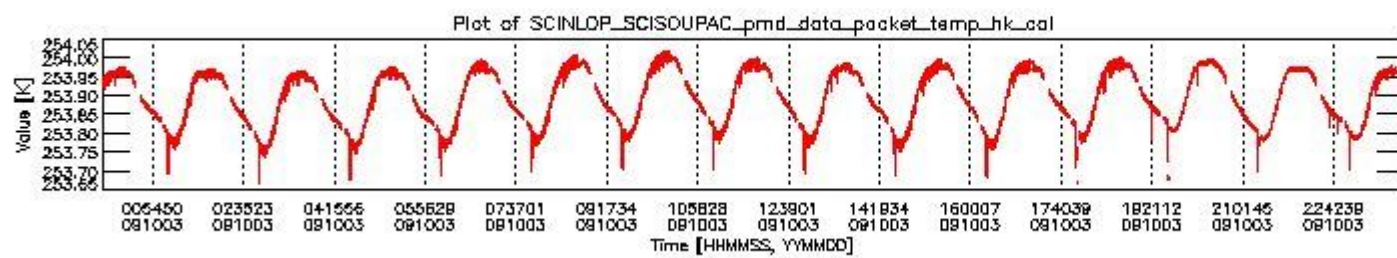
sciamachy_daily_report_level0_KSPT_L0_4303_N_20091003_3.PNG
