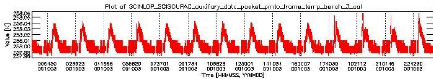
sciamachy_daily_report_level0_KSPT_L0_4303_N_20091003_2.PNG
