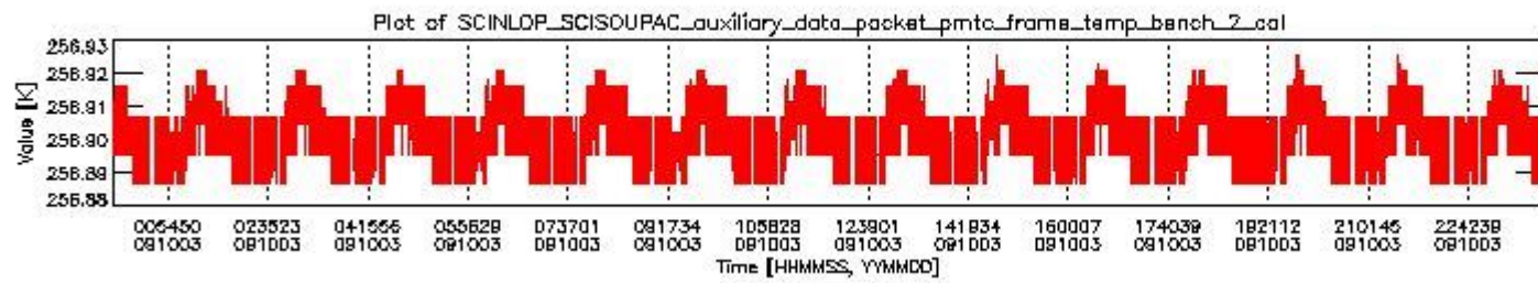
sciamachy_daily_report_level0_KSPT_L0_4303_N_20091003_1.PNG
