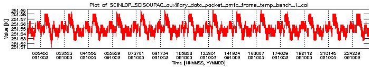
sciamachy_daily_report_level0_KSPT_L0_4303_N_20091003_0.PNG
