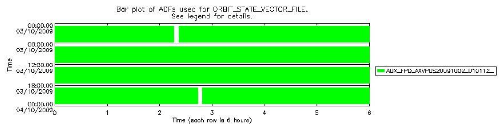
sciamachy_daily_report_level0_KSPT_L0_4303_N_20091003_7.PNG
