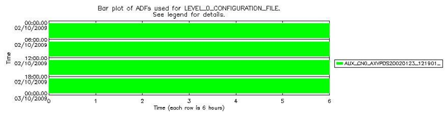
sciamachy_daily_report_level0_KSPT_L0_4303_N_20091002_6.PNG
