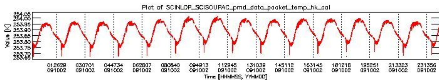
sciamachy_daily_report_level0_KSPT_L0_4303_N_20091002_3.PNG
