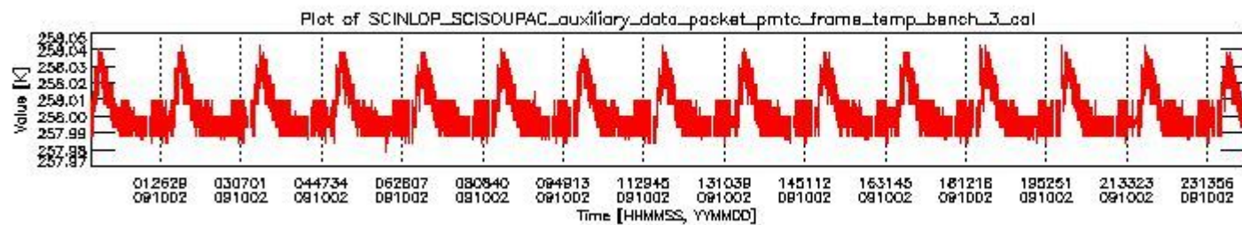
sciamachy_daily_report_level0_KSPT_L0_4303_N_20091002_2.PNG
