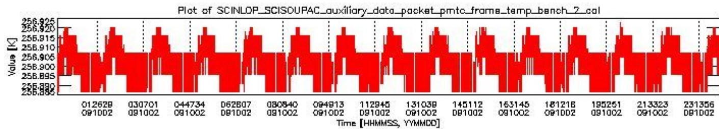
sciamachy_daily_report_level0_KSPT_L0_4303_N_20091002_1.PNG
