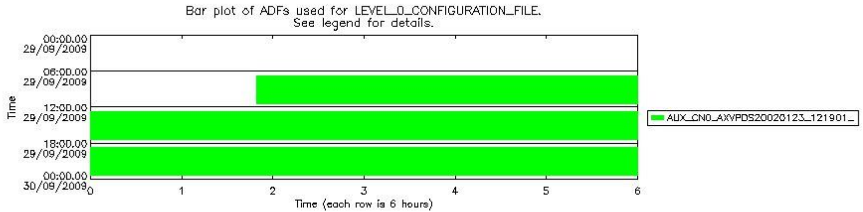
sciamachy_daily_report_level0_KSPT_L0_4303_N_20090929_6.PNG
