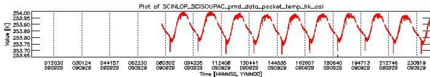
sciamachy_daily_report_level0_KSPT_L0_4303_N_20090929_3.PNG
