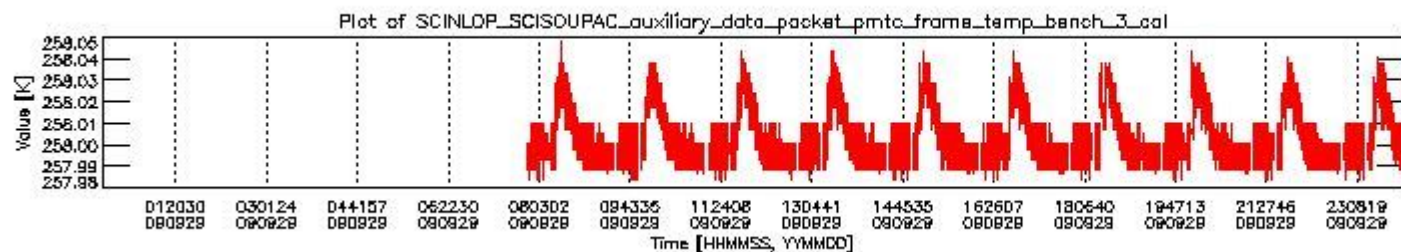
sciamachy_daily_report_level0_KSPT_L0_4303_N_20090929_2.PNG
