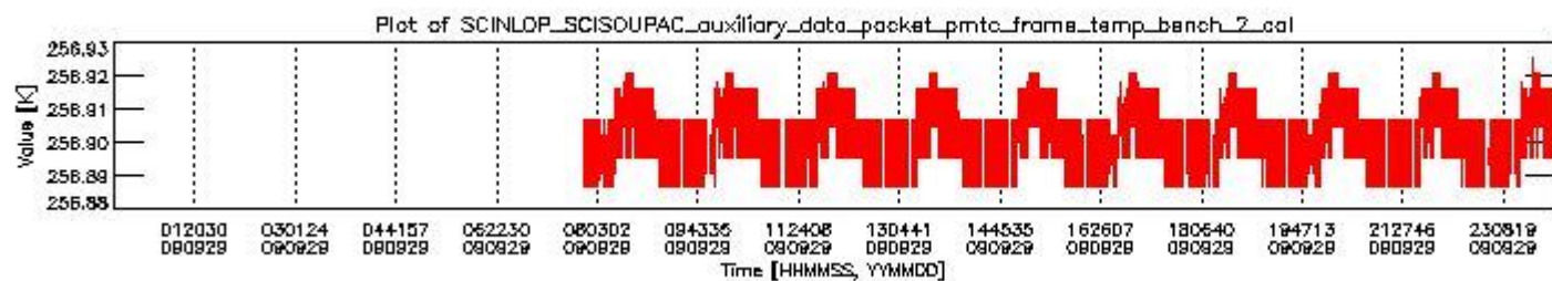
sciamachy_daily_report_level0_KSPT_L0_4303_N_20090929_1.PNG
