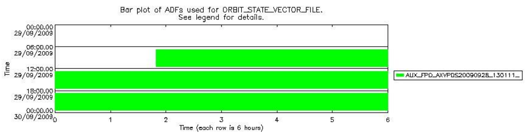
sciamachy_daily_report_level0_KSPT_L0_4303_N_20090929_7.PNG
