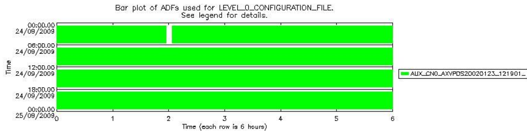
sciamachy_daily_report_level0_KSPT_L0_4303_N_20090924_6.PNG
