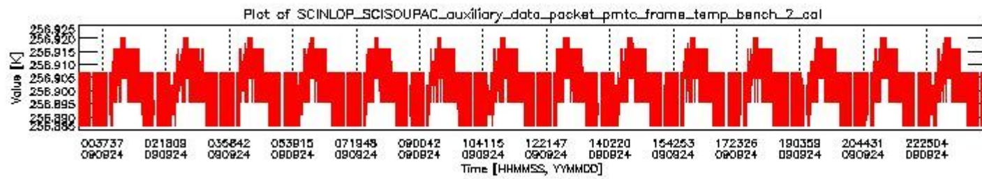
sciamachy_daily_report_level0_KSPT_L0_4303_N_20090924_1.PNG
