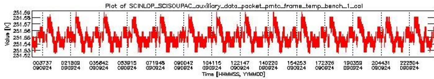
sciamachy_daily_report_level0_KSPT_L0_4303_N_20090924_0.PNG
