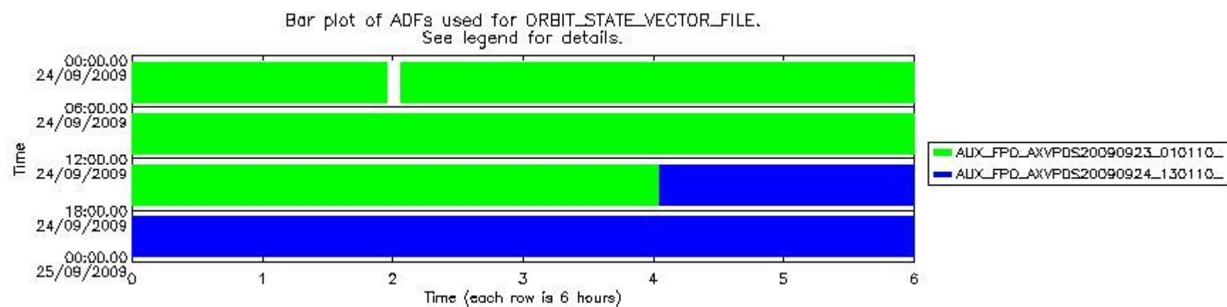
sciamachy_daily_report_level0_KSPT_L0_4303_N_20090924_7.PNG
