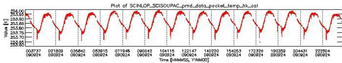
sciamachy_daily_report_level0_KSPT_L0_4303_N_20090924_3.PNG
