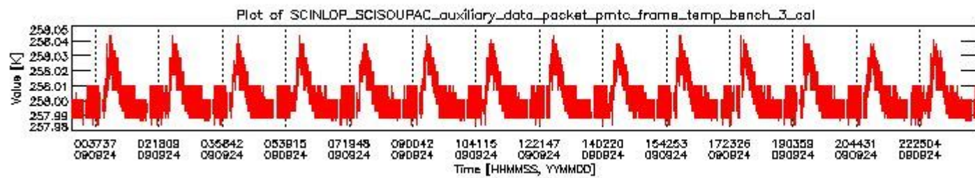
sciamachy_daily_report_level0_KSPT_L0_4303_N_20090924_2.PNG
