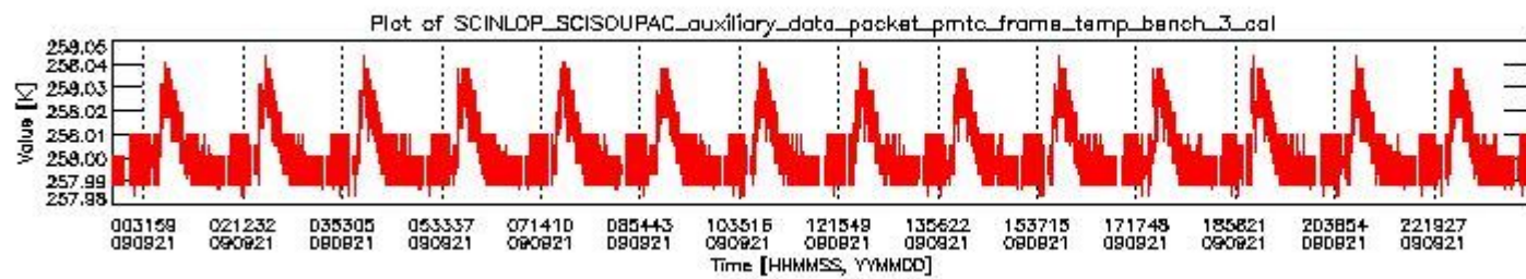
sciamachy_daily_report_level0_KSPT_L0_4303_N_20090921_2.PNG
