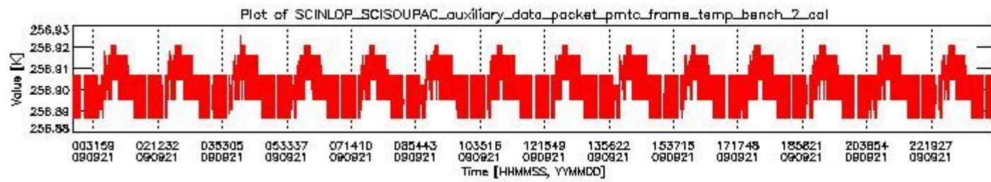
sciamachy_daily_report_level0_KSPT_L0_4303_N_20090921_1.PNG
