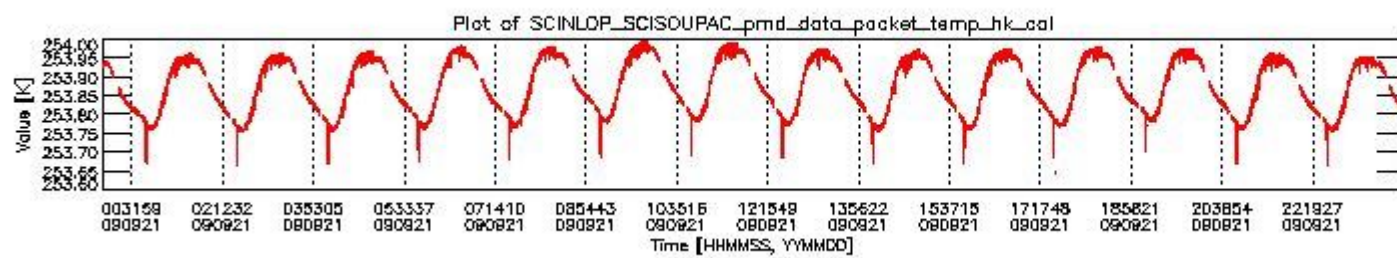
sciamachy_daily_report_level0_KSPT_L0_4303_N_20090921_3.PNG
