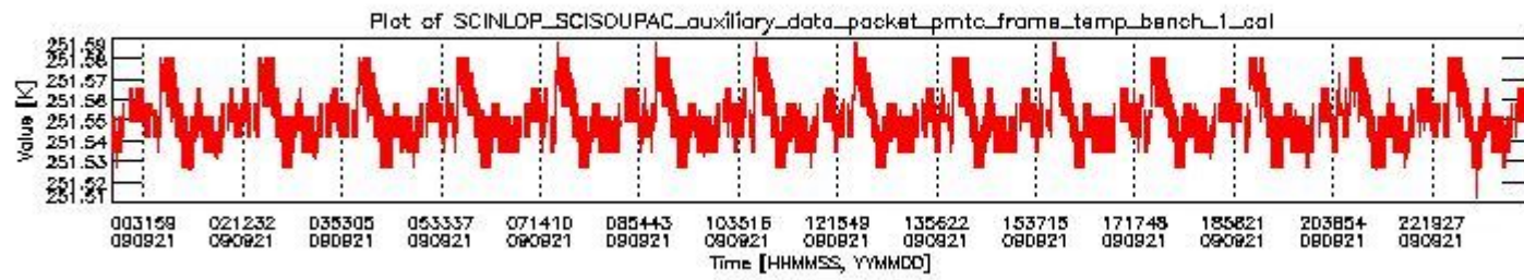
sciamachy_daily_report_level0_KSPT_L0_4303_N_20090921_0.PNG
