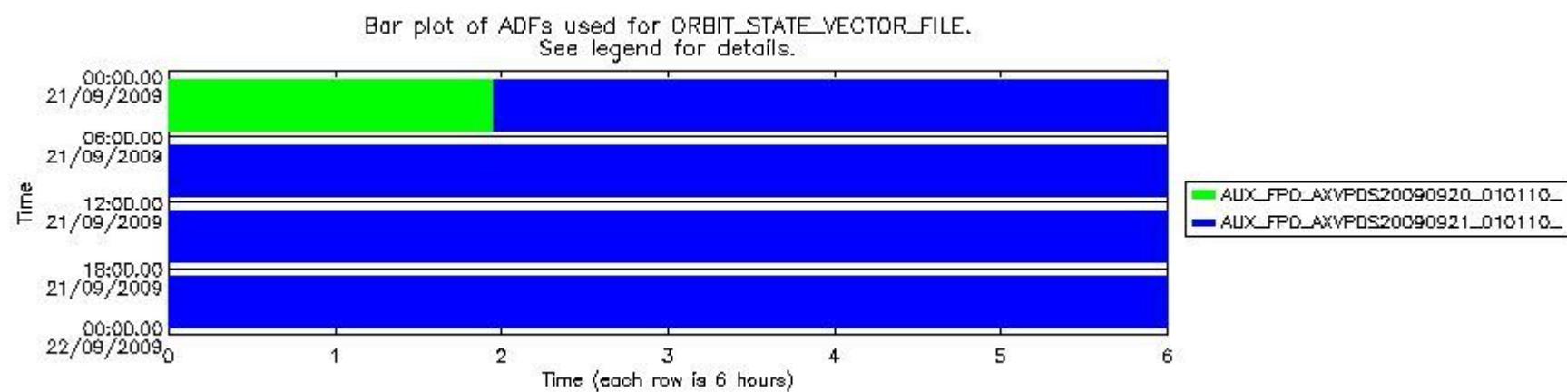
sciamachy_daily_report_level0_KSPT_L0_4303_N_20090921_7.PNG
