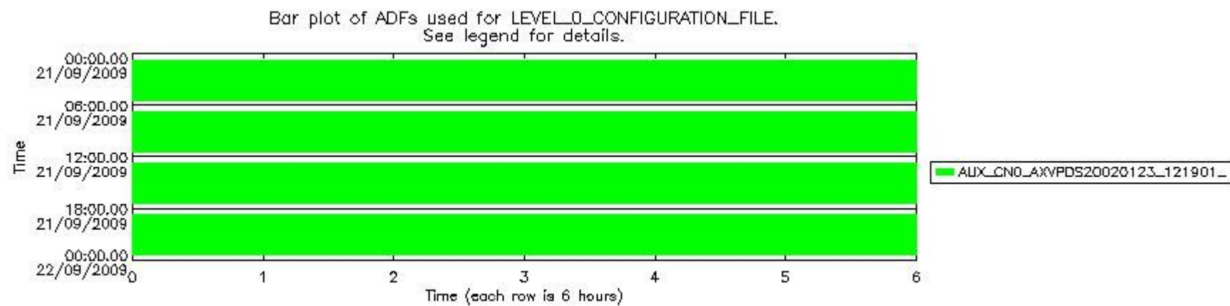
sciamachy_daily_report_level0_KSPT_L0_4303_N_20090921_6.PNG
