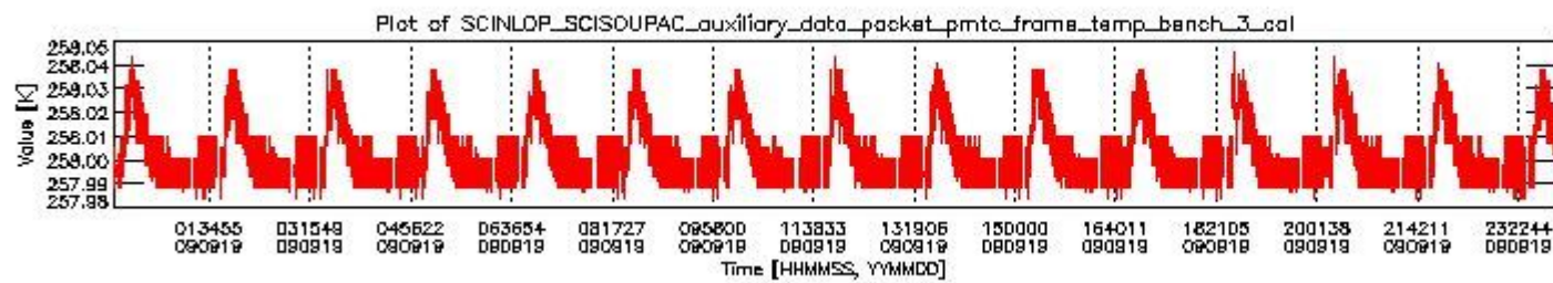
sciamachy_daily_report_level0_KSPT_L0_4303_N_20090919_2.PNG
