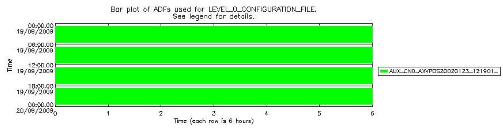
sciamachy_daily_report_level0_KSPT_L0_4303_N_20090919_6.PNG
