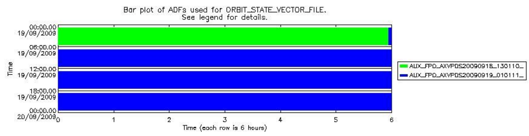
sciamachy_daily_report_level0_KSPT_L0_4303_N_20090919_7.PNG
