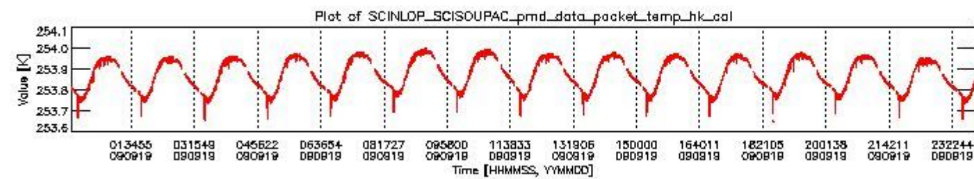
sciamachy_daily_report_level0_KSPT_L0_4303_N_20090919_3.PNG
