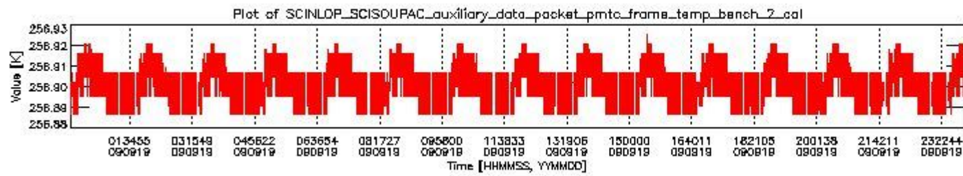
sciamachy_daily_report_level0_KSPT_L0_4303_N_20090919_1.PNG
