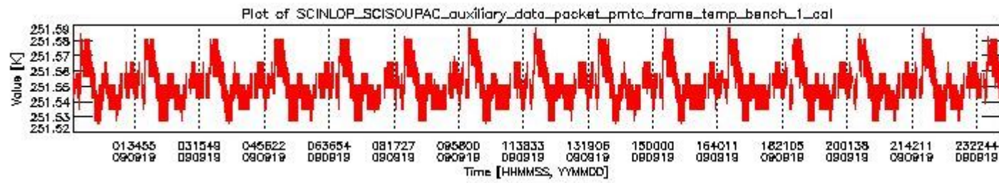
sciamachy_daily_report_level0_KSPT_L0_4303_N_20090919_0.PNG
