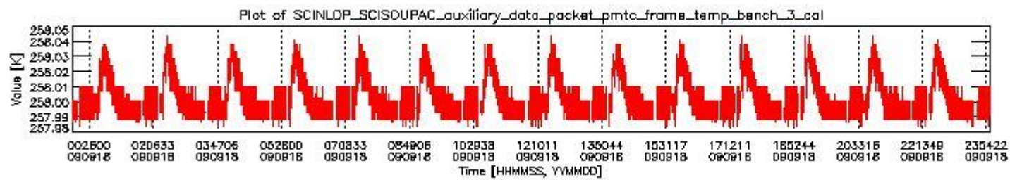
sciamachy_daily_report_level0_KSPT_L0_4303_N_20090918_2.PNG
