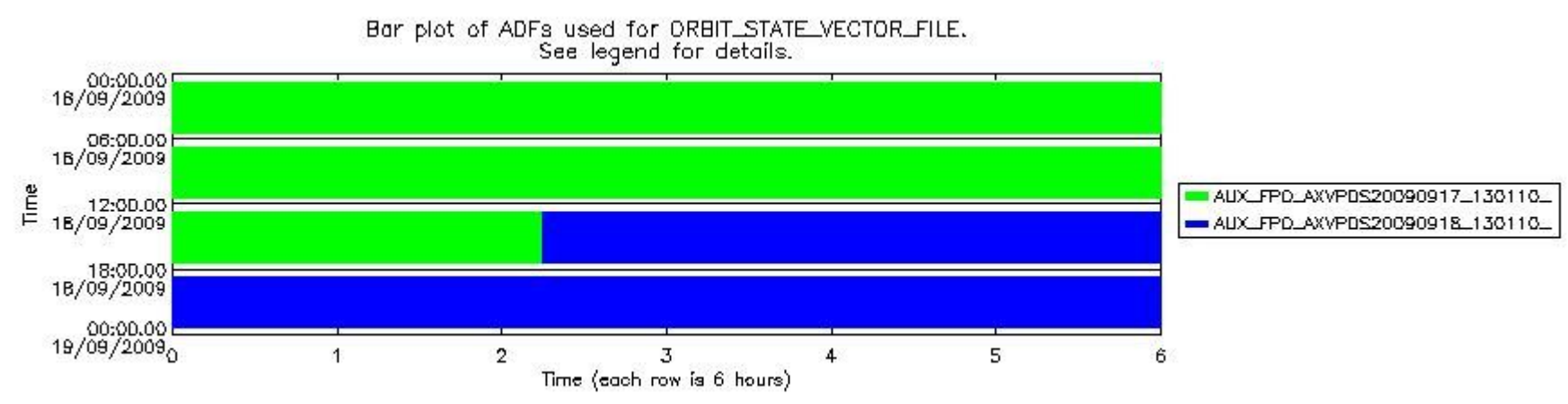
sciamachy_daily_report_level0_KSPT_L0_4303_N_20090918_7.PNG
