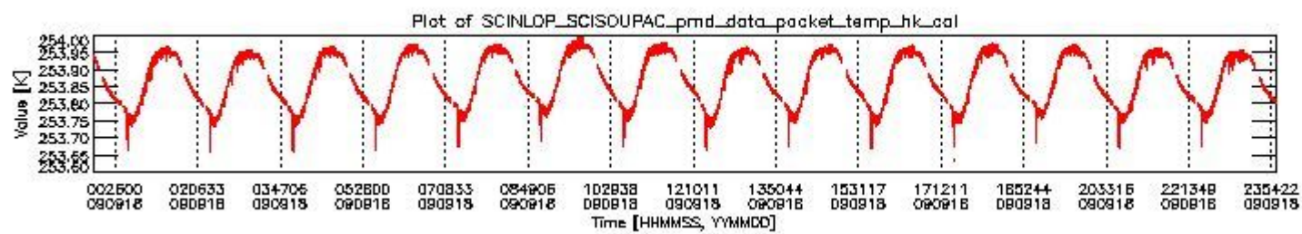
sciamachy_daily_report_level0_KSPT_L0_4303_N_20090918_3.PNG
