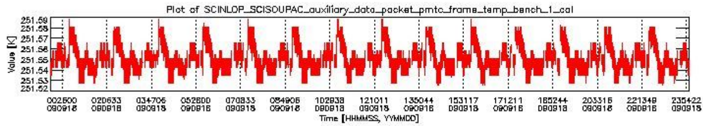
sciamachy_daily_report_level0_KSPT_L0_4303_N_20090918_0.PNG
