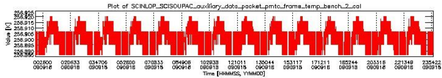
sciamachy_daily_report_level0_KSPT_L0_4303_N_20090918_1.PNG
