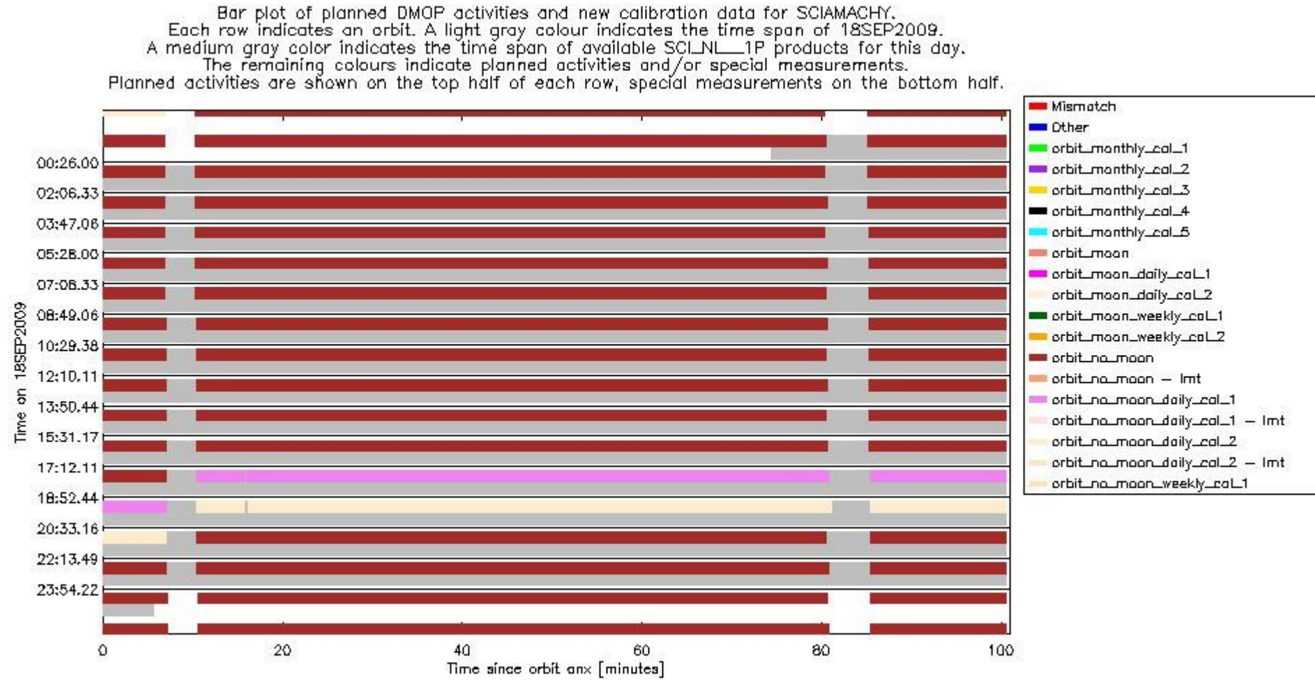
sciamachy_daily_report_level0_KSPT_L0_4303_N_20090918_5.PNG
