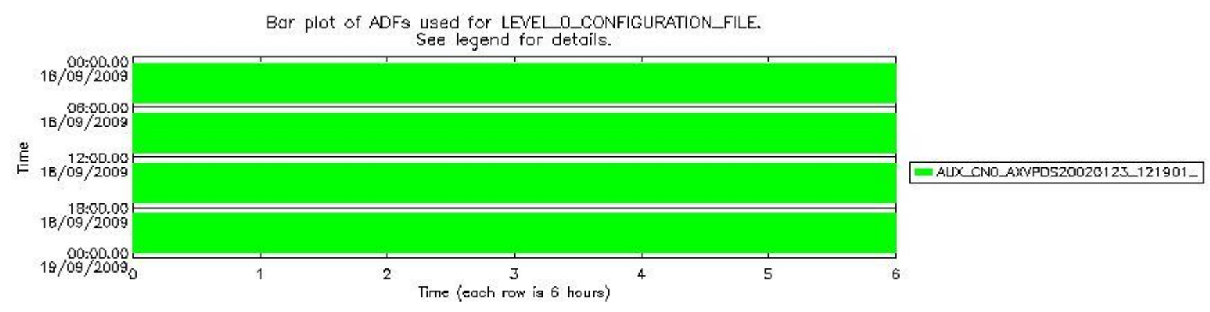
sciamachy_daily_report_level0_KSPT_L0_4303_N_20090918_6.PNG
