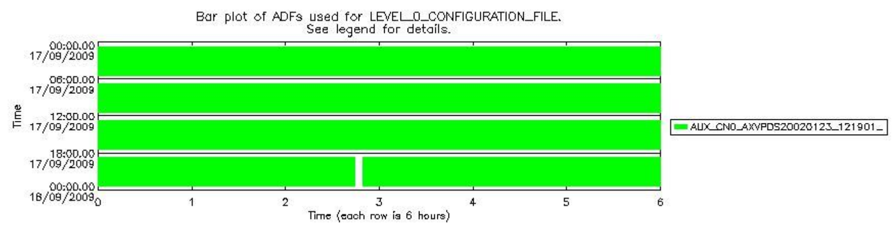
sciamachy_daily_report_level0_KSPT_L0_4303_N_20090917_6.PNG
