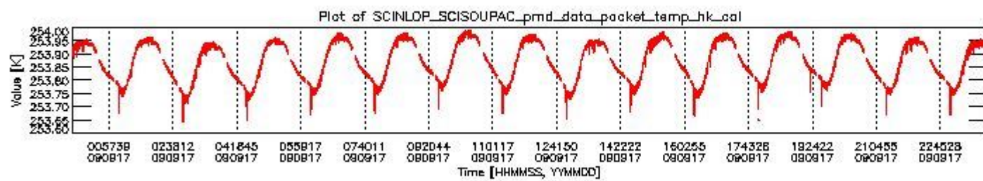
sciamachy_daily_report_level0_KSPT_L0_4303_N_20090917_3.PNG
