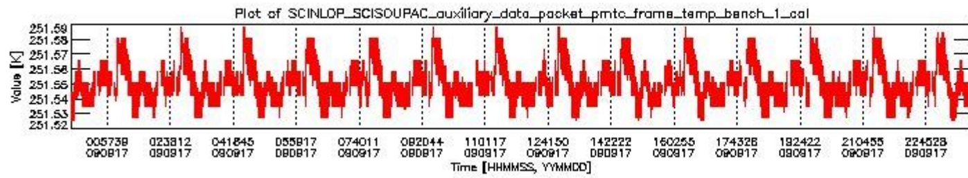
sciamachy_daily_report_level0_KSPT_L0_4303_N_20090917_0.PNG
