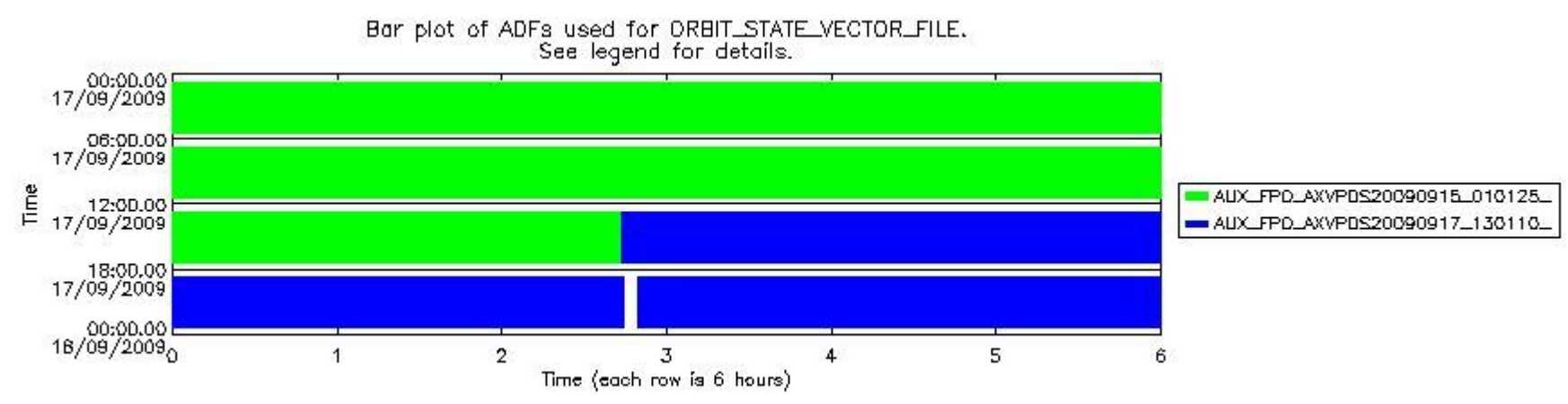
sciamachy_daily_report_level0_KSPT_L0_4303_N_20090917_7.PNG
