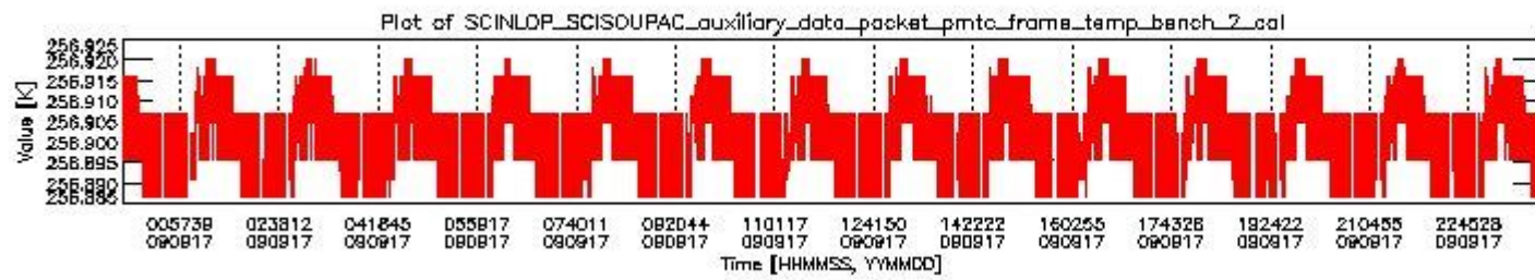
sciamachy_daily_report_level0_KSPT_L0_4303_N_20090917_1.PNG
