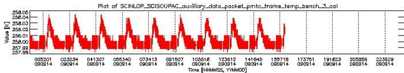
sciamachy_daily_report_level0_KSPT_L0_4303_N_20090914_2.PNG
