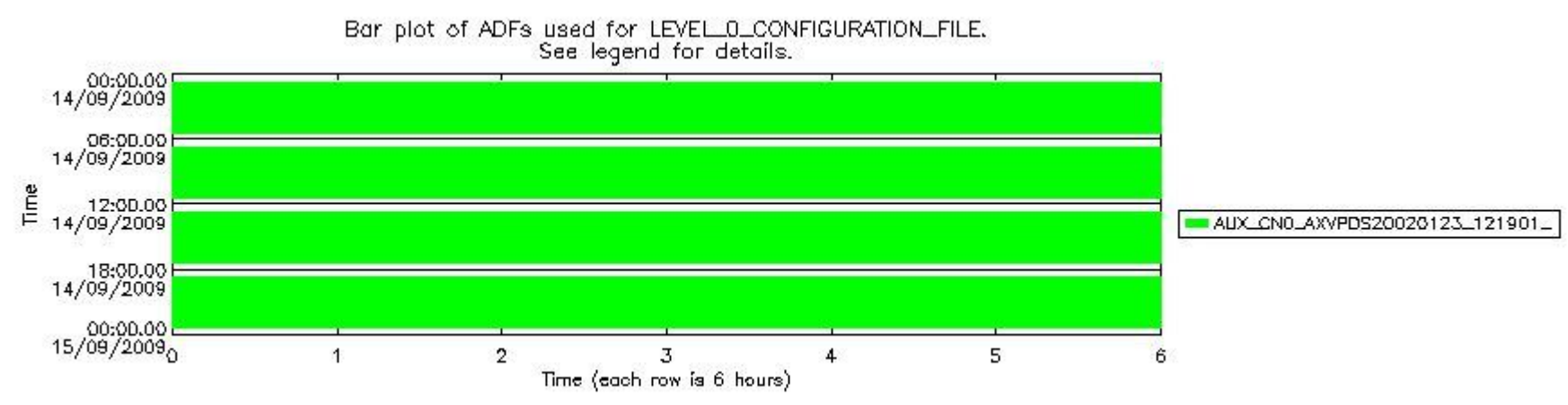
sciamachy_daily_report_level0_KSPT_L0_4303_N_20090914_6.PNG
