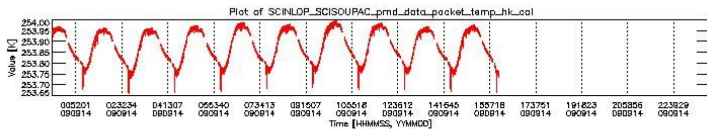
sciamachy_daily_report_level0_KSPT_L0_4303_N_20090914_3.PNG
