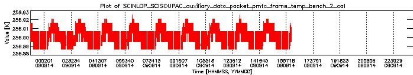
sciamachy_daily_report_level0_KSPT_L0_4303_N_20090914_1.PNG
