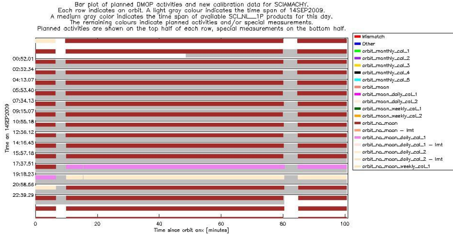
sciamachy_daily_report_level0_KSPT_L0_4303_N_20090914_5.PNG
