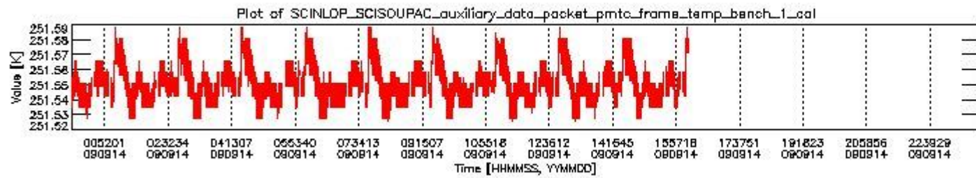
sciamachy_daily_report_level0_KSPT_L0_4303_N_20090914_0.PNG
