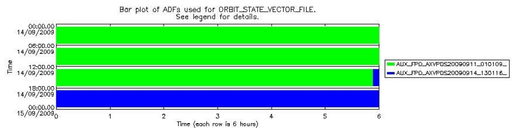
sciamachy_daily_report_level0_KSPT_L0_4303_N_20090914_7.PNG
