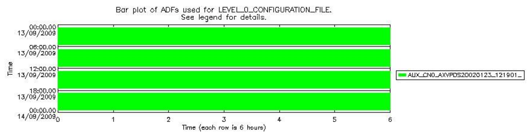
sciamachy_daily_report_level0_KSPT_L0_4303_N_20090913_6.PNG
