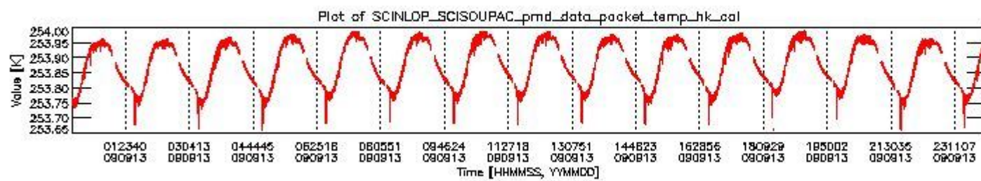
sciamachy_daily_report_level0_KSPT_L0_4303_N_20090913_3.PNG
