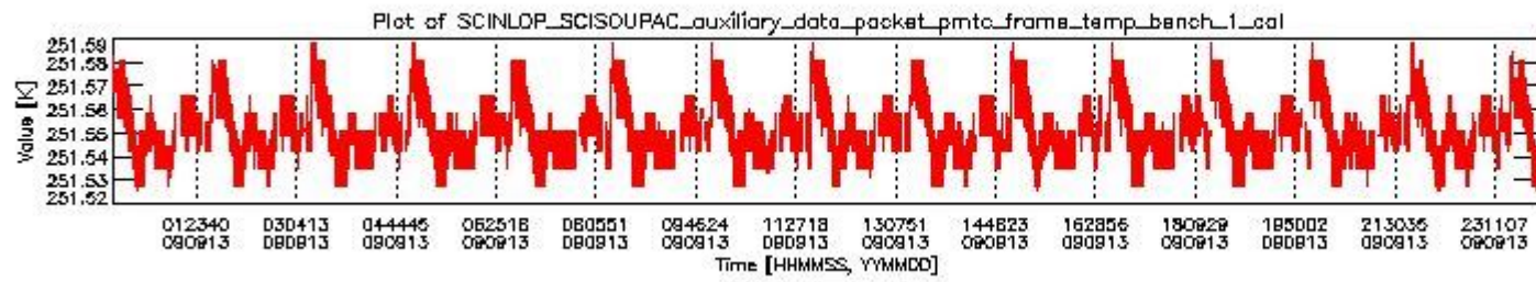
sciamachy_daily_report_level0_KSPT_L0_4303_N_20090913_0.PNG
