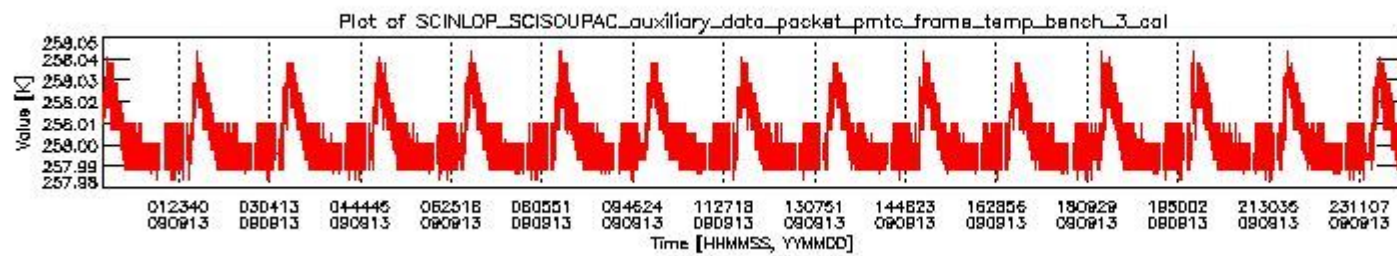
sciamachy_daily_report_level0_KSPT_L0_4303_N_20090913_2.PNG
