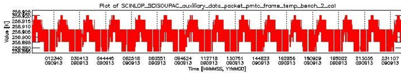
sciamachy_daily_report_level0_KSPT_L0_4303_N_20090913_1.PNG
