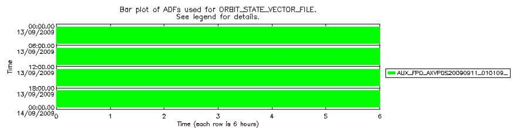
sciamachy_daily_report_level0_KSPT_L0_4303_N_20090913_7.PNG
