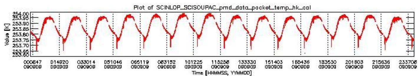
sciamachy_daily_report_level0_KSPT_L0_4303_N_20090909_3.PNG
