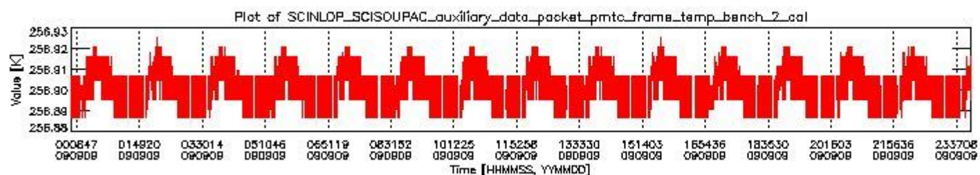
sciamachy_daily_report_level0_KSPT_L0_4303_N_20090909_1.PNG
