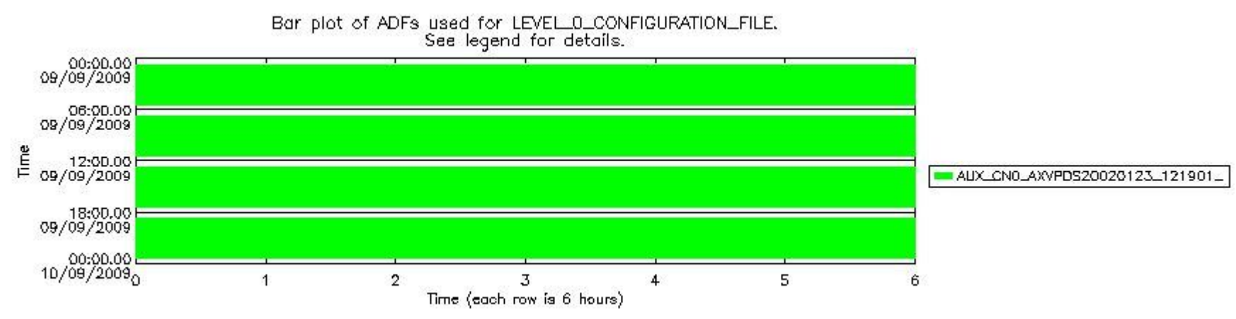
sciamachy_daily_report_level0_KSPT_L0_4303_N_20090909_6.PNG
