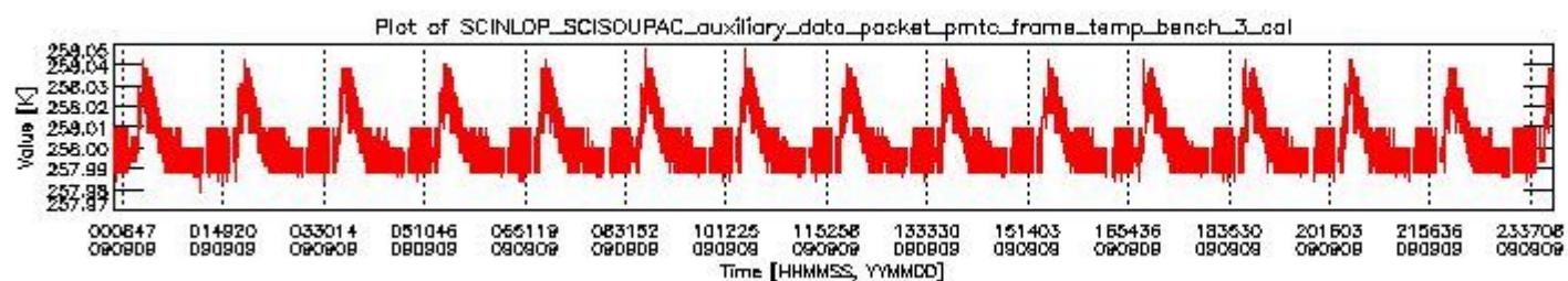
sciamachy_daily_report_level0_KSPT_L0_4303_N_20090909_2.PNG
