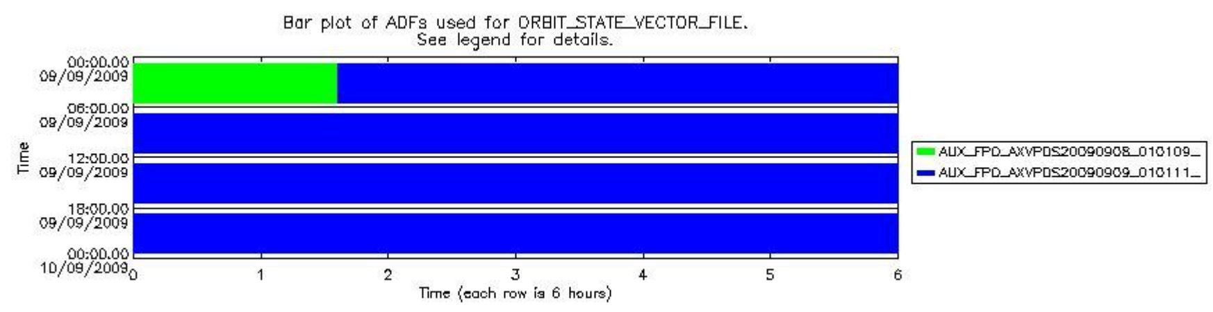
sciamachy_daily_report_level0_KSPT_L0_4303_N_20090909_7.PNG
