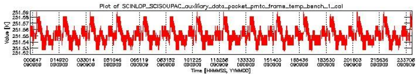
sciamachy_daily_report_level0_KSPT_L0_4303_N_20090909_0.PNG
