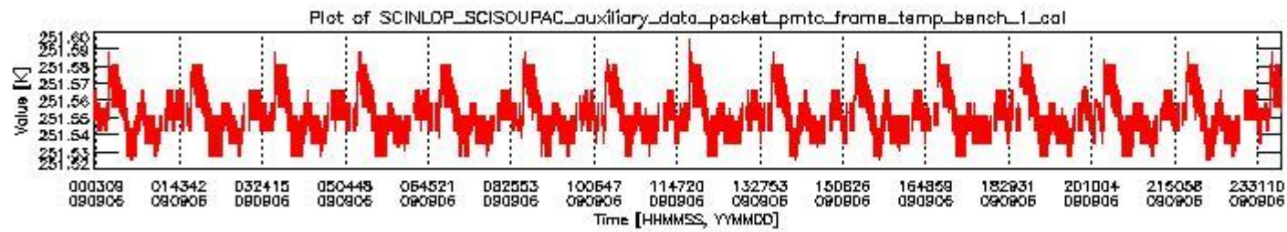
sciamachy_daily_report_level0_KSPT_L0_4303_N_20090906_0.PNG
