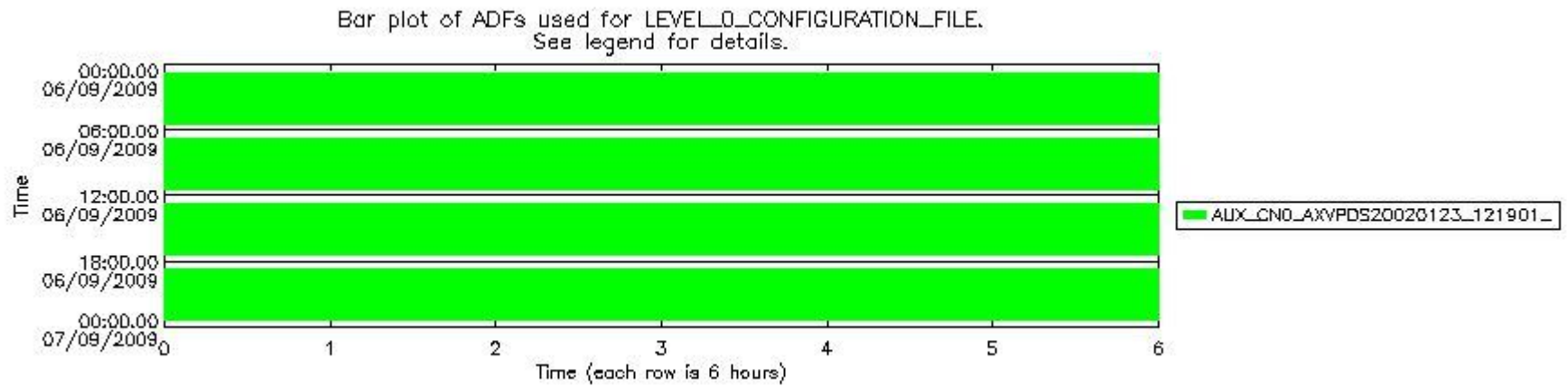
sciamachy_daily_report_level0_KSPT_L0_4303_N_20090906_6.PNG
