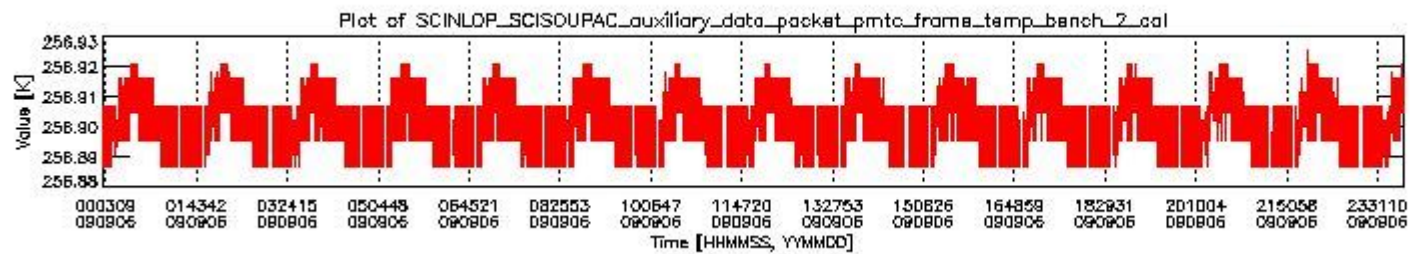
sciamachy_daily_report_level0_KSPT_L0_4303_N_20090906_1.PNG
