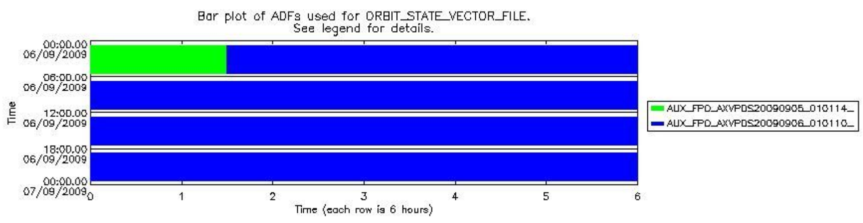
sciamachy_daily_report_level0_KSPT_L0_4303_N_20090906_7.PNG
