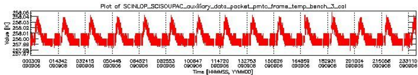
sciamachy_daily_report_level0_KSPT_L0_4303_N_20090906_2.PNG
