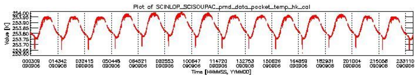
sciamachy_daily_report_level0_KSPT_L0_4303_N_20090906_3.PNG
