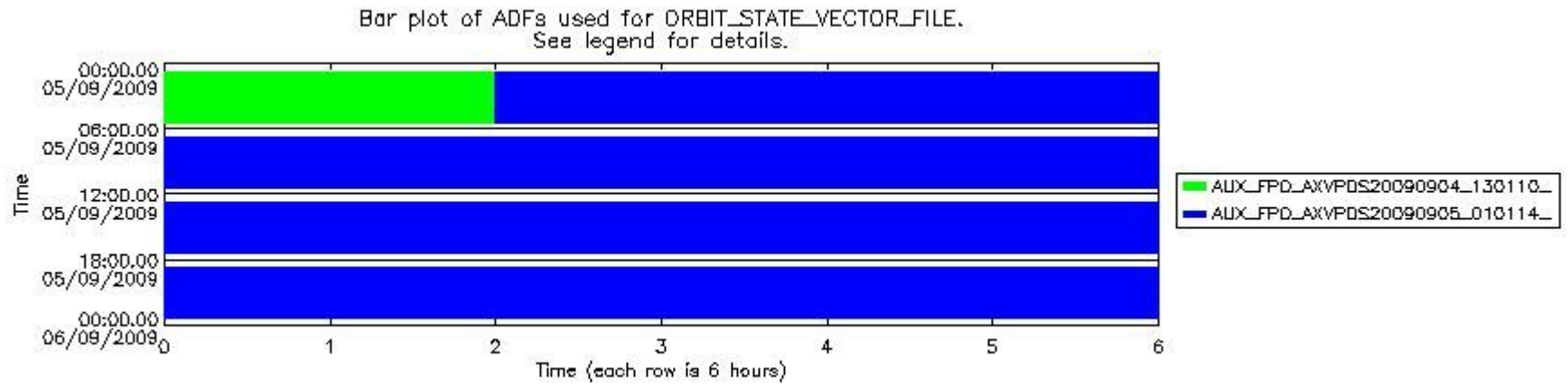
sciamachy_daily_report_level0_KSPT_L0_4303_N_20090905_7.PNG
