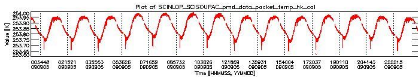
sciamachy_daily_report_level0_KSPT_L0_4303_N_20090905_3.PNG
