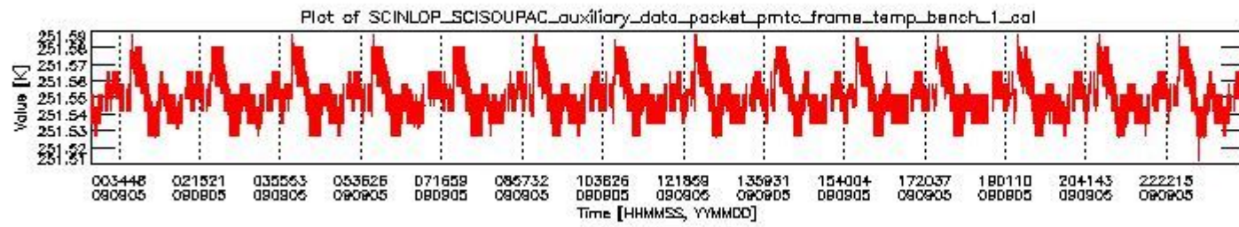
sciamachy_daily_report_level0_KSPT_L0_4303_N_20090905_0.PNG
