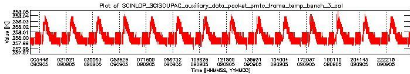
sciamachy_daily_report_level0_KSPT_L0_4303_N_20090905_2.PNG
