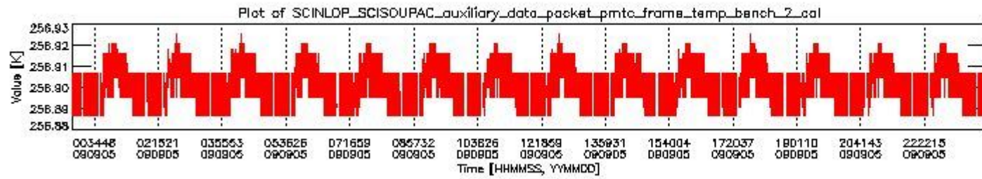
sciamachy_daily_report_level0_KSPT_L0_4303_N_20090905_1.PNG
