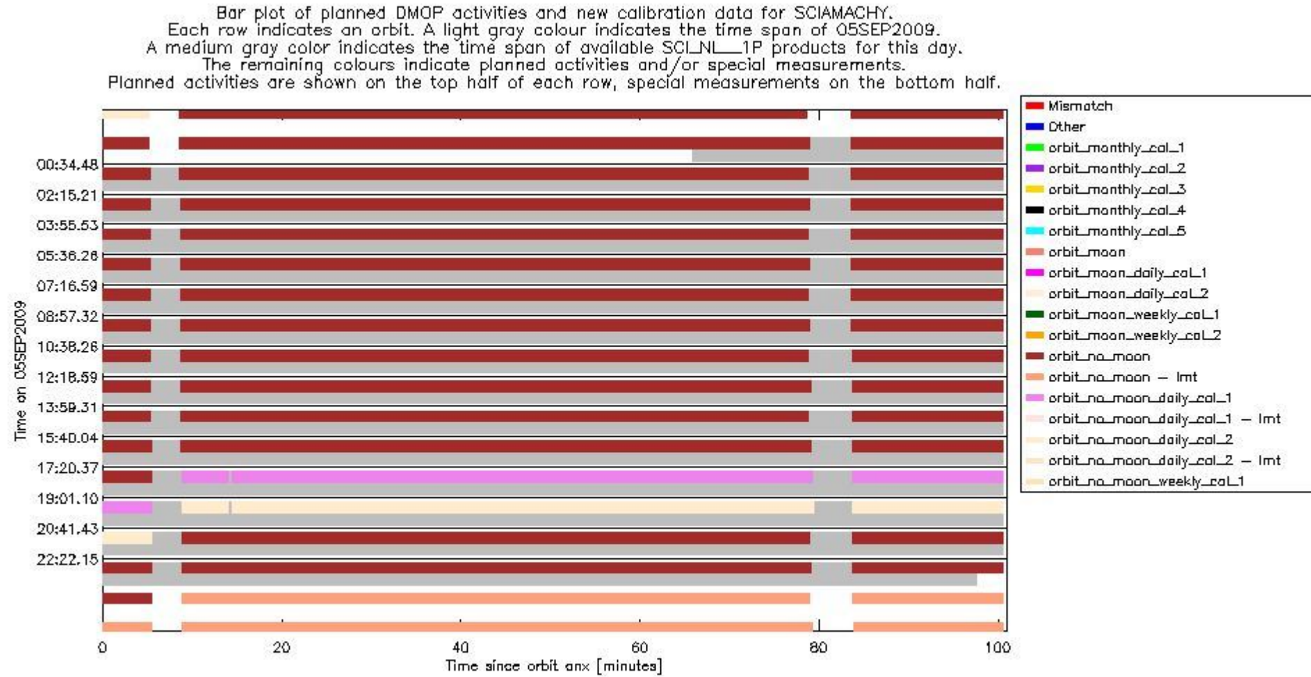
sciamachy_daily_report_level0_KSPT_L0_4303_N_20090905_5.PNG
