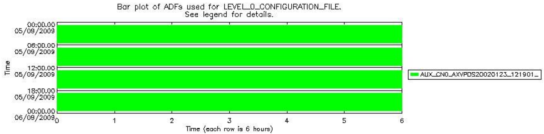
sciamachy_daily_report_level0_KSPT_L0_4303_N_20090905_6.PNG
