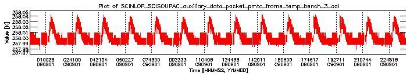
sciamachy_daily_report_level0_KSPT_L0_4303_N_20090901_2.PNG
