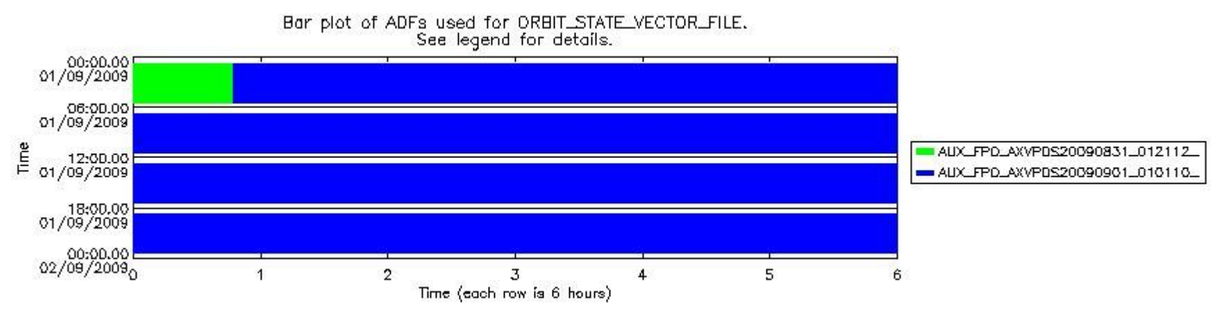
sciamachy_daily_report_level0_KSPT_L0_4303_N_20090901_7.PNG
