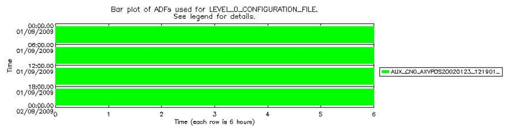
sciamachy_daily_report_level0_KSPT_L0_4303_N_20090901_6.PNG
