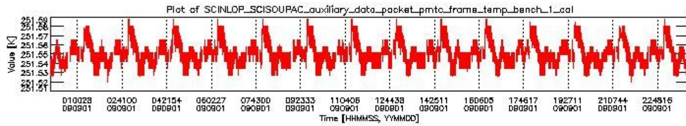
sciamachy_daily_report_level0_KSPT_L0_4303_N_20090901_0.PNG
