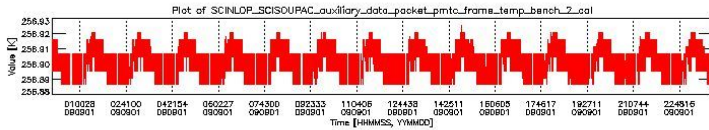
sciamachy_daily_report_level0_KSPT_L0_4303_N_20090901_1.PNG
