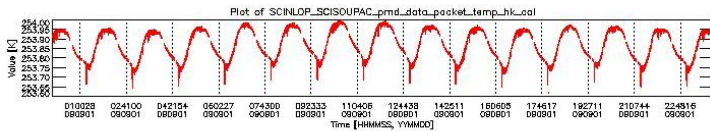
sciamachy_daily_report_level0_KSPT_L0_4303_N_20090901_3.PNG
