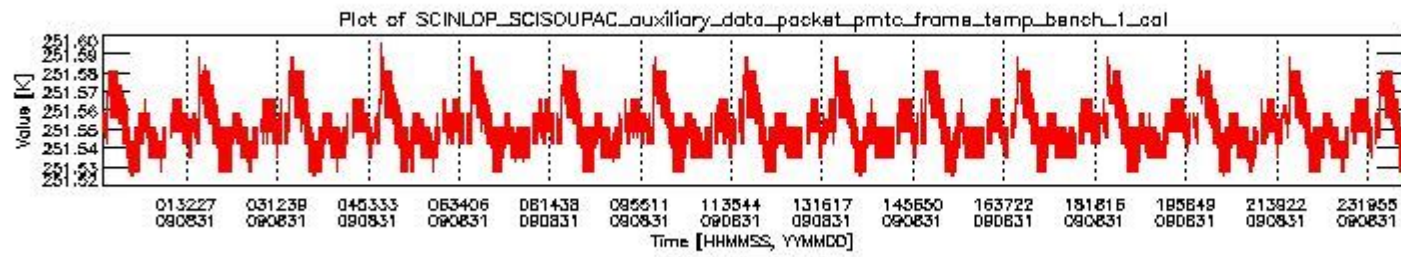
sciamachy_daily_report_level0_KSPT_L0_4303_N_20090831_0.PNG
