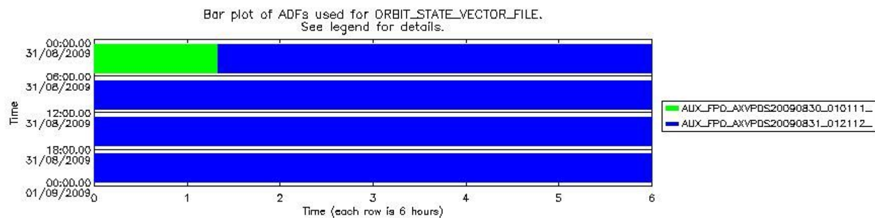
sciamachy_daily_report_level0_KSPT_L0_4303_N_20090831_7.PNG
