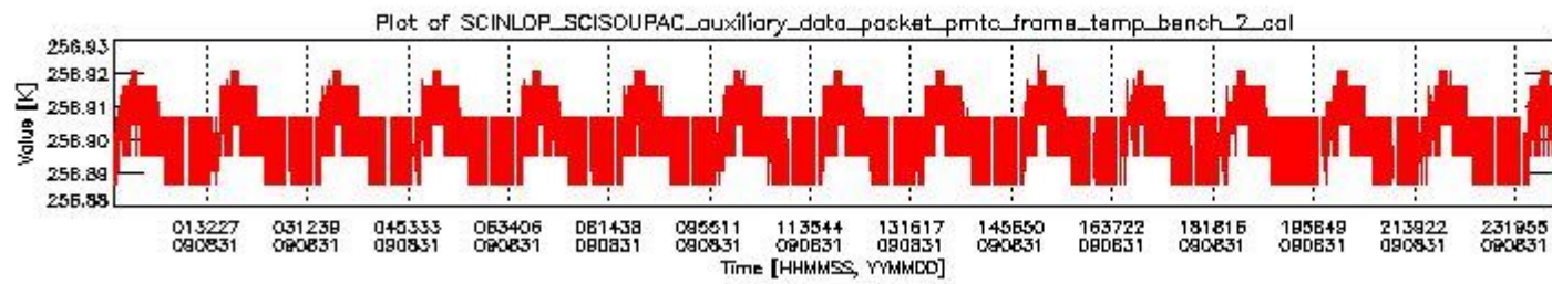
sciamachy_daily_report_level0_KSPT_L0_4303_N_20090831_1.PNG
