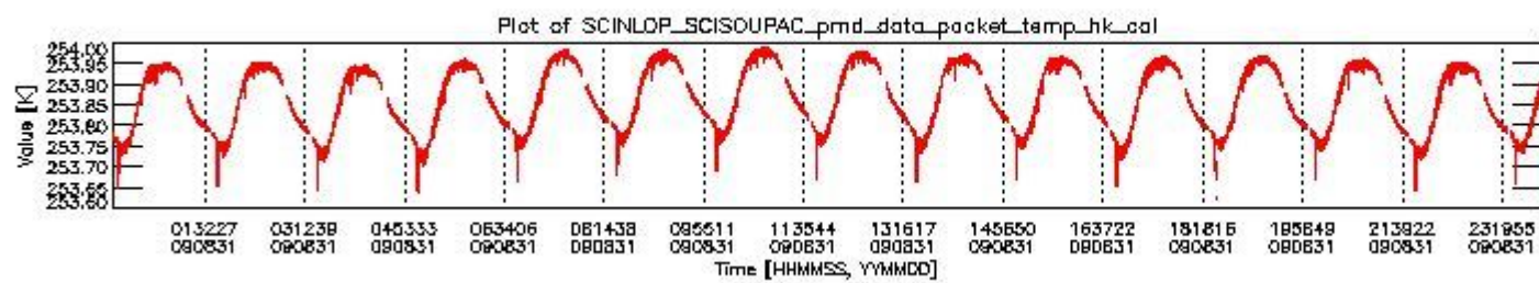
sciamachy_daily_report_level0_KSPT_L0_4303_N_20090831_3.PNG
