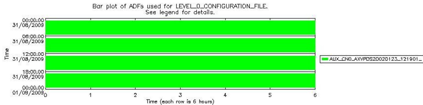
sciamachy_daily_report_level0_KSPT_L0_4303_N_20090831_6.PNG
