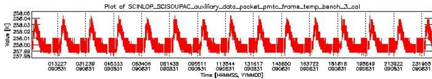
sciamachy_daily_report_level0_KSPT_L0_4303_N_20090831_2.PNG
