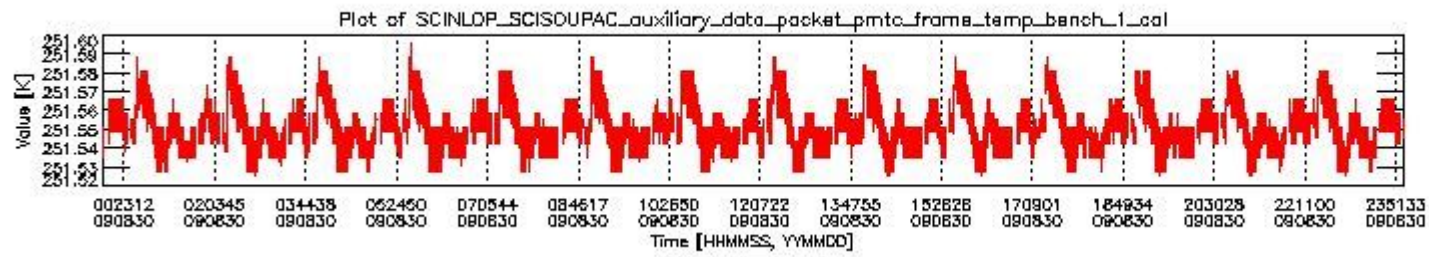
sciamachy_daily_report_level0_KSPT_L0_4303_N_20090830_0.PNG
