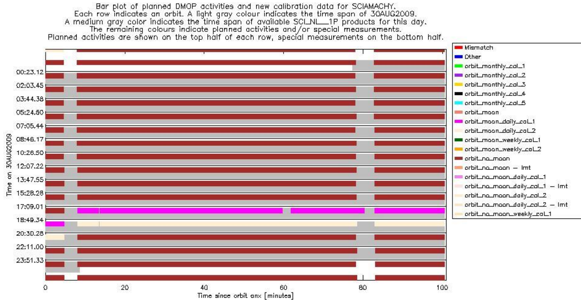
sciamachy_daily_report_level0_KSPT_L0_4303_N_20090830_5.PNG
