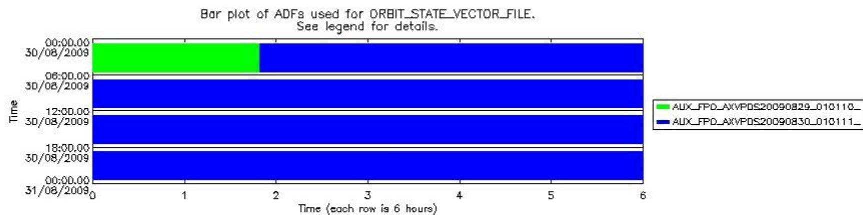
sciamachy_daily_report_level0_KSPT_L0_4303_N_20090830_7.PNG
