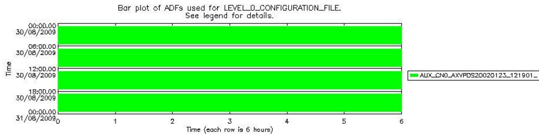
sciamachy_daily_report_level0_KSPT_L0_4303_N_20090830_6.PNG
