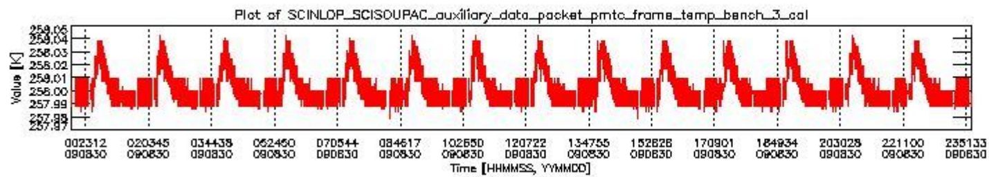
sciamachy_daily_report_level0_KSPT_L0_4303_N_20090830_2.PNG
