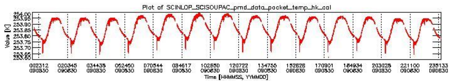
sciamachy_daily_report_level0_KSPT_L0_4303_N_20090830_3.PNG
