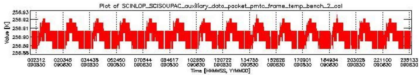
sciamachy_daily_report_level0_KSPT_L0_4303_N_20090830_1.PNG
