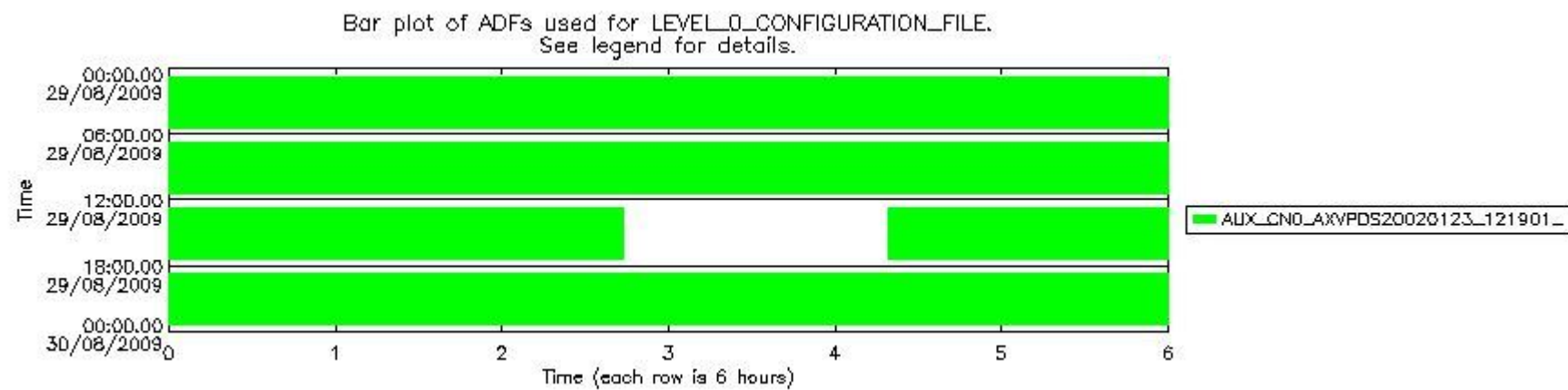
sciamachy_daily_report_level0_KSPT_L0_4303_N_20090829_6.PNG
