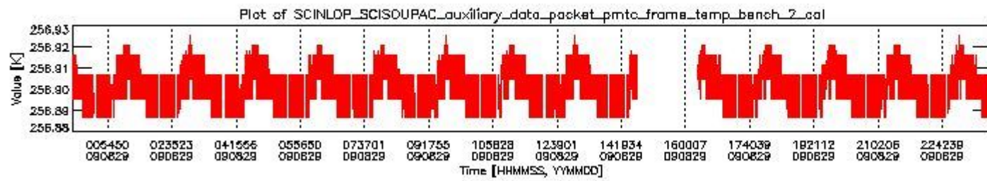
sciamachy_daily_report_level0_KSPT_L0_4303_N_20090829_1.PNG
