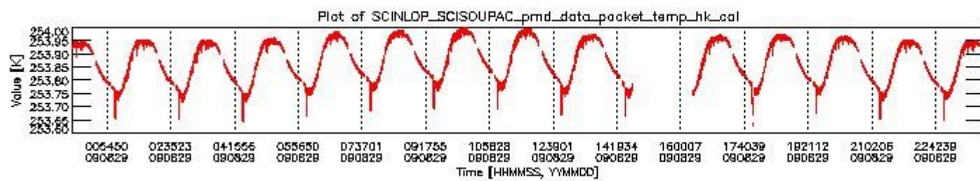
sciamachy_daily_report_level0_KSPT_L0_4303_N_20090829_3.PNG
