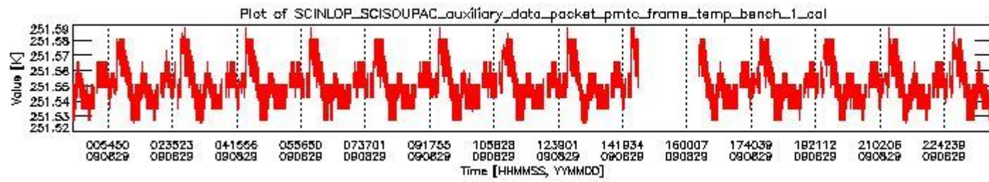
sciamachy_daily_report_level0_KSPT_L0_4303_N_20090829_0.PNG
