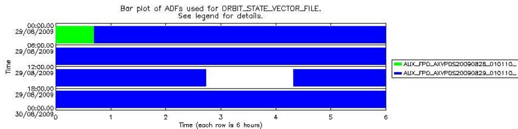
sciamachy_daily_report_level0_KSPT_L0_4303_N_20090829_7.PNG
