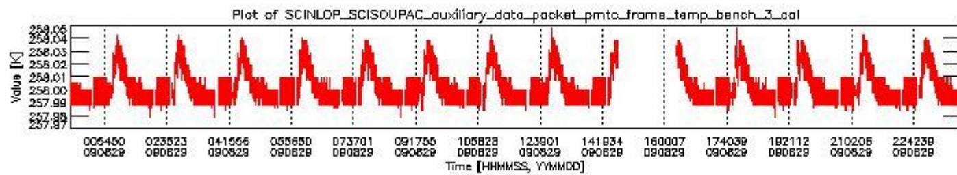
sciamachy_daily_report_level0_KSPT_L0_4303_N_20090829_2.PNG
