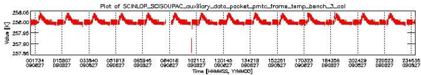
sciamachy_daily_report_level0_KSPT_L0_4303_N_20090827_2.PNG
