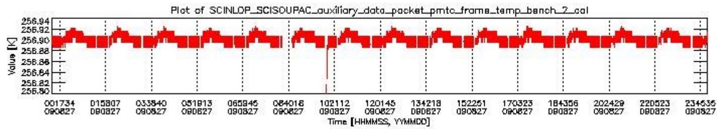
sciamachy_daily_report_level0_KSPT_L0_4303_N_20090827_1.PNG
