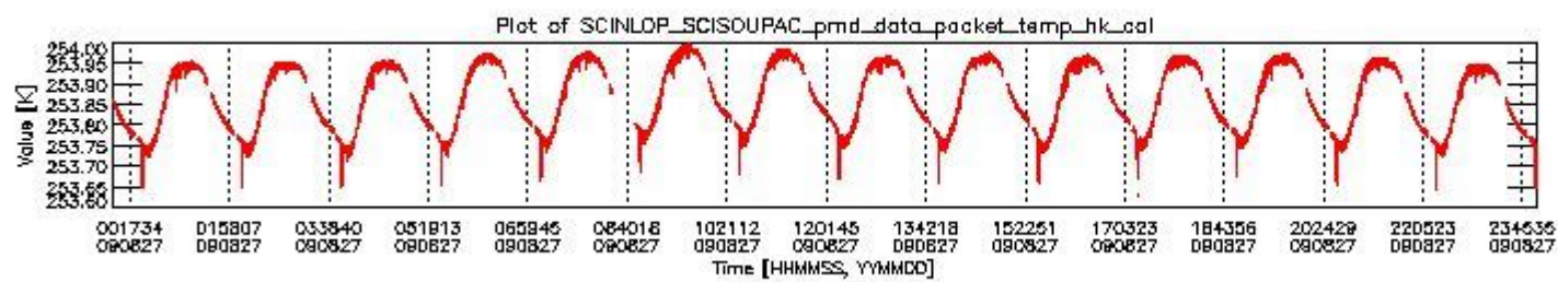
sciamachy_daily_report_level0_KSPT_L0_4303_N_20090827_3.PNG
