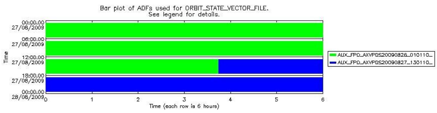
sciamachy_daily_report_level0_KSPT_L0_4303_N_20090827_7.PNG
