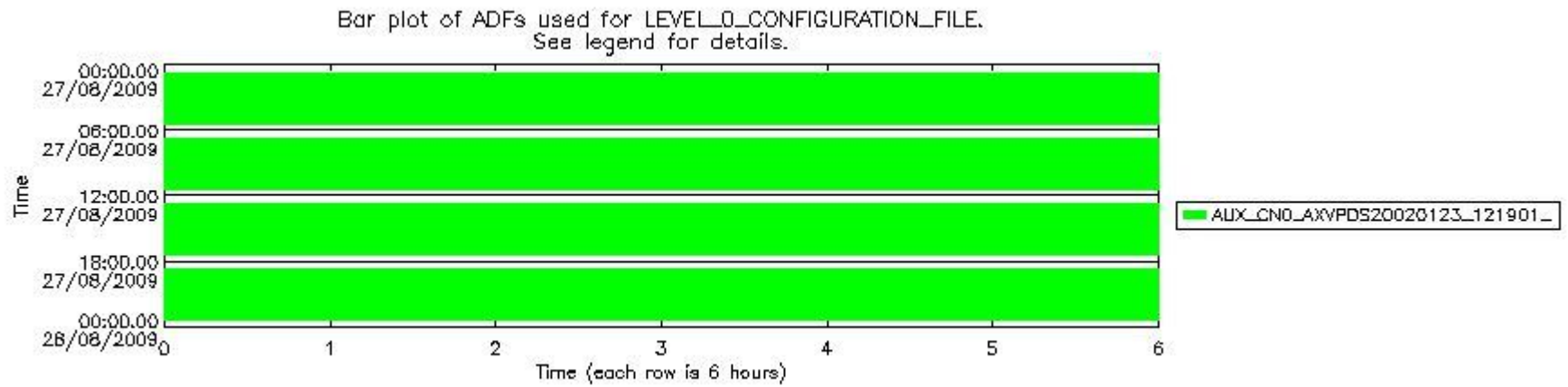
sciamachy_daily_report_level0_KSPT_L0_4303_N_20090827_6.PNG
