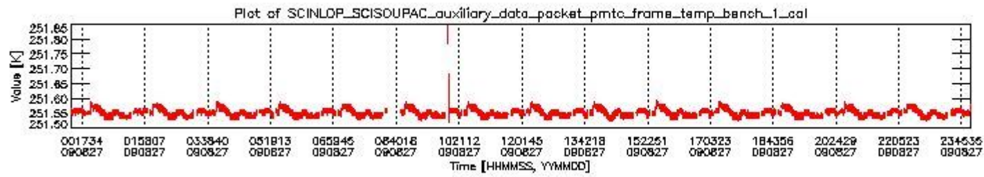
sciamachy_daily_report_level0_KSPT_L0_4303_N_20090827_0.PNG
