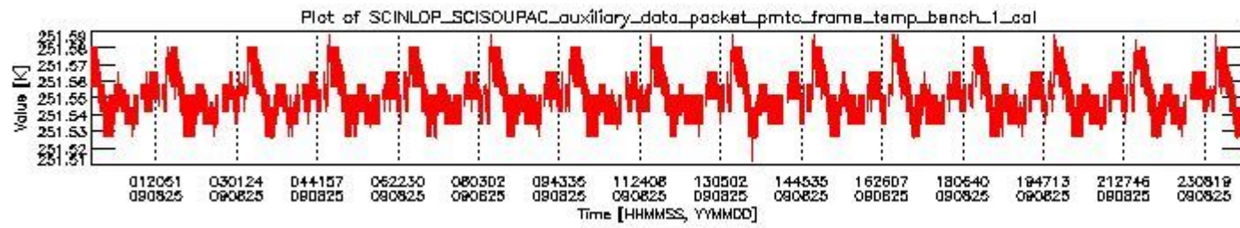
sciamachy_daily_report_level0_KSPT_L0_4303_N_20090825_0.PNG
