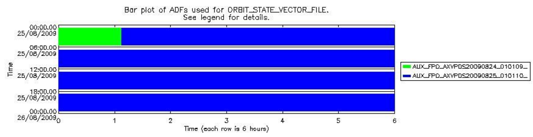
sciamachy_daily_report_level0_KSPT_L0_4303_N_20090825_7.PNG
