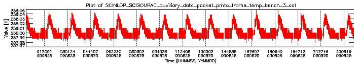
sciamachy_daily_report_level0_KSPT_L0_4303_N_20090825_2.PNG
