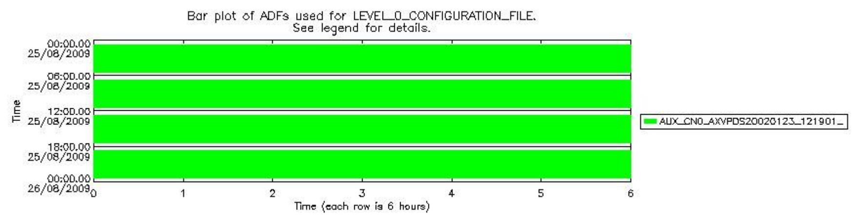
sciamachy_daily_report_level0_KSPT_L0_4303_N_20090825_6.PNG
