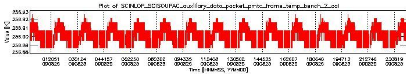
sciamachy_daily_report_level0_KSPT_L0_4303_N_20090825_1.PNG
