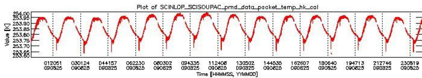
sciamachy_daily_report_level0_KSPT_L0_4303_N_20090825_3.PNG
