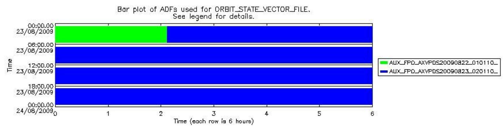
sciamachy_daily_report_level0_KSPT_L0_4303_N_20090823_7.PNG
