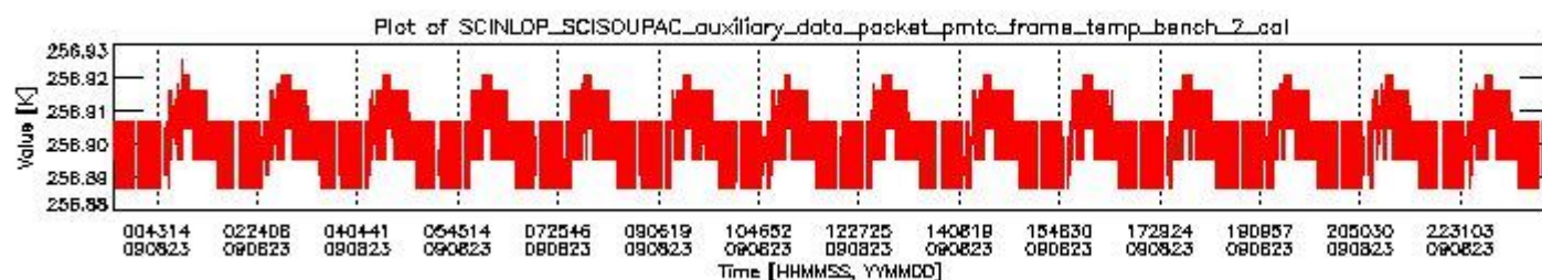
sciamachy_daily_report_level0_KSPT_L0_4303_N_20090823_1.PNG
