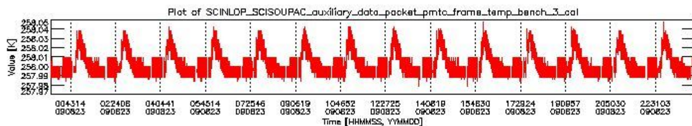
sciamachy_daily_report_level0_KSPT_L0_4303_N_20090823_2.PNG
