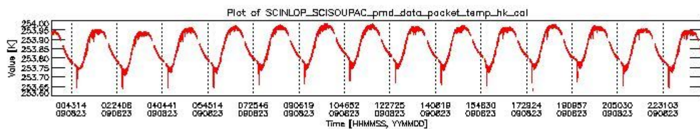
sciamachy_daily_report_level0_KSPT_L0_4303_N_20090823_3.PNG
