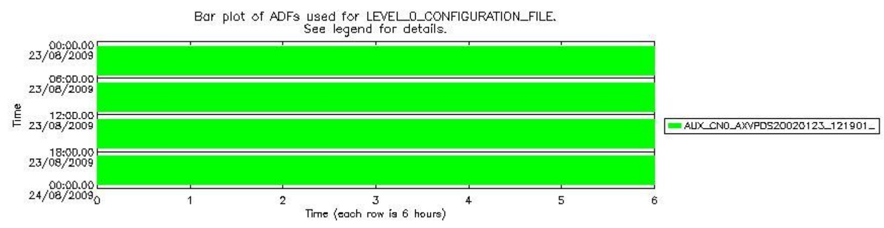
sciamachy_daily_report_level0_KSPT_L0_4303_N_20090823_6.PNG
