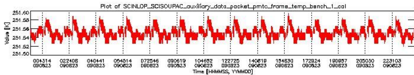
sciamachy_daily_report_level0_KSPT_L0_4303_N_20090823_0.PNG
