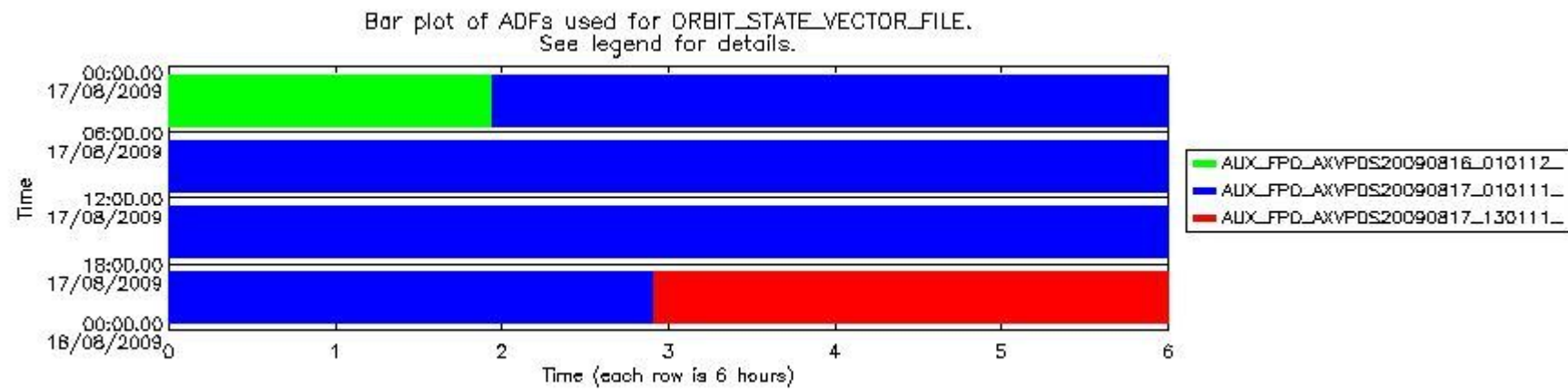
sciamachy_daily_report_level0_KSPT_L0_4303_N_20090817_7.PNG
