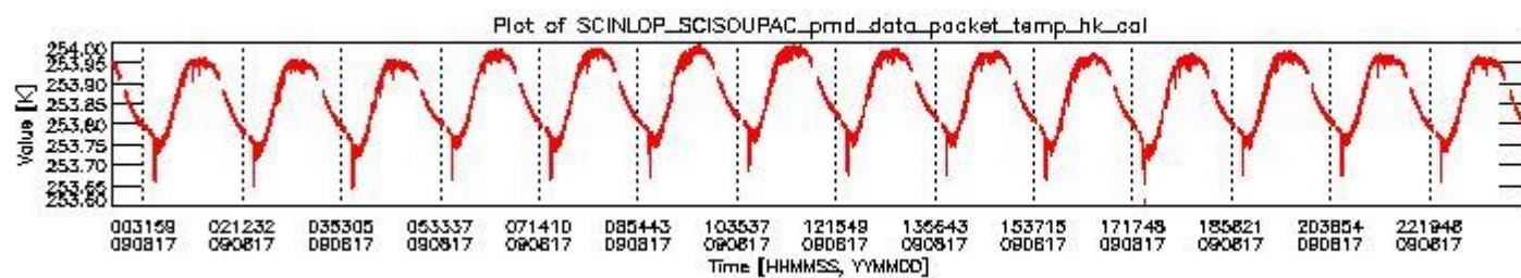
sciamachy_daily_report_level0_KSPT_L0_4303_N_20090817_3.PNG
