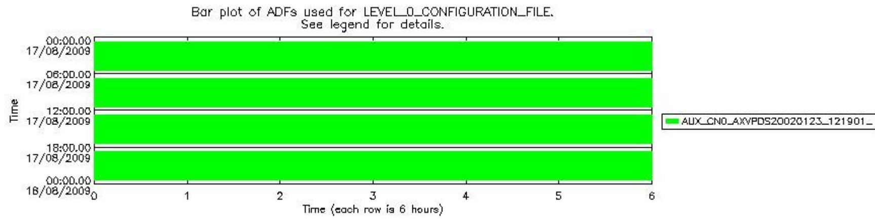
sciamachy_daily_report_level0_KSPT_L0_4303_N_20090817_6.PNG
