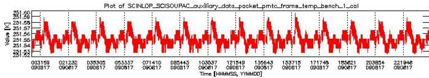
sciamachy_daily_report_level0_KSPT_L0_4303_N_20090817_0.PNG
