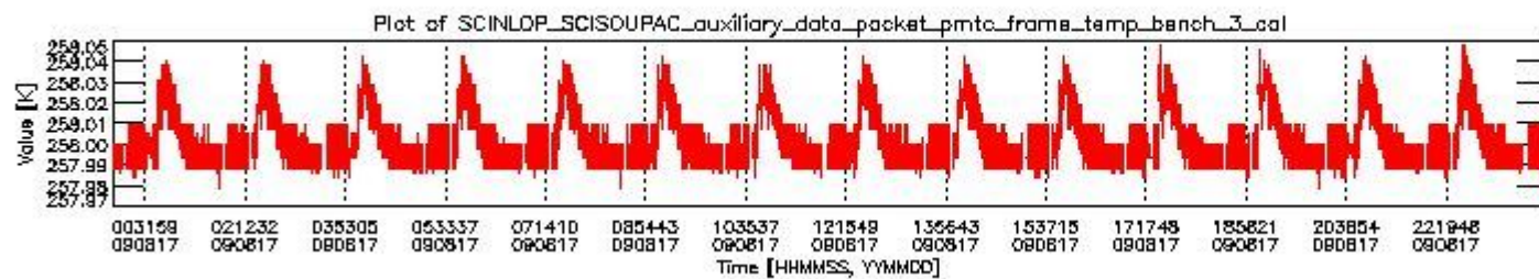
sciamachy_daily_report_level0_KSPT_L0_4303_N_20090817_2.PNG
