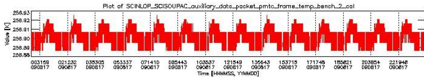
sciamachy_daily_report_level0_KSPT_L0_4303_N_20090817_1.PNG
