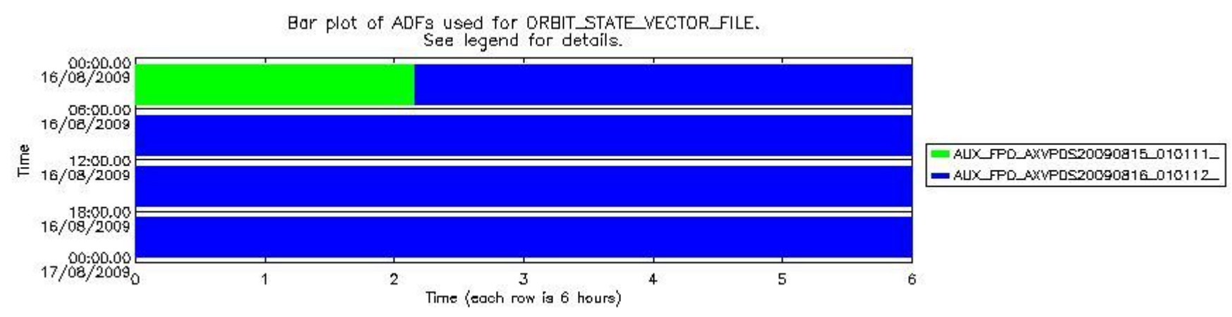
sciamachy_daily_report_level0_KSPT_L0_4303_N_20090816_7.PNG
