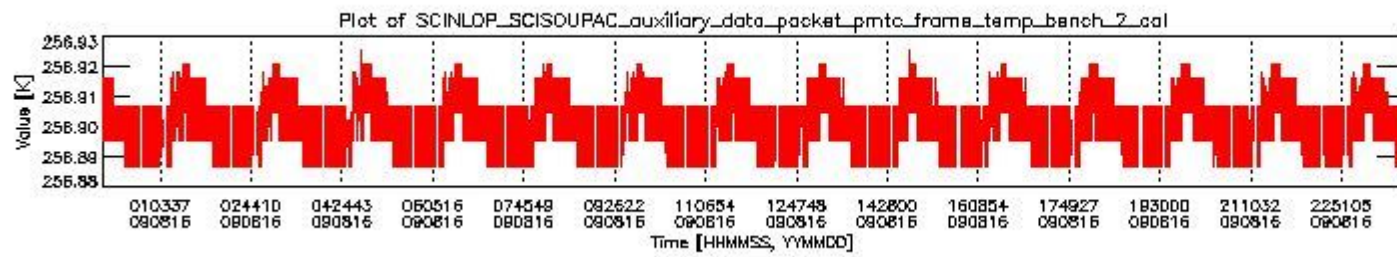
sciamachy_daily_report_level0_KSPT_L0_4303_N_20090816_1.PNG
