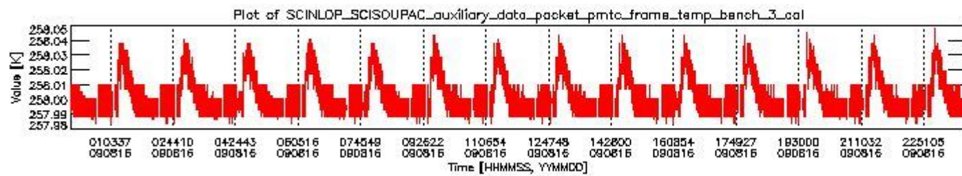
sciamachy_daily_report_level0_KSPT_L0_4303_N_20090816_2.PNG
