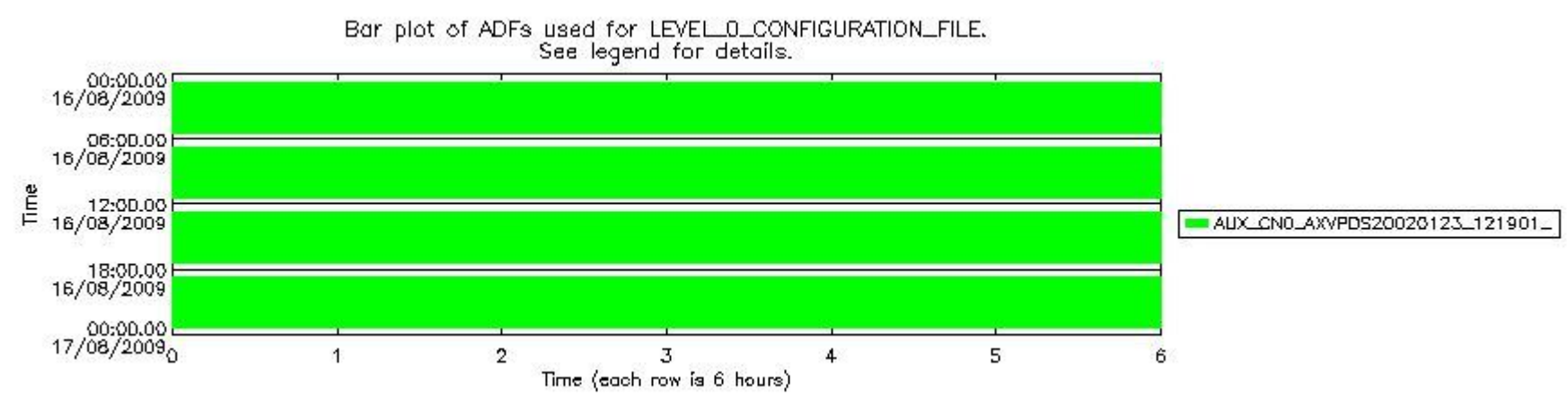
sciamachy_daily_report_level0_KSPT_L0_4303_N_20090816_6.PNG
