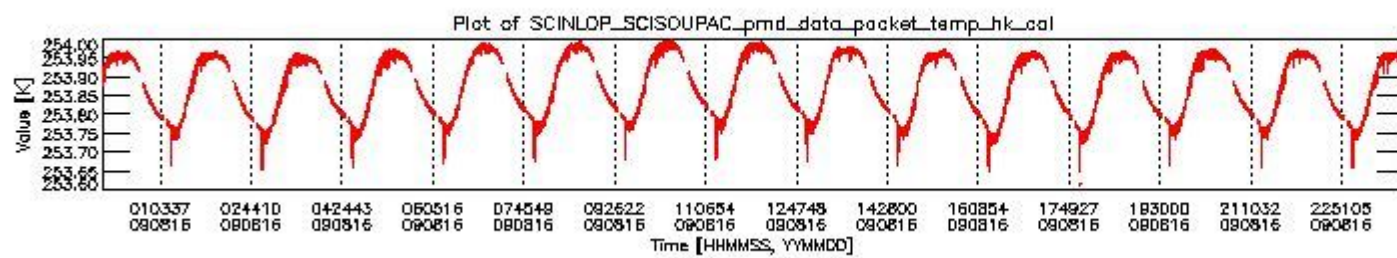
sciamachy_daily_report_level0_KSPT_L0_4303_N_20090816_3.PNG
