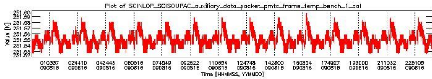
sciamachy_daily_report_level0_KSPT_L0_4303_N_20090816_0.PNG
