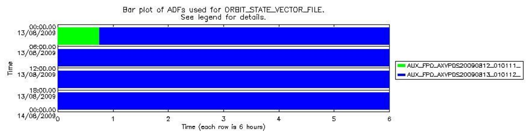
sciamachy_daily_report_level0_KSPT_L0_4303_N_20090813_7.PNG
