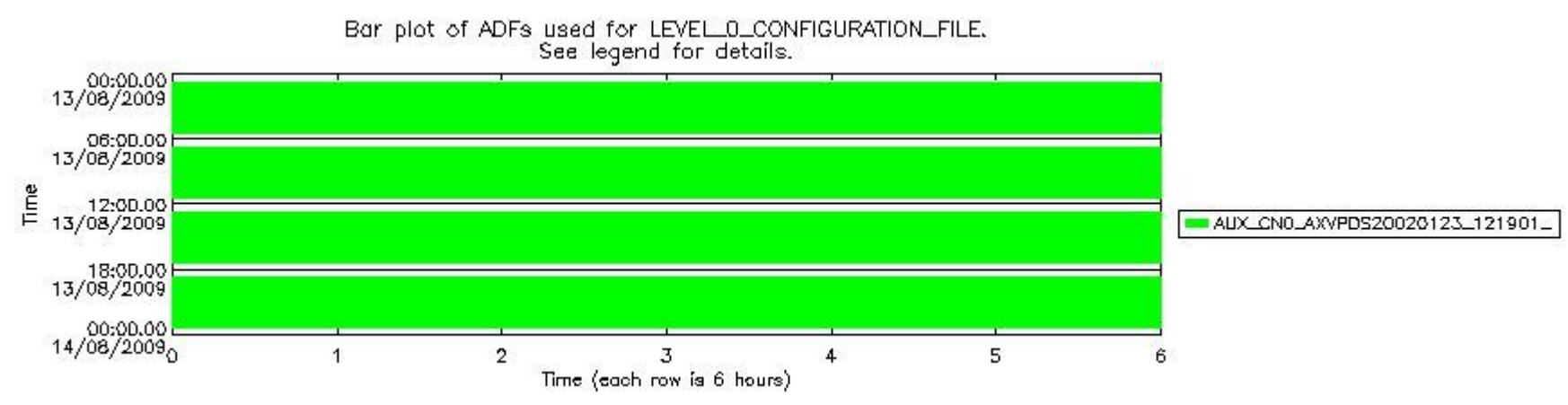
sciamachy_daily_report_level0_KSPT_L0_4303_N_20090813_6.PNG
