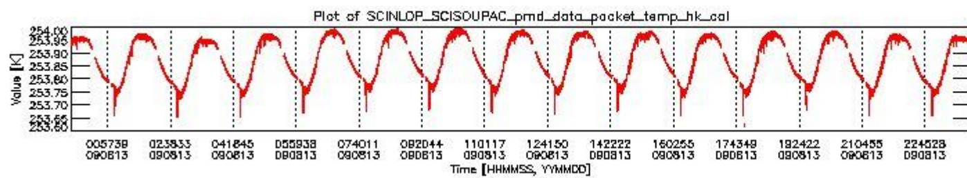
sciamachy_daily_report_level0_KSPT_L0_4303_N_20090813_3.PNG
