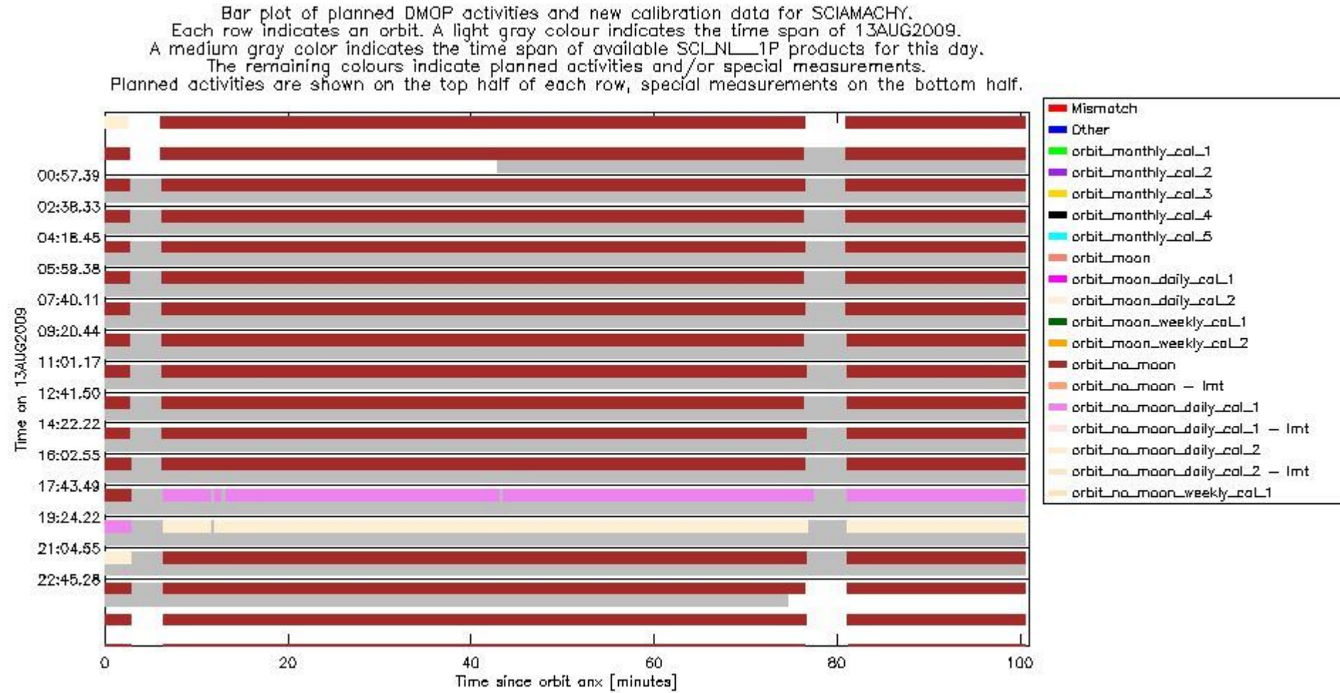
sciamachy_daily_report_level0_KSPT_L0_4303_N_20090813_5.PNG
