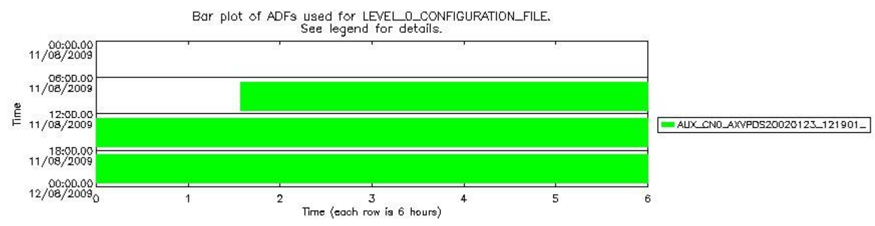
sciamachy_daily_report_level0_KSPT_L0_4303_N_20090811_6.PNG
