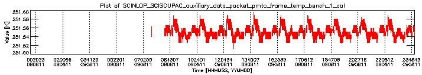
sciamachy_daily_report_level0_KSPT_L0_4303_N_20090811_0.PNG
