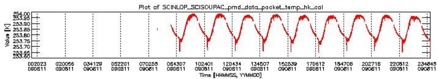
sciamachy_daily_report_level0_KSPT_L0_4303_N_20090811_3.PNG
