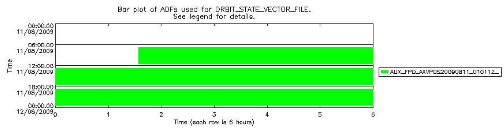
sciamachy_daily_report_level0_KSPT_L0_4303_N_20090811_7.PNG
