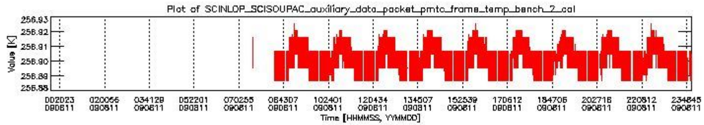
sciamachy_daily_report_level0_KSPT_L0_4303_N_20090811_1.PNG
