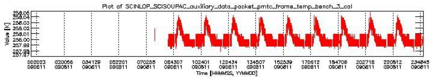
sciamachy_daily_report_level0_KSPT_L0_4303_N_20090811_2.PNG
