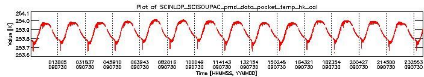
sciamachy_daily_report_level0_KSPT_L0_4303_N_20090730_3.PNG
