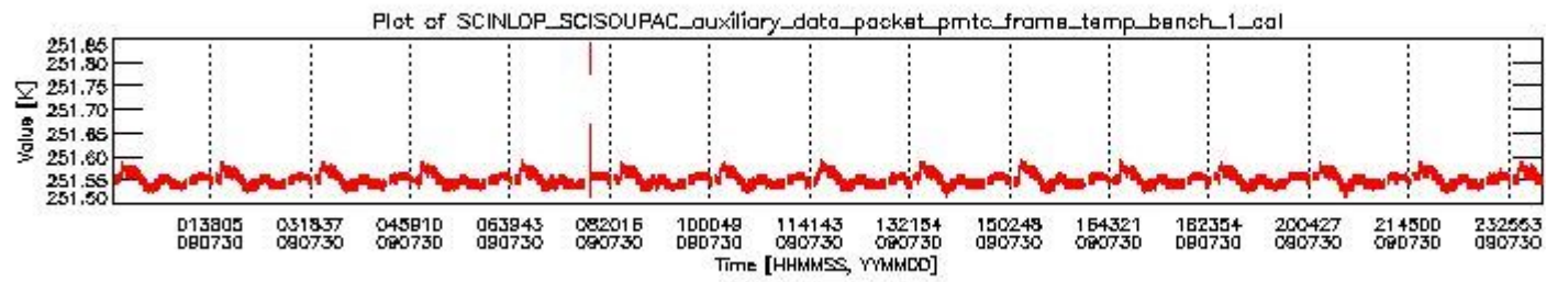
sciamachy_daily_report_level0_KSPT_L0_4303_N_20090730_0.PNG
