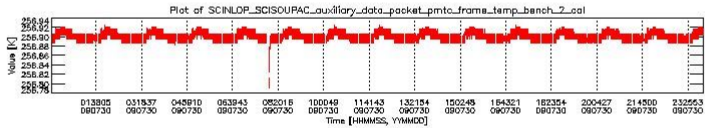
sciamachy_daily_report_level0_KSPT_L0_4303_N_20090730_1.PNG
