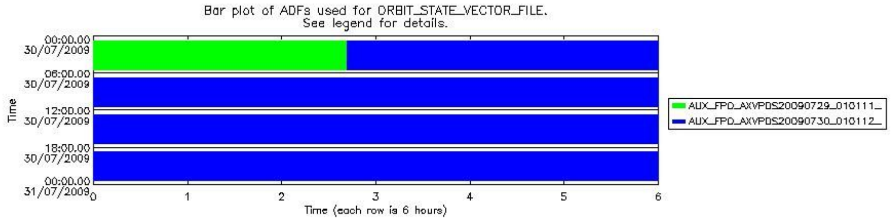
sciamachy_daily_report_level0_KSPT_L0_4303_N_20090730_7.PNG
