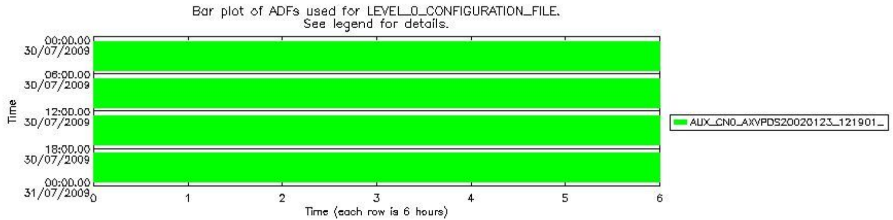
sciamachy_daily_report_level0_KSPT_L0_4303_N_20090730_6.PNG
