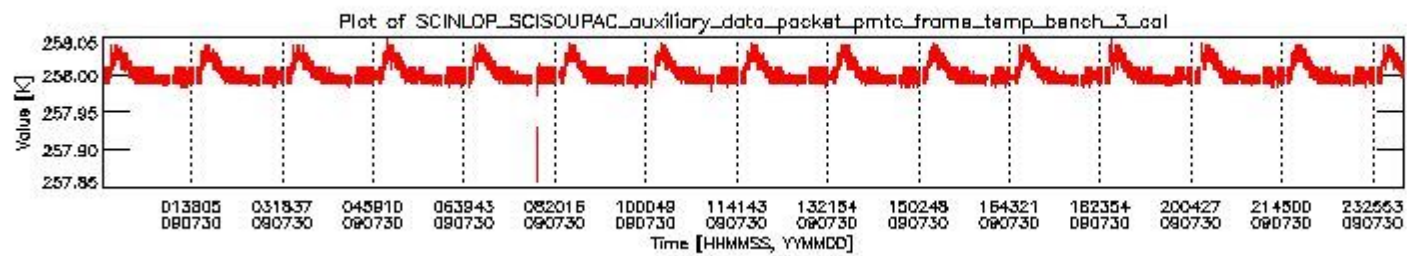
sciamachy_daily_report_level0_KSPT_L0_4303_N_20090730_2.PNG
