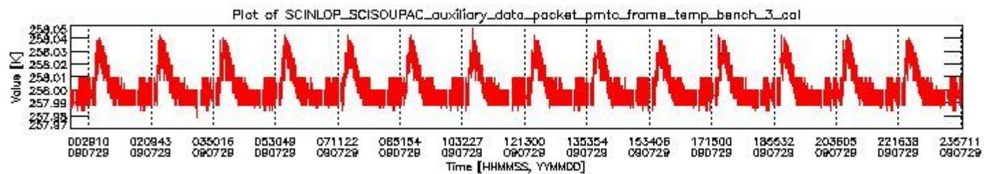
sciamachy_daily_report_level0_KSPT_L0_4303_N_20090729_2.PNG
