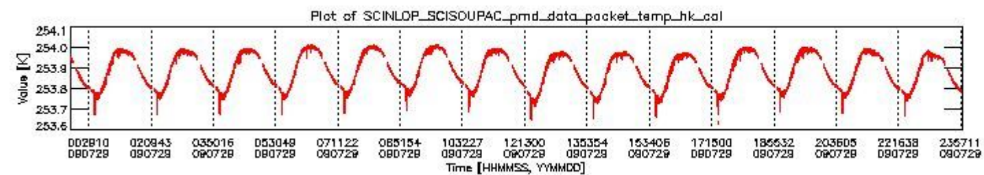
sciamachy_daily_report_level0_KSPT_L0_4303_N_20090729_3.PNG
