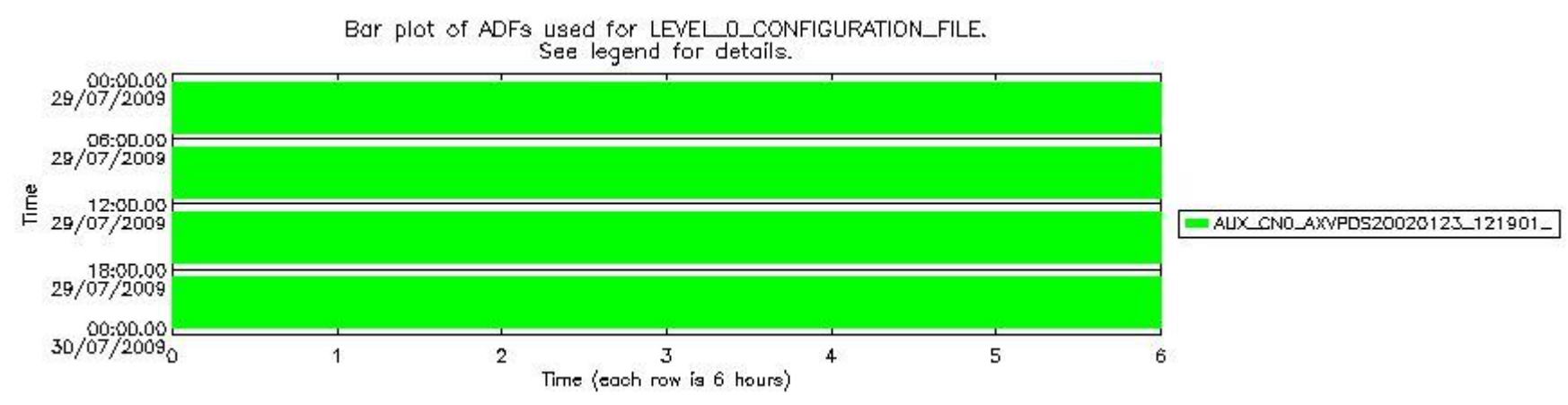
sciamachy_daily_report_level0_KSPT_L0_4303_N_20090729_6.PNG
