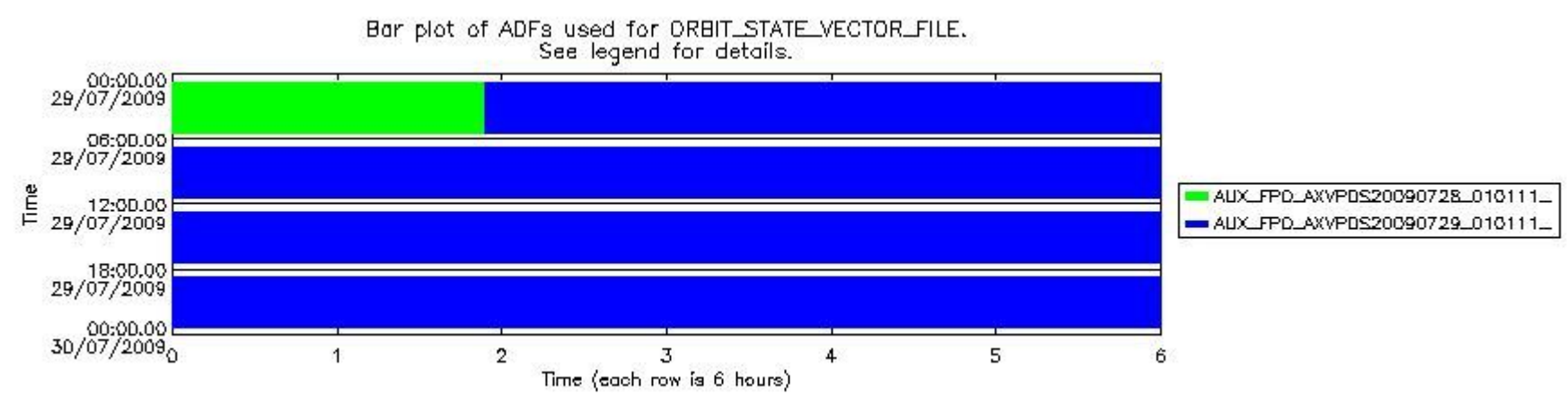
sciamachy_daily_report_level0_KSPT_L0_4303_N_20090729_7.PNG
