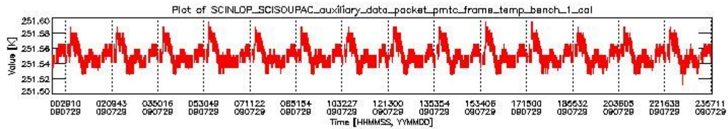
sciamachy_daily_report_level0_KSPT_L0_4303_N_20090729_0.PNG
