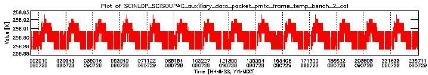
sciamachy_daily_report_level0_KSPT_L0_4303_N_20090729_1.PNG
