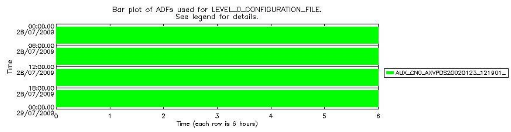
sciamachy_daily_report_level0_KSPT_L0_4303_N_20090728_6.PNG
