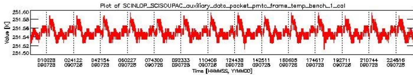
sciamachy_daily_report_level0_KSPT_L0_4303_N_20090728_0.PNG
