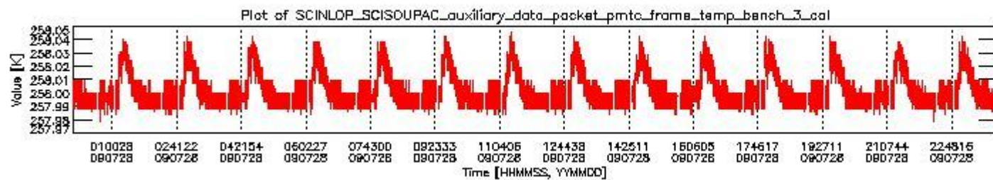
sciamachy_daily_report_level0_KSPT_L0_4303_N_20090728_2.PNG
