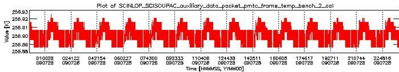
sciamachy_daily_report_level0_KSPT_L0_4303_N_20090728_1.PNG
