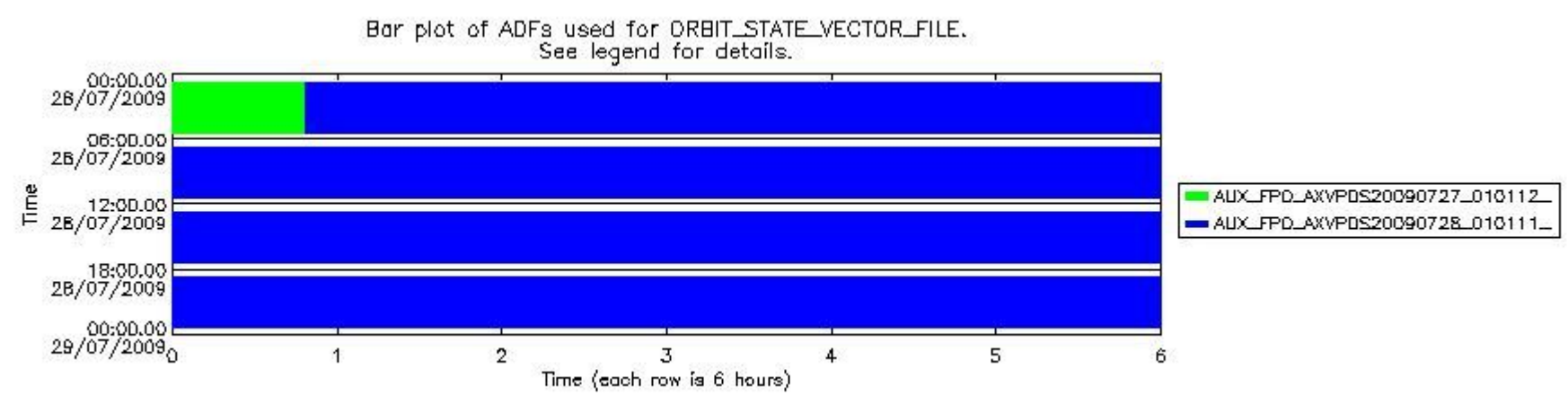
sciamachy_daily_report_level0_KSPT_L0_4303_N_20090728_7.PNG
