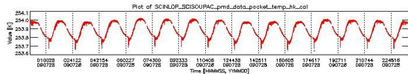
sciamachy_daily_report_level0_KSPT_L0_4303_N_20090728_3.PNG
