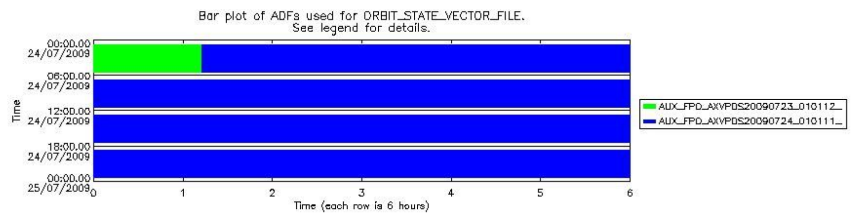
sciamachy_daily_report_level0_KSPT_L0_4303_N_20090724_7.PNG
