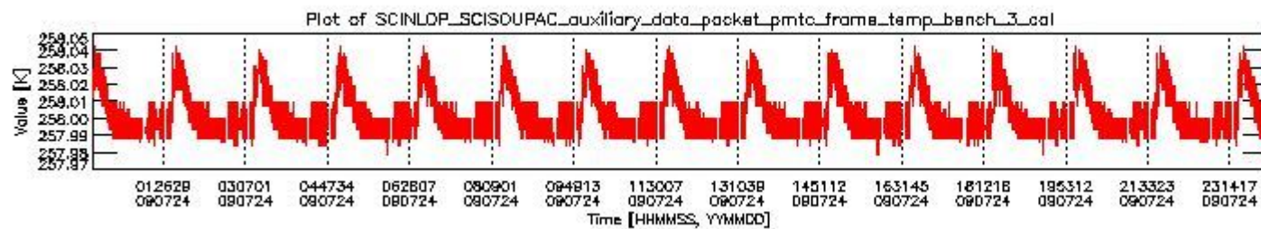
sciamachy_daily_report_level0_KSPT_L0_4303_N_20090724_2.PNG
