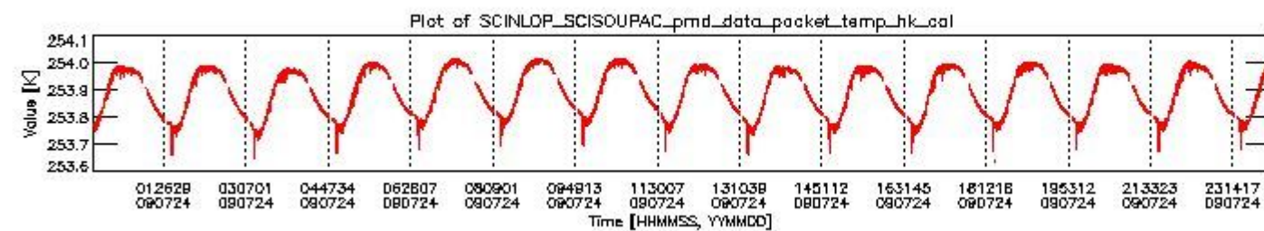
sciamachy_daily_report_level0_KSPT_L0_4303_N_20090724_3.PNG
