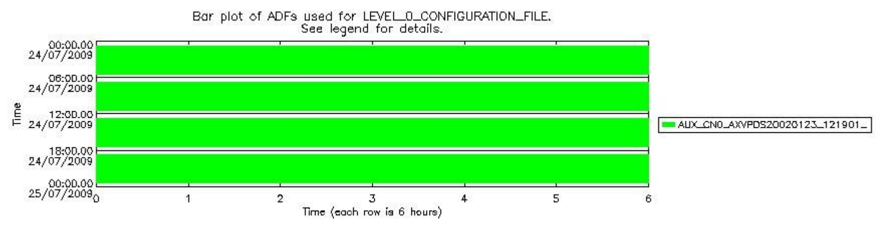
sciamachy_daily_report_level0_KSPT_L0_4303_N_20090724_6.PNG
