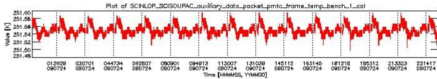
sciamachy_daily_report_level0_KSPT_L0_4303_N_20090724_0.PNG
