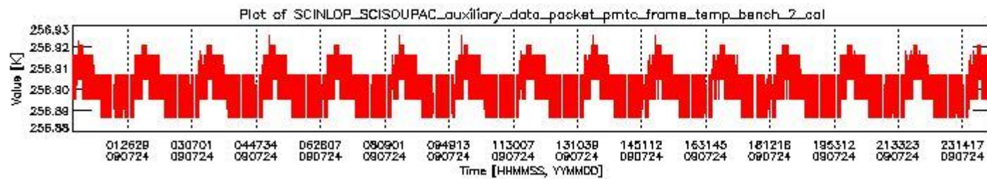
sciamachy_daily_report_level0_KSPT_L0_4303_N_20090724_1.PNG
