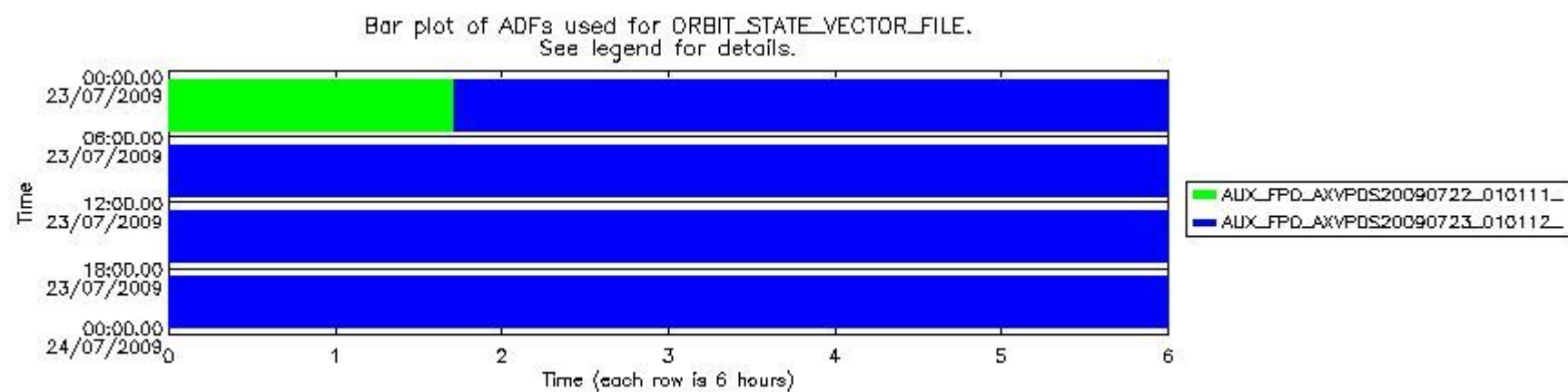
sciamachy_daily_report_level0_KSPT_L0_4303_N_20090723_7.PNG
