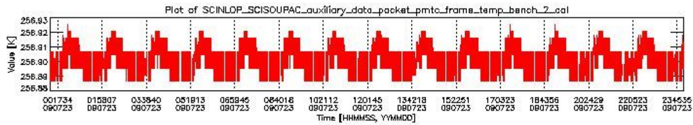
sciamachy_daily_report_level0_KSPT_L0_4303_N_20090723_1.PNG
