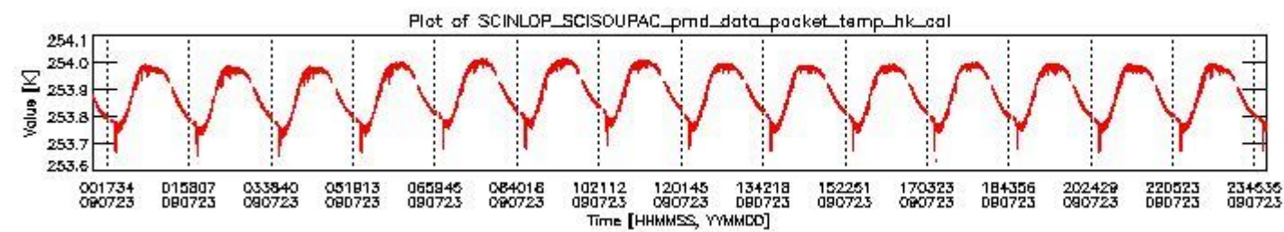
sciamachy_daily_report_level0_KSPT_L0_4303_N_20090723_3.PNG
