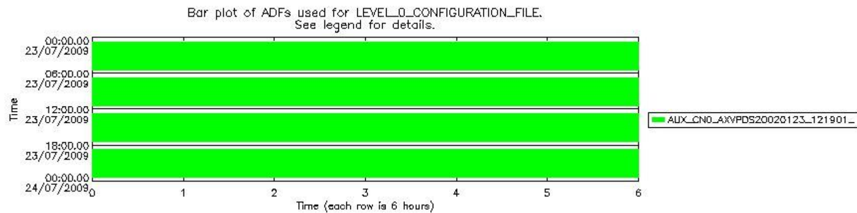
sciamachy_daily_report_level0_KSPT_L0_4303_N_20090723_6.PNG
