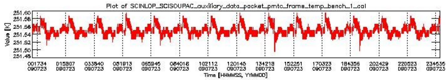
sciamachy_daily_report_level0_KSPT_L0_4303_N_20090723_0.PNG
