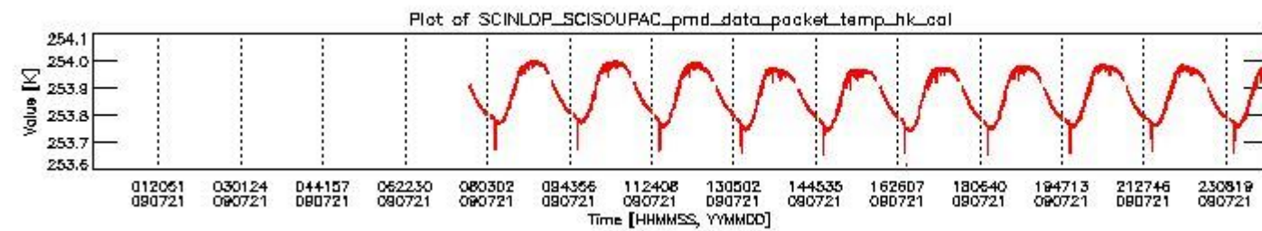
sciamachy_daily_report_level0_KSPT_L0_4303_N_20090721_3.PNG
