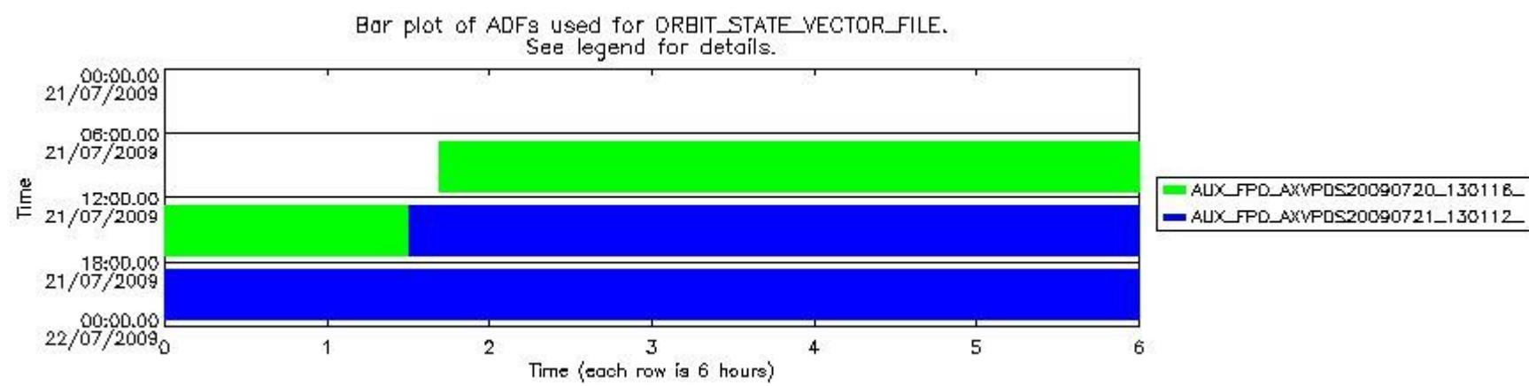
sciamachy_daily_report_level0_KSPT_L0_4303_N_20090721_7.PNG
