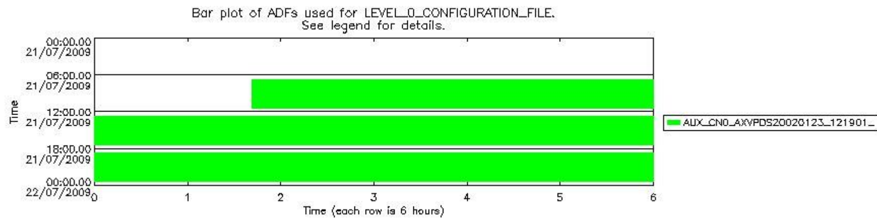
sciamachy_daily_report_level0_KSPT_L0_4303_N_20090721_6.PNG
