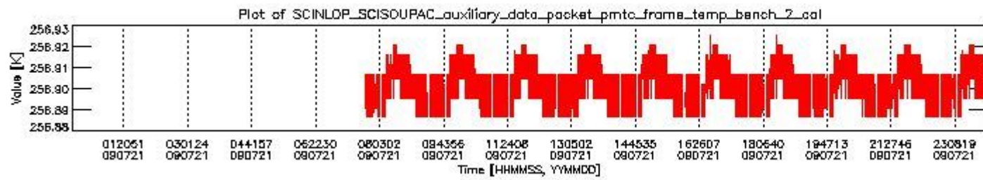
sciamachy_daily_report_level0_KSPT_L0_4303_N_20090721_1.PNG
