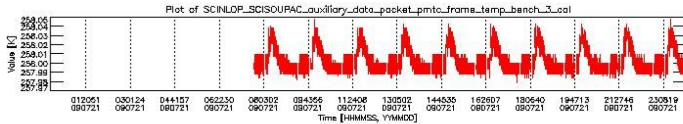
sciamachy_daily_report_level0_KSPT_L0_4303_N_20090721_2.PNG
