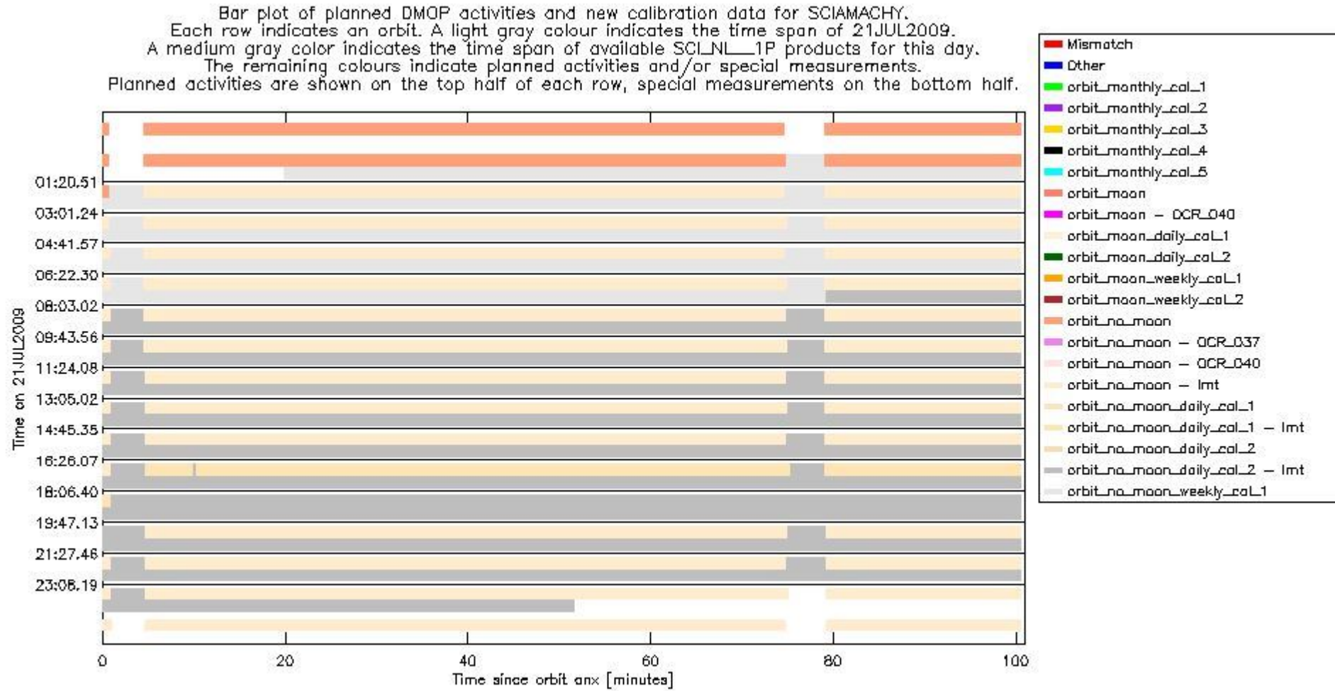
sciamachy_daily_report_level0_KSPT_L0_4303_N_20090721_5.PNG
