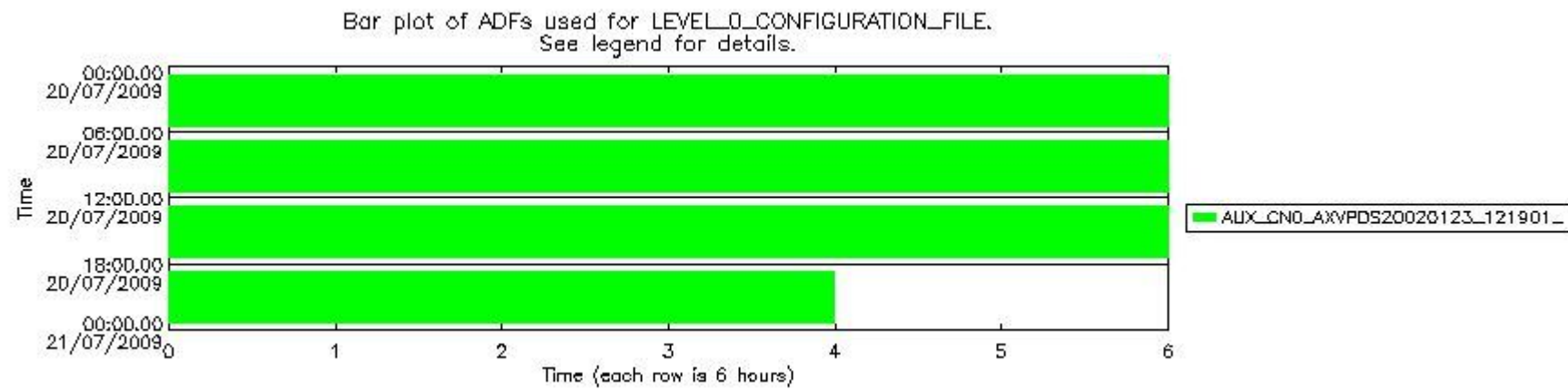
sciamachy_daily_report_level0_KSPT_L0_4303_N_20090720_6.PNG
