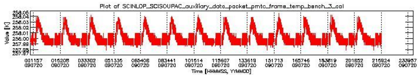
sciamachy_daily_report_level0_KSPT_L0_4303_N_20090720_2.PNG
