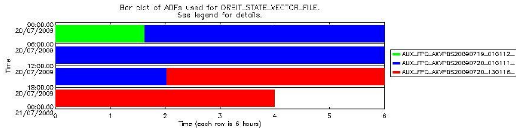
sciamachy_daily_report_level0_KSPT_L0_4303_N_20090720_7.PNG
