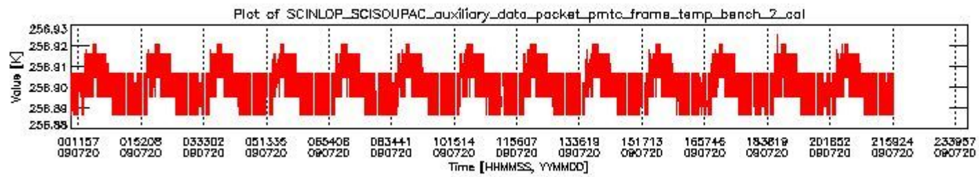
sciamachy_daily_report_level0_KSPT_L0_4303_N_20090720_1.PNG
