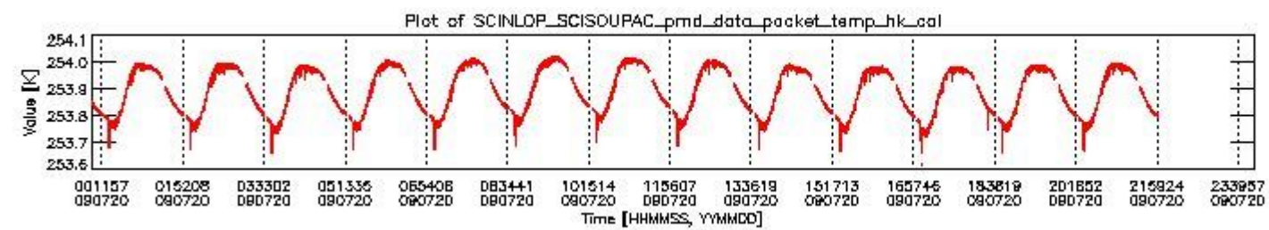
sciamachy_daily_report_level0_KSPT_L0_4303_N_20090720_3.PNG
