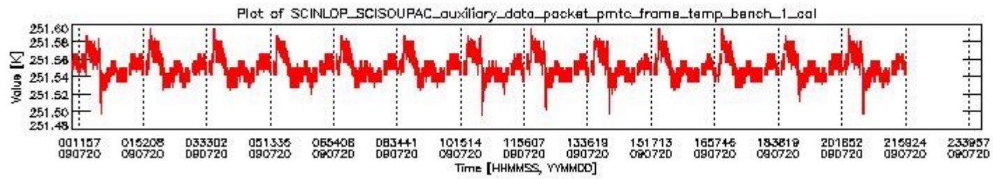
sciamachy_daily_report_level0_KSPT_L0_4303_N_20090720_0.PNG
