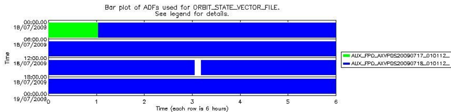
sciamachy_daily_report_level0_KSPT_L0_4303_N_20090718_7.PNG
