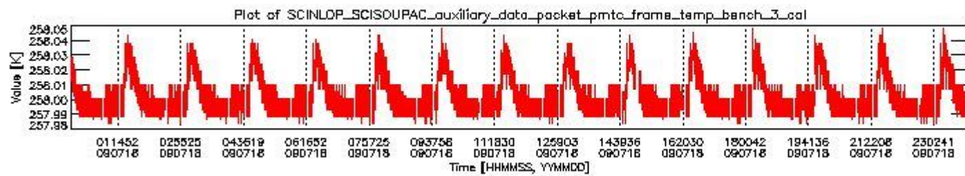
sciamachy_daily_report_level0_KSPT_L0_4303_N_20090718_2.PNG
