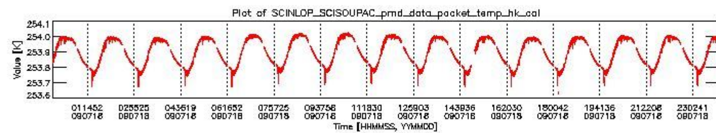
sciamachy_daily_report_level0_KSPT_L0_4303_N_20090718_3.PNG
