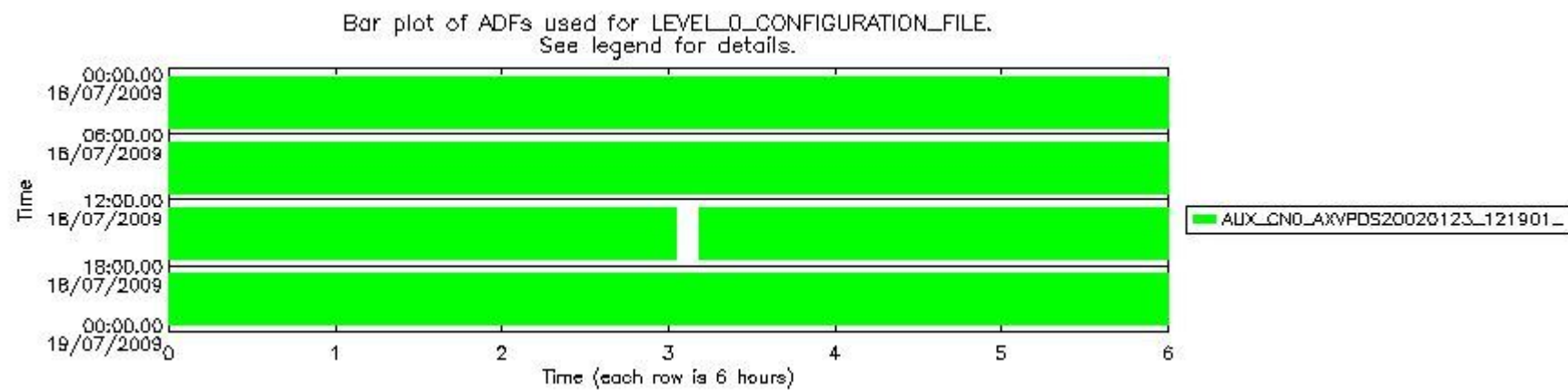
sciamachy_daily_report_level0_KSPT_L0_4303_N_20090718_6.PNG
