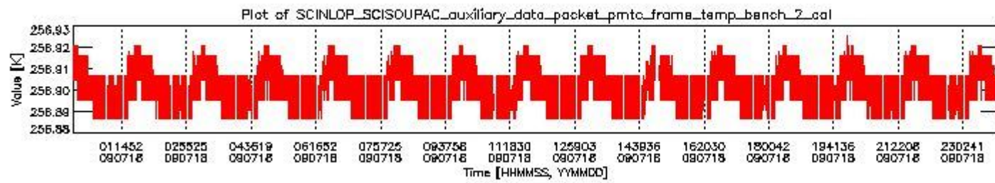
sciamachy_daily_report_level0_KSPT_L0_4303_N_20090718_1.PNG
