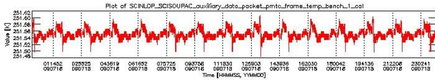
sciamachy_daily_report_level0_KSPT_L0_4303_N_20090718_0.PNG
