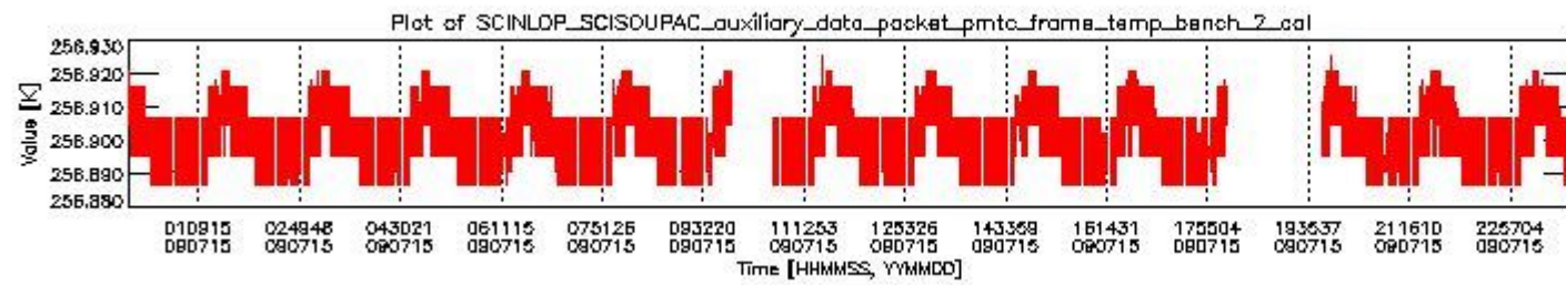
sciamachy_daily_report_level0_KSPT_L0_4303_N_20090715_1.PNG
