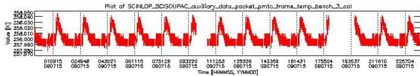
sciamachy_daily_report_level0_KSPT_L0_4303_N_20090715_2.PNG
