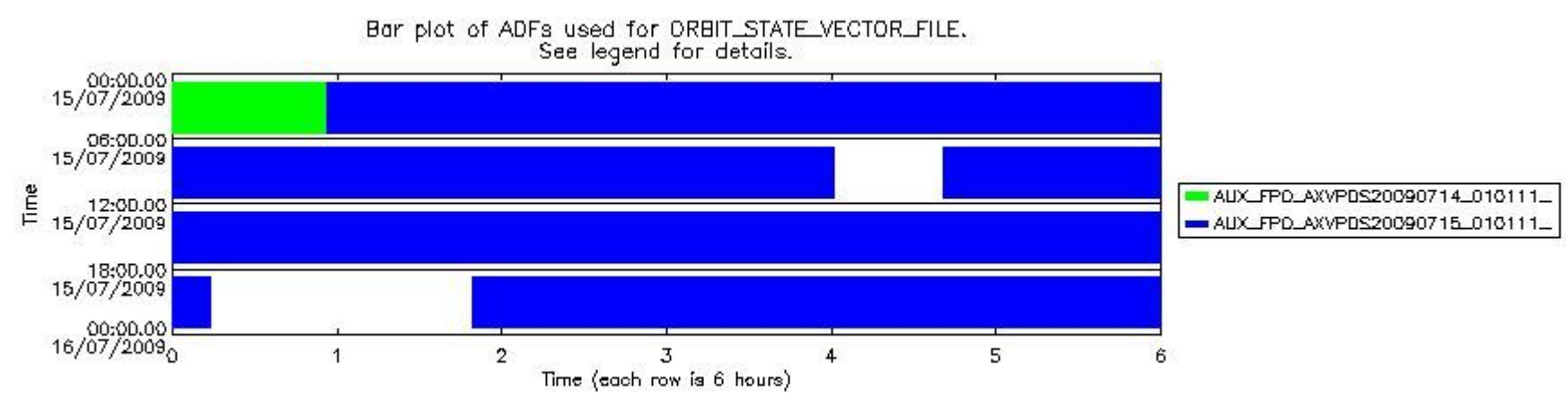
sciamachy_daily_report_level0_KSPT_L0_4303_N_20090715_7.PNG
