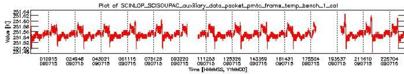
sciamachy_daily_report_level0_KSPT_L0_4303_N_20090715_0.PNG
