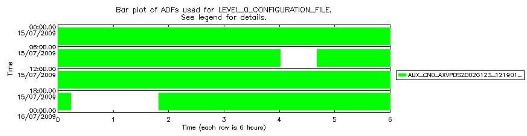
sciamachy_daily_report_level0_KSPT_L0_4303_N_20090715_6.PNG
