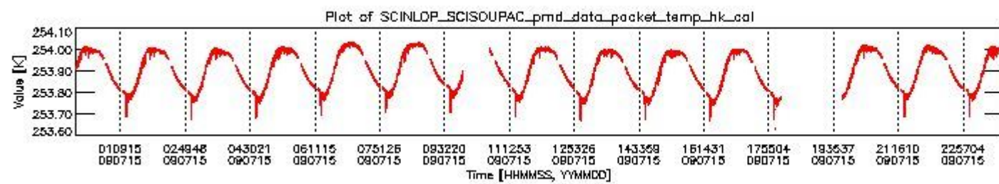
sciamachy_daily_report_level0_KSPT_L0_4303_N_20090715_3.PNG
