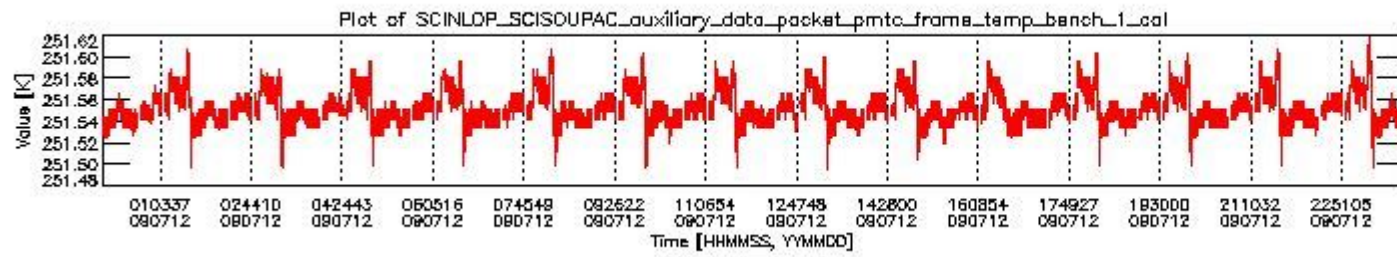
sciamachy_daily_report_level0_KSPT_L0_4303_N_20090712_0.PNG
