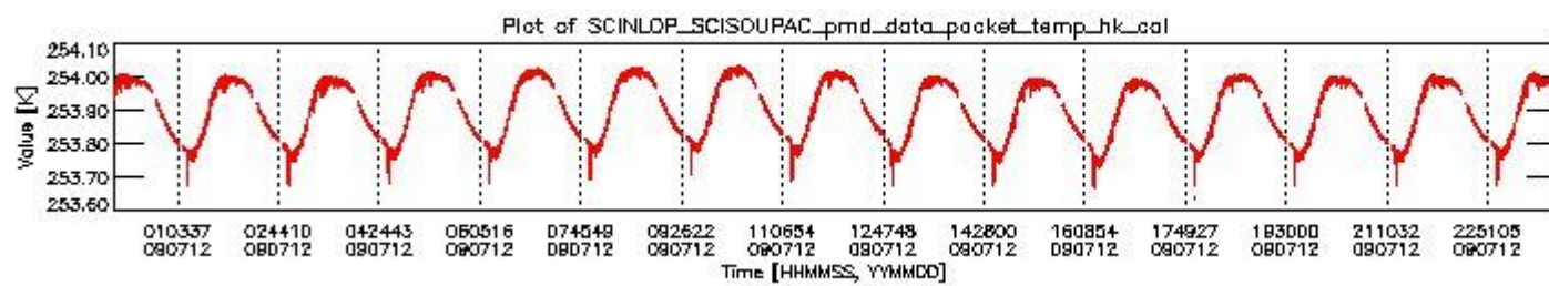
sciamachy_daily_report_level0_KSPT_L0_4303_N_20090712_3.PNG
