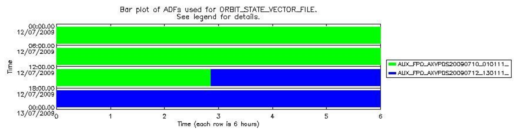
sciamachy_daily_report_level0_KSPT_L0_4303_N_20090712_7.PNG
