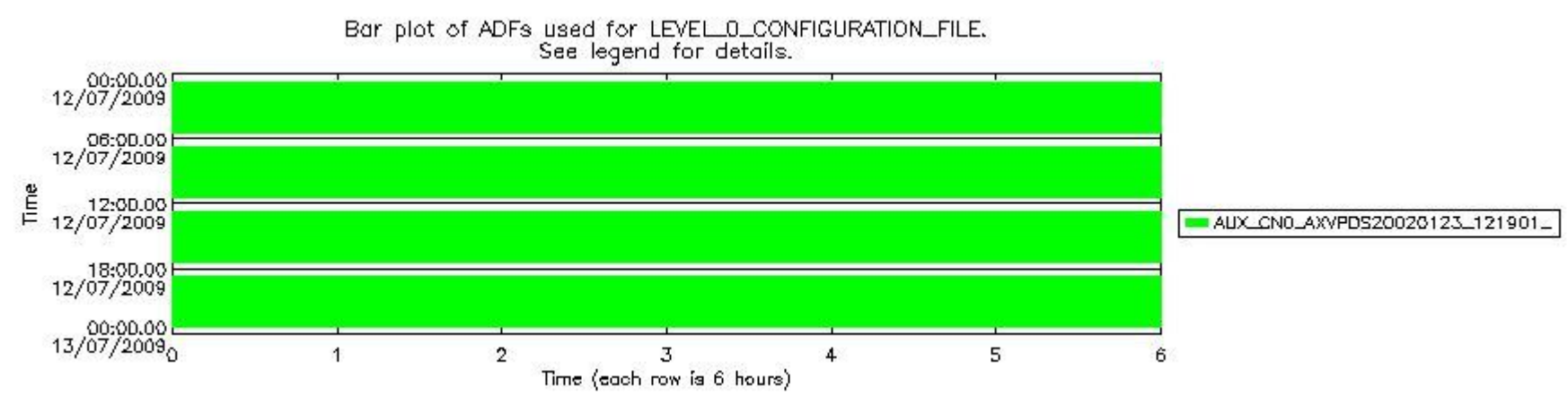
sciamachy_daily_report_level0_KSPT_L0_4303_N_20090712_6.PNG
