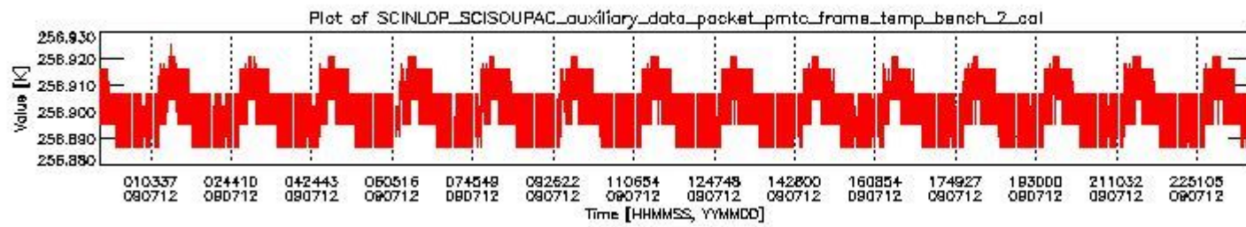
sciamachy_daily_report_level0_KSPT_L0_4303_N_20090712_1.PNG
