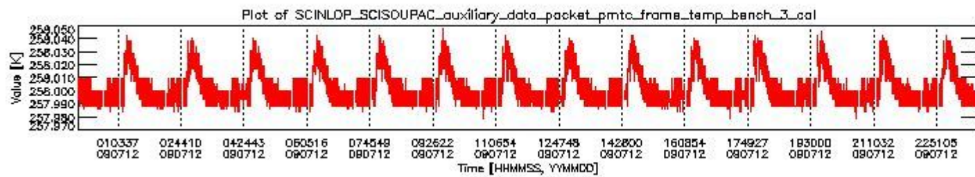
sciamachy_daily_report_level0_KSPT_L0_4303_N_20090712_2.PNG
