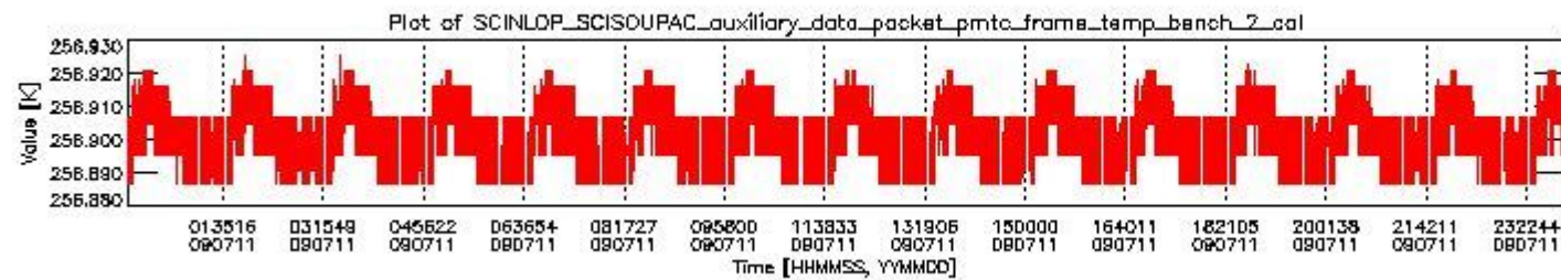
sciamachy_daily_report_level0_KSPT_L0_4303_N_20090711_1.PNG
