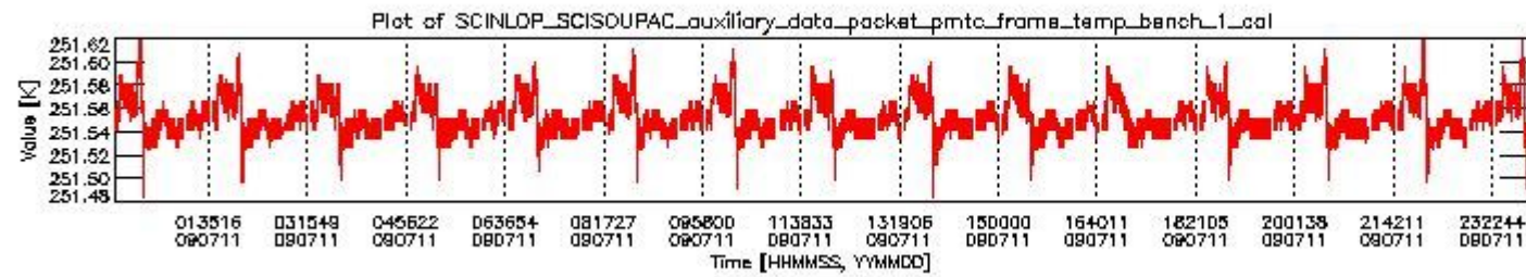
sciamachy_daily_report_level0_KSPT_L0_4303_N_20090711_0.PNG
