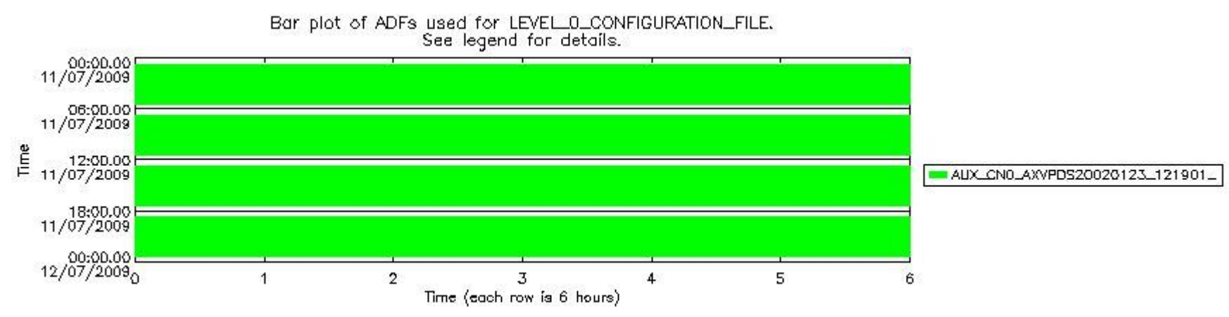
sciamachy_daily_report_level0_KSPT_L0_4303_N_20090711_6.PNG
