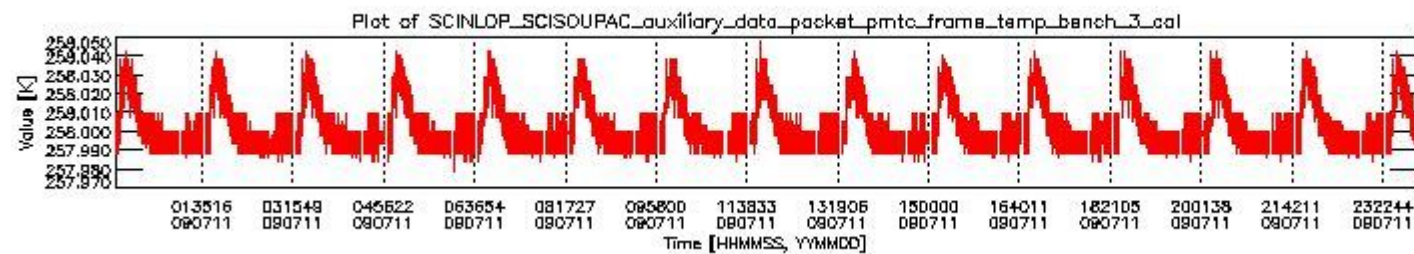
sciamachy_daily_report_level0_KSPT_L0_4303_N_20090711_2.PNG
