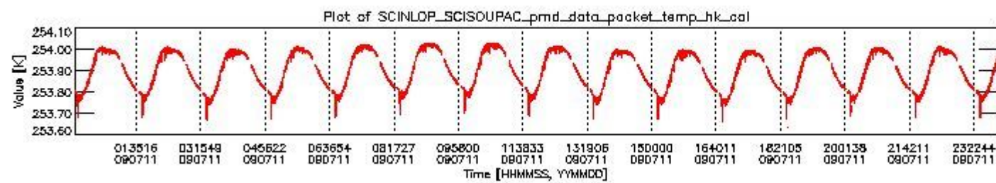
sciamachy_daily_report_level0_KSPT_L0_4303_N_20090711_3.PNG
