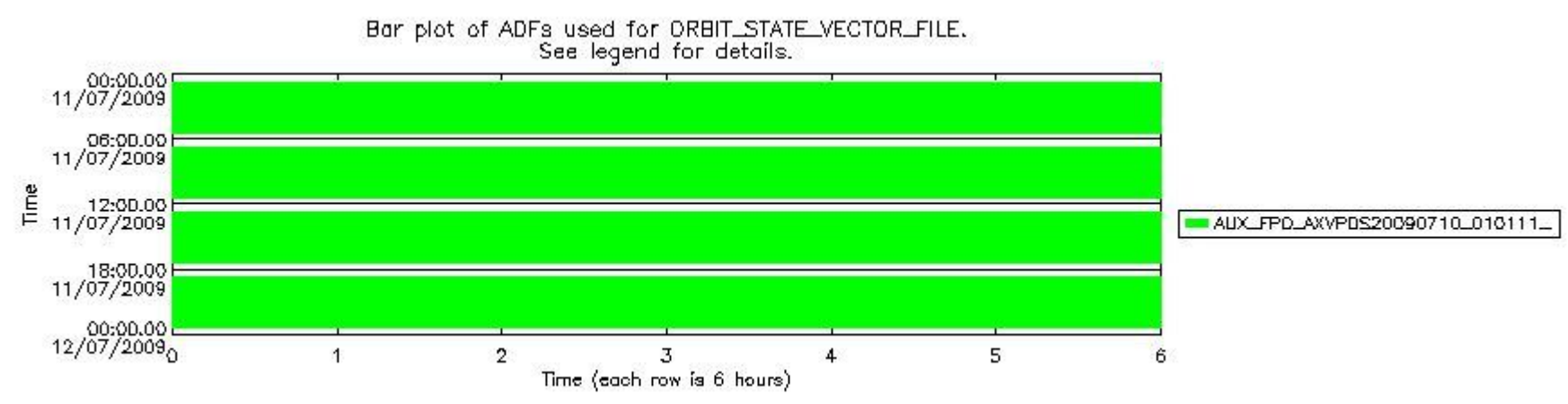
sciamachy_daily_report_level0_KSPT_L0_4303_N_20090711_7.PNG
