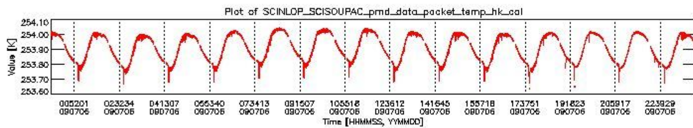
sciamachy_daily_report_level0_KSPT_L0_4303_N_20090706_3.PNG
