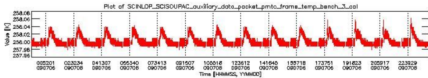
sciamachy_daily_report_level0_KSPT_L0_4303_N_20090706_2.PNG
