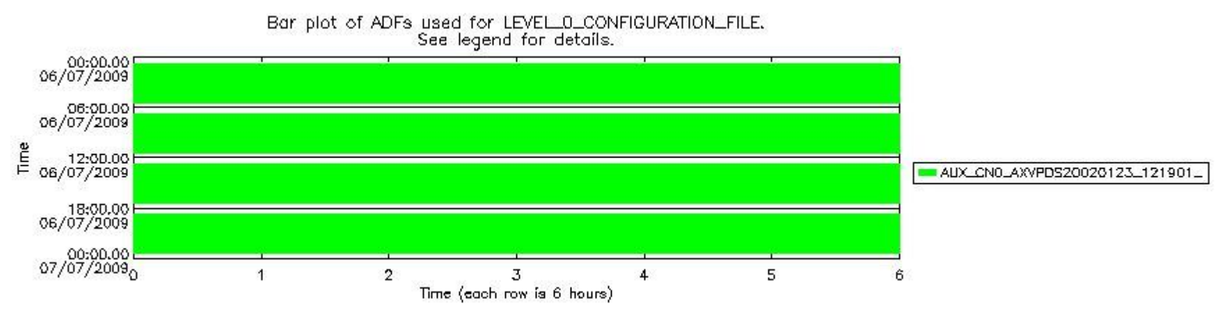
sciamachy_daily_report_level0_KSPT_L0_4303_N_20090706_6.PNG
