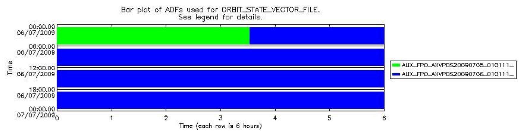
sciamachy_daily_report_level0_KSPT_L0_4303_N_20090706_7.PNG
