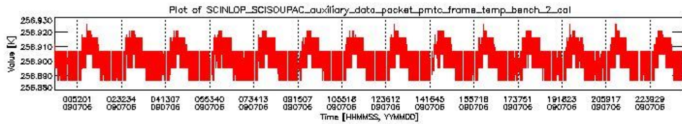
sciamachy_daily_report_level0_KSPT_L0_4303_N_20090706_1.PNG
