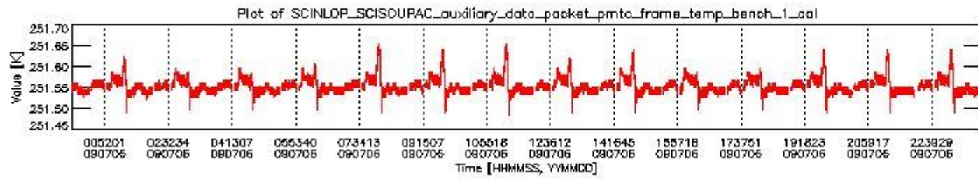
sciamachy_daily_report_level0_KSPT_L0_4303_N_20090706_0.PNG
