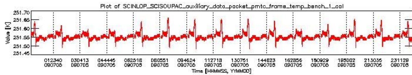
sciamachy_daily_report_level0_KSPT_L0_4303_N_20090705_0.PNG
