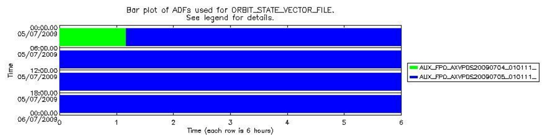
sciamachy_daily_report_level0_KSPT_L0_4303_N_20090705_7.PNG
