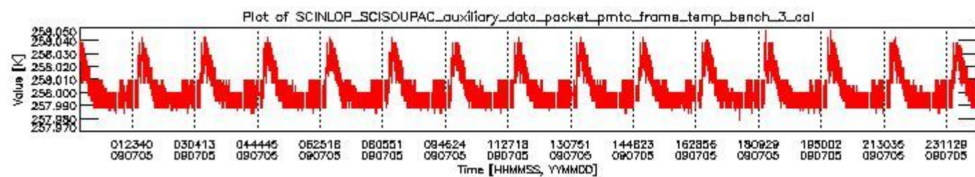
sciamachy_daily_report_level0_KSPT_L0_4303_N_20090705_2.PNG
