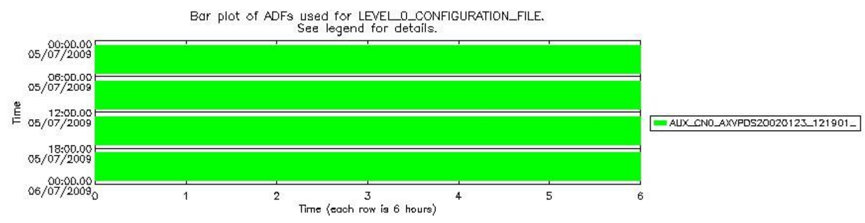
sciamachy_daily_report_level0_KSPT_L0_4303_N_20090705_6.PNG
