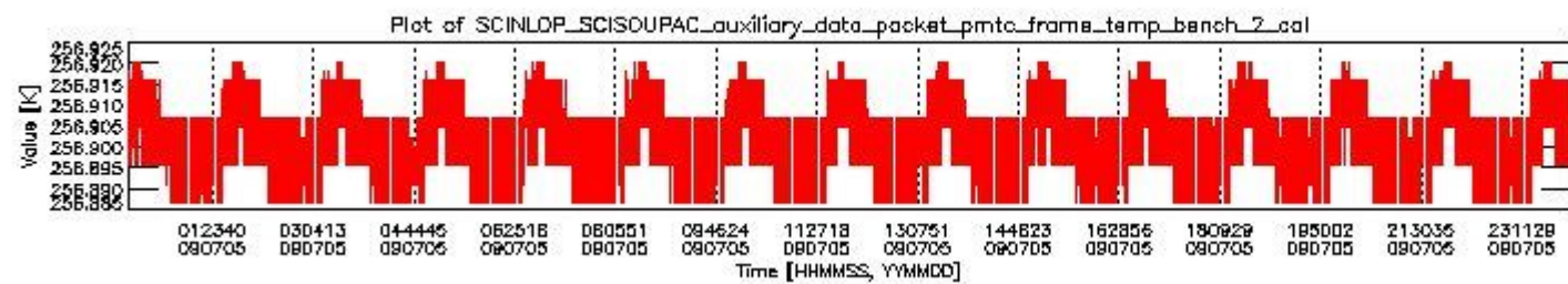
sciamachy_daily_report_level0_KSPT_L0_4303_N_20090705_1.PNG
