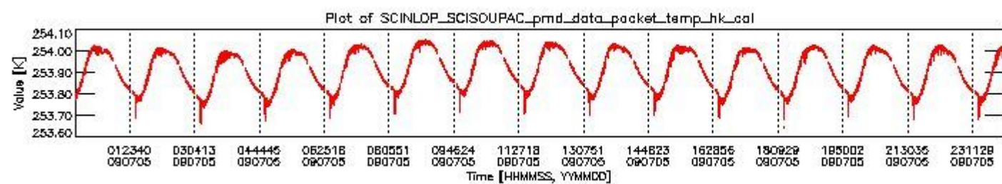
sciamachy_daily_report_level0_KSPT_L0_4303_N_20090705_3.PNG
