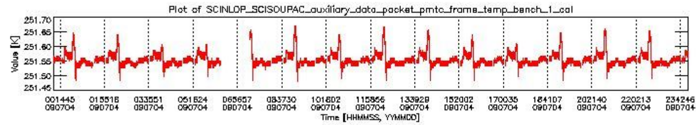
sciamachy_daily_report_level0_KSPT_L0_4303_N_20090704_0.PNG
