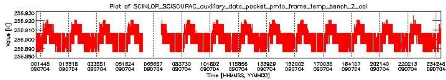
sciamachy_daily_report_level0_KSPT_L0_4303_N_20090704_1.PNG
