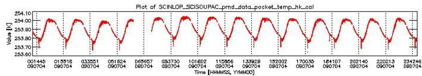
sciamachy_daily_report_level0_KSPT_L0_4303_N_20090704_3.PNG
