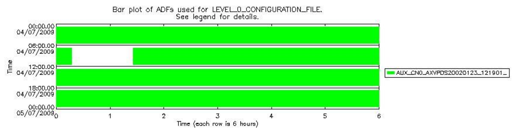
sciamachy_daily_report_level0_KSPT_L0_4303_N_20090704_6.PNG
