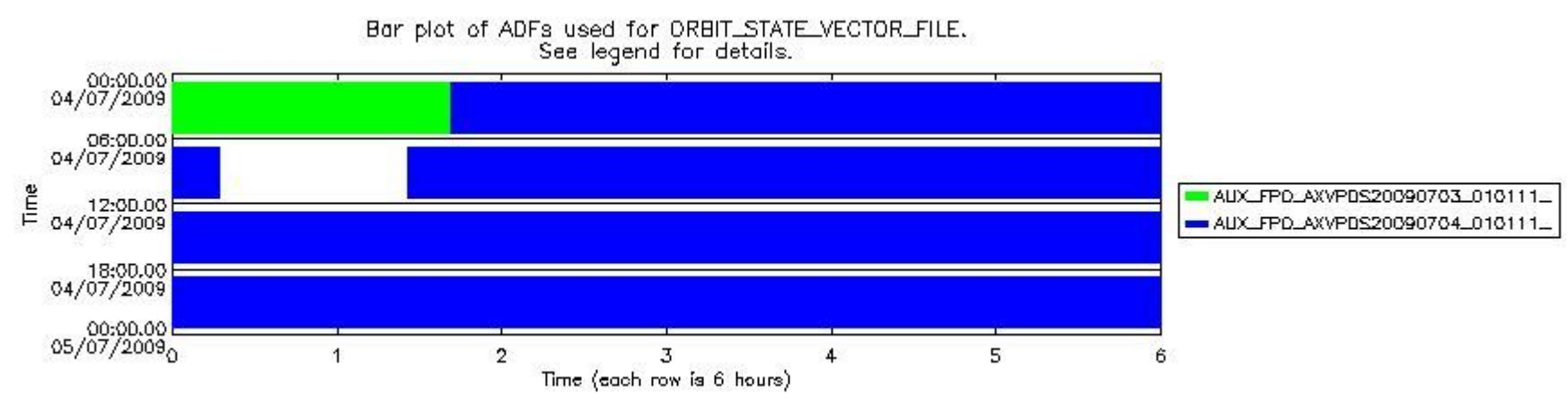
sciamachy_daily_report_level0_KSPT_L0_4303_N_20090704_7.PNG
