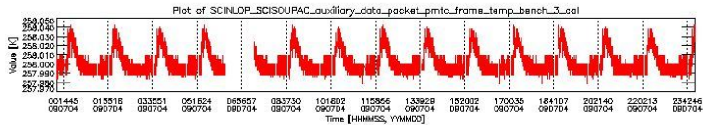
sciamachy_daily_report_level0_KSPT_L0_4303_N_20090704_2.PNG
