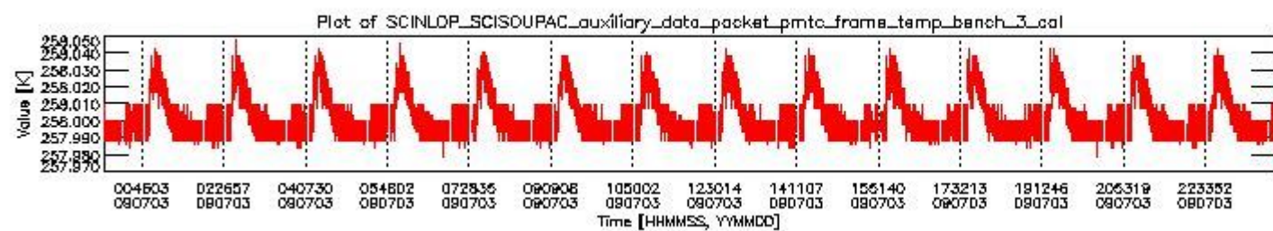
sciamachy_daily_report_level0_KSPT_L0_4303_N_20090703_2.PNG
