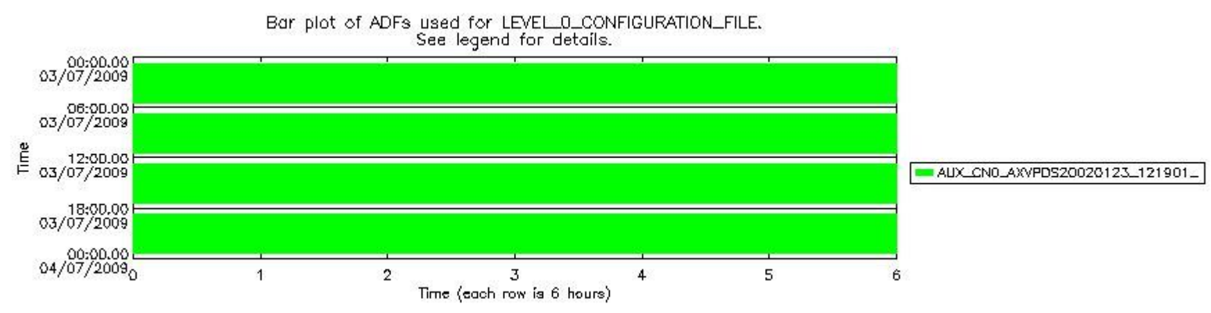
sciamachy_daily_report_level0_KSPT_L0_4303_N_20090703_6.PNG
