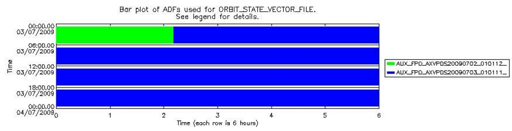
sciamachy_daily_report_level0_KSPT_L0_4303_N_20090703_7.PNG
