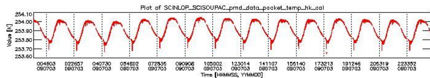
sciamachy_daily_report_level0_KSPT_L0_4303_N_20090703_3.PNG
