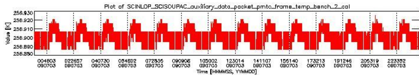
sciamachy_daily_report_level0_KSPT_L0_4303_N_20090703_1.PNG
