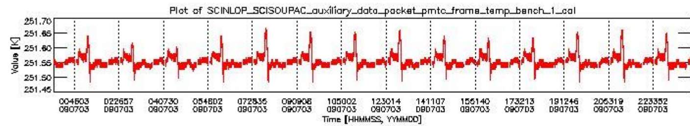
sciamachy_daily_report_level0_KSPT_L0_4303_N_20090703_0.PNG
