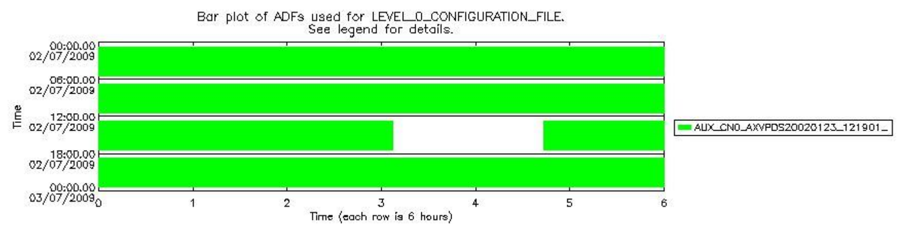
sciamachy_daily_report_level0_KSPT_L0_4303_N_20090702_6.PNG
