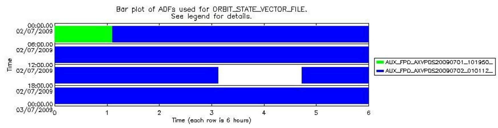
sciamachy_daily_report_level0_KSPT_L0_4303_N_20090702_7.PNG
