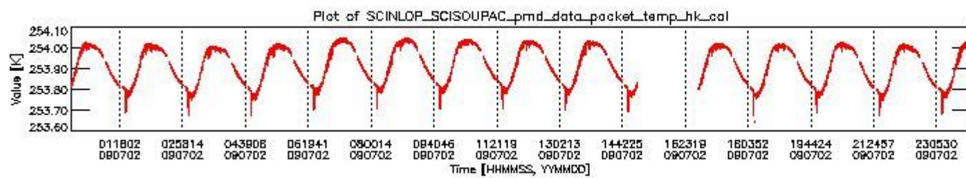
sciamachy_daily_report_level0_KSPT_L0_4303_N_20090702_3.PNG
