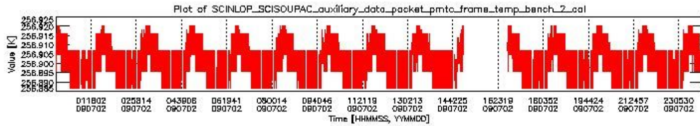
sciamachy_daily_report_level0_KSPT_L0_4303_N_20090702_1.PNG
