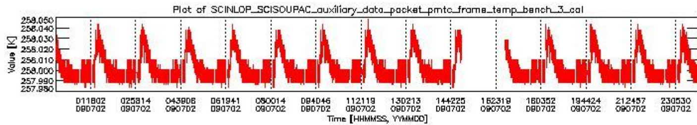
sciamachy_daily_report_level0_KSPT_L0_4303_N_20090702_2.PNG
