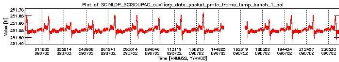
sciamachy_daily_report_level0_KSPT_L0_4303_N_20090702_0.PNG
