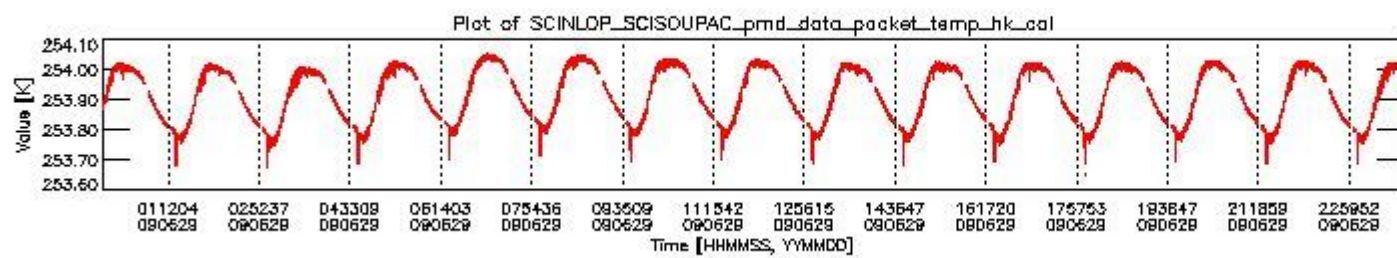
sciamachy_daily_report_level0_KSPT_L0_4303_N_20090629_3.PNG
