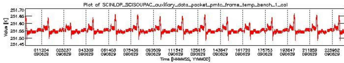
sciamachy_daily_report_level0_KSPT_L0_4303_N_20090629_0.PNG
