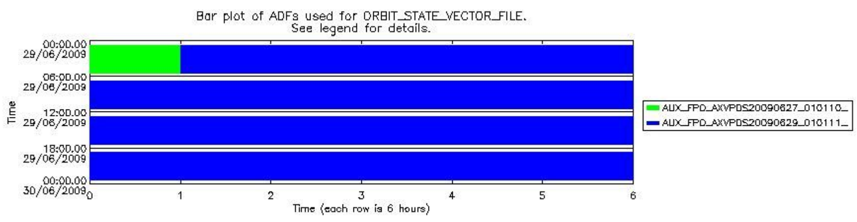
sciamachy_daily_report_level0_KSPT_L0_4303_N_20090629_7.PNG
