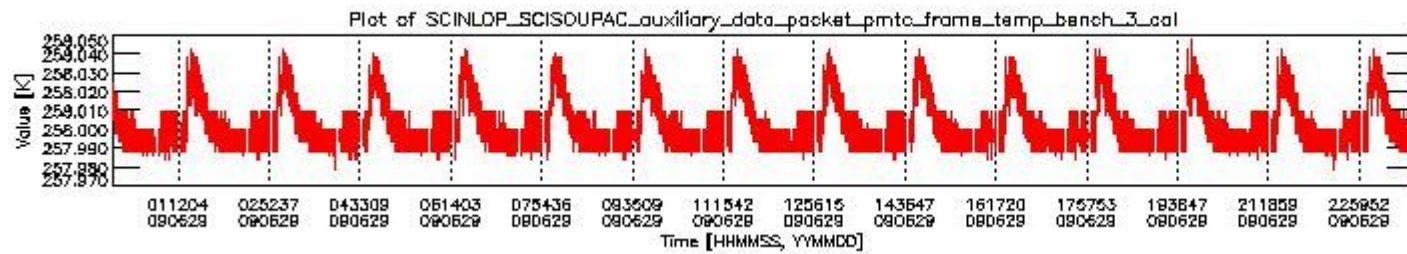
sciamachy_daily_report_level0_KSPT_L0_4303_N_20090629_2.PNG
