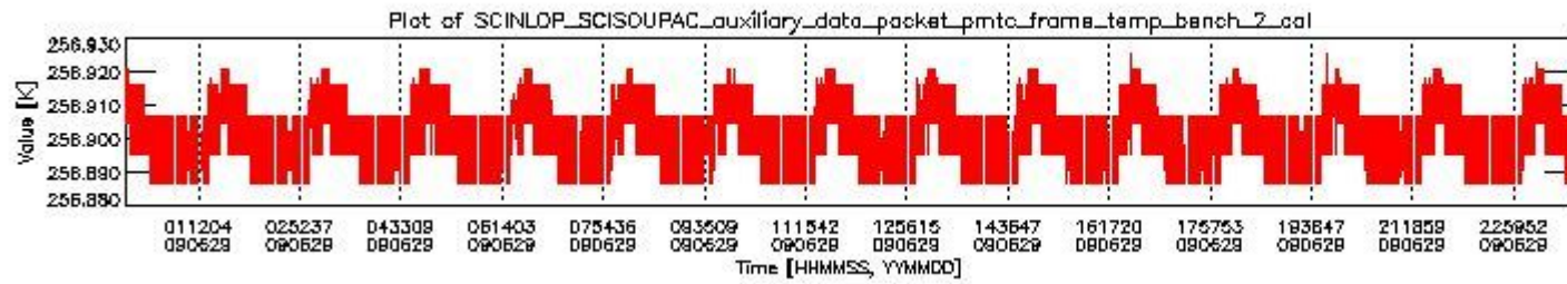
sciamachy_daily_report_level0_KSPT_L0_4303_N_20090629_1.PNG
