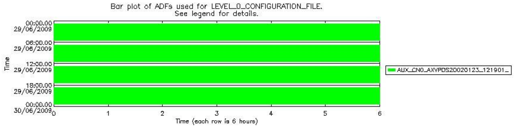
sciamachy_daily_report_level0_KSPT_L0_4303_N_20090629_6.PNG
