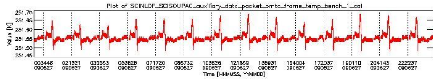
sciamachy_daily_report_level0_KSPT_L0_4303_N_20090627_0.PNG
