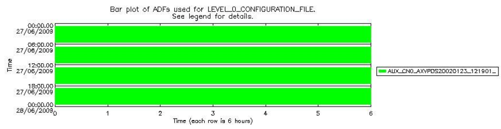
sciamachy_daily_report_level0_KSPT_L0_4303_N_20090627_6.PNG
