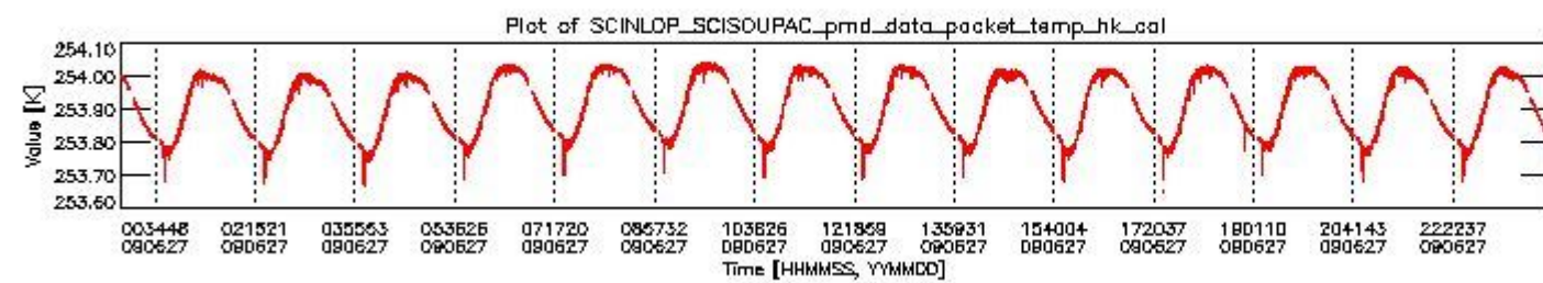
sciamachy_daily_report_level0_KSPT_L0_4303_N_20090627_3.PNG
