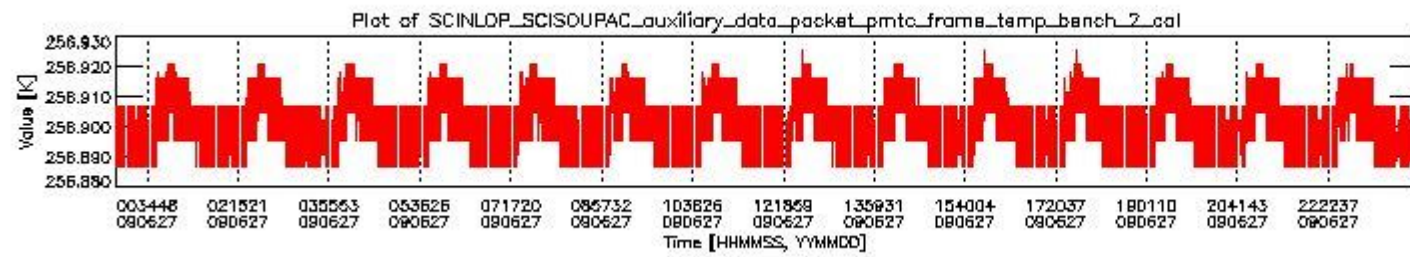
sciamachy_daily_report_level0_KSPT_L0_4303_N_20090627_1.PNG
