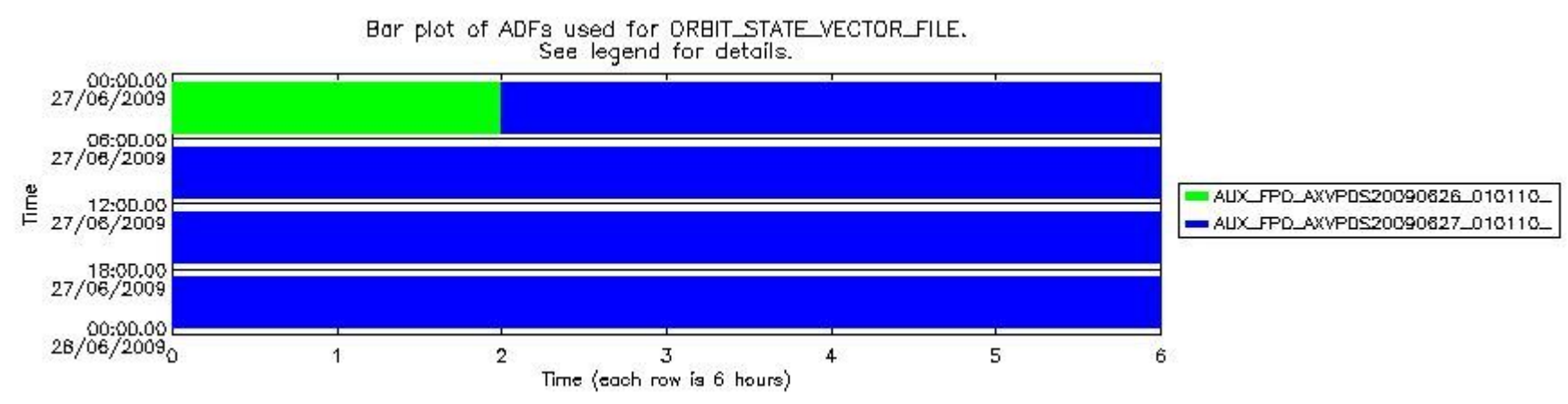
sciamachy_daily_report_level0_KSPT_L0_4303_N_20090627_7.PNG
