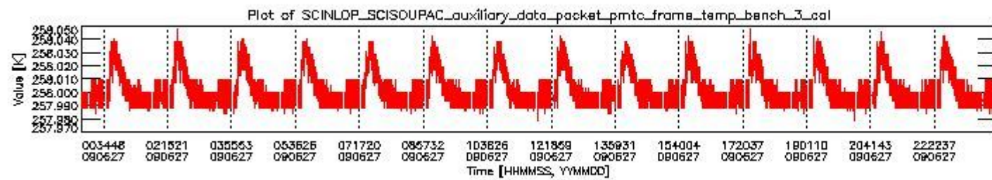
sciamachy_daily_report_level0_KSPT_L0_4303_N_20090627_2.PNG
