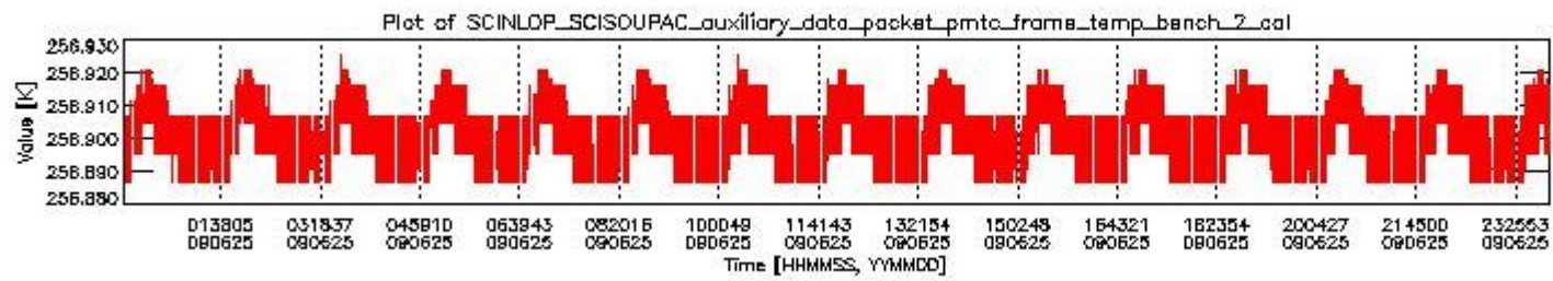
sciamachy_daily_report_level0_KSPT_L0_4303_N_20090625_1.PNG
