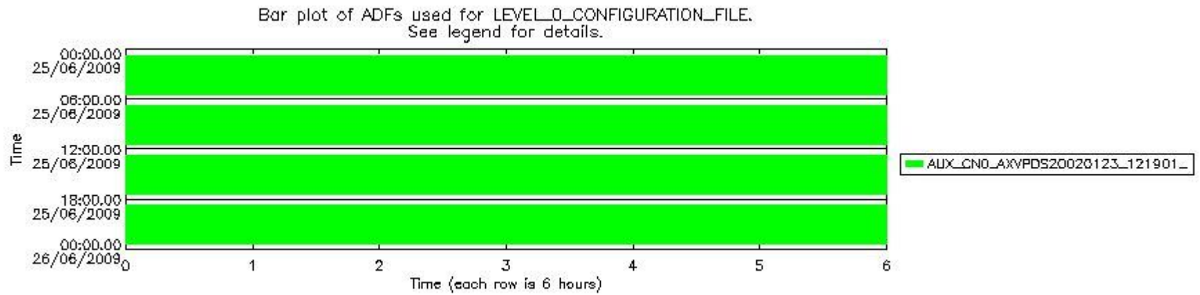
sciamachy_daily_report_level0_KSPT_L0_4303_N_20090625_6.PNG
