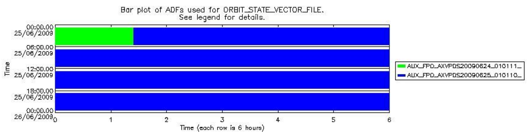
sciamachy_daily_report_level0_KSPT_L0_4303_N_20090625_7.PNG
