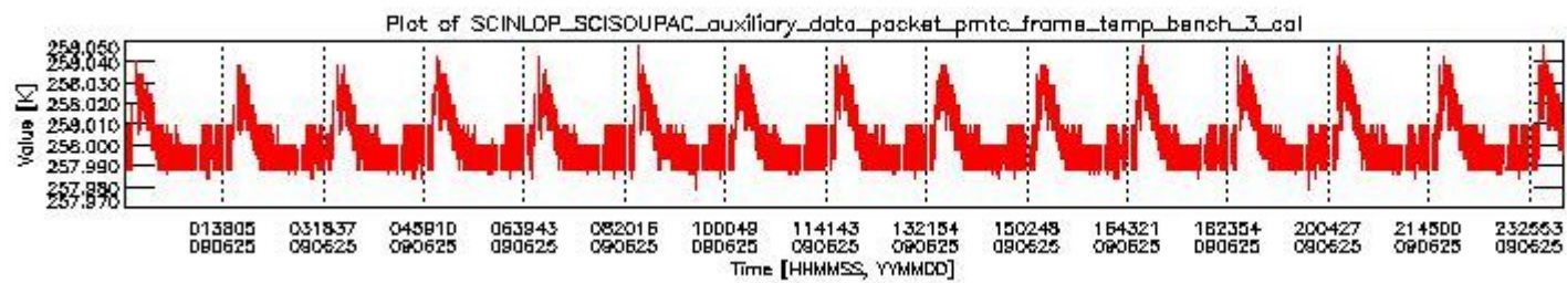
sciamachy_daily_report_level0_KSPT_L0_4303_N_20090625_2.PNG
