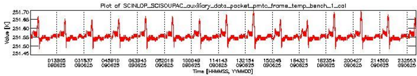
sciamachy_daily_report_level0_KSPT_L0_4303_N_20090625_0.PNG
