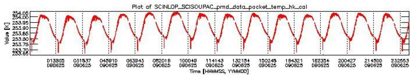
sciamachy_daily_report_level0_KSPT_L0_4303_N_20090625_3.PNG
