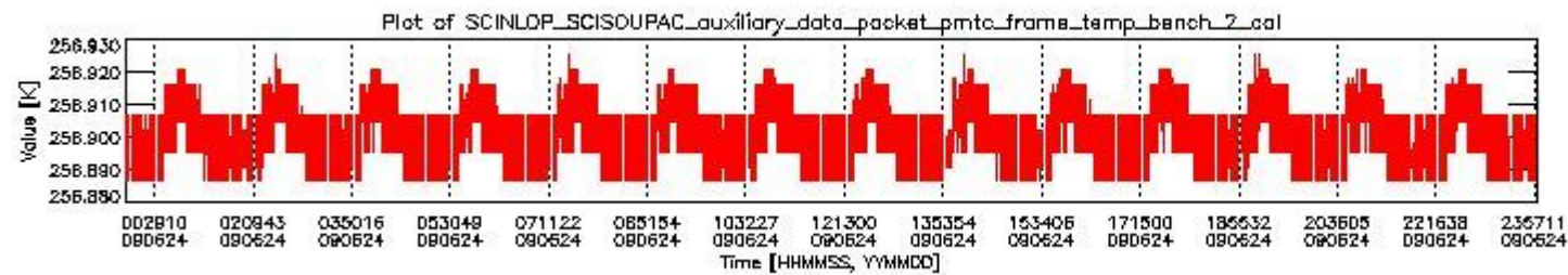
sciamachy_daily_report_level0_KSPT_L0_4303_N_20090624_1.PNG
