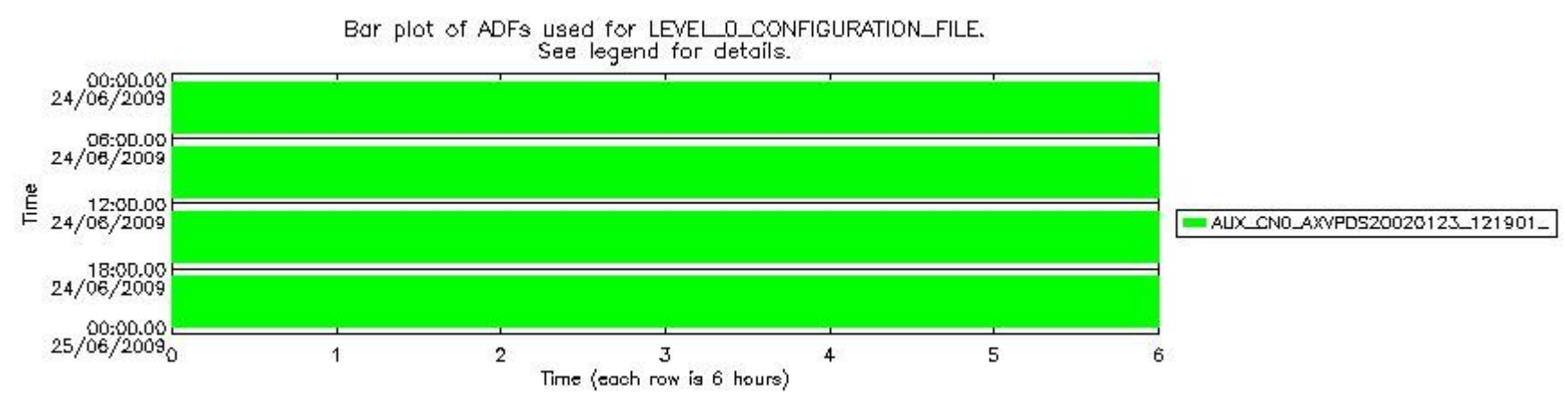
sciamachy_daily_report_level0_KSPT_L0_4303_N_20090624_6.PNG
