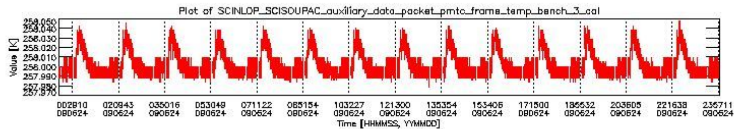
sciamachy_daily_report_level0_KSPT_L0_4303_N_20090624_2.PNG
