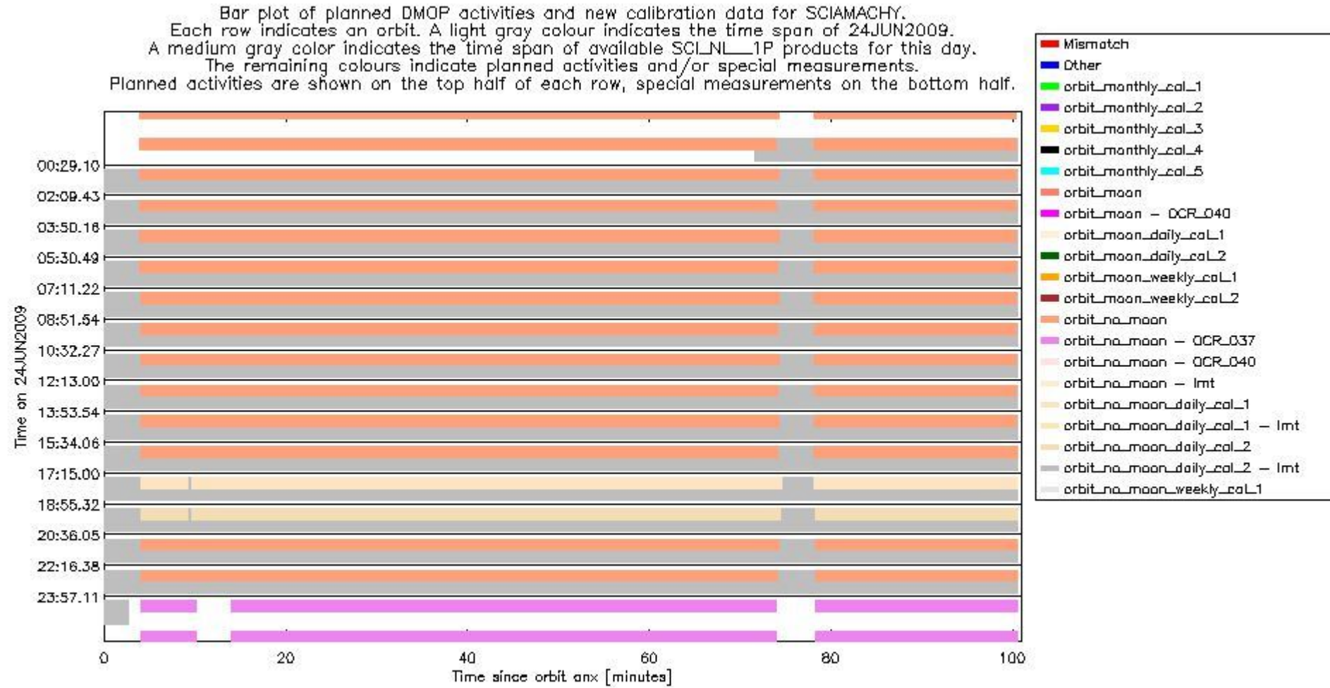
sciamachy_daily_report_level0_KSPT_L0_4303_N_20090624_5.PNG
