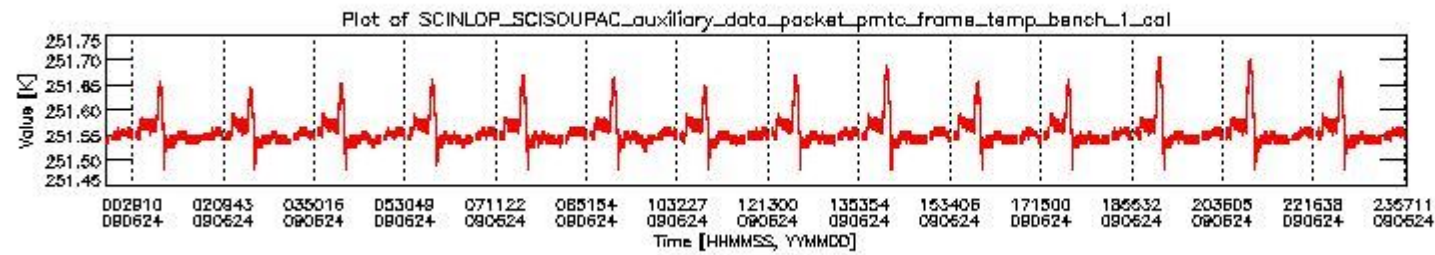
sciamachy_daily_report_level0_KSPT_L0_4303_N_20090624_0.PNG
