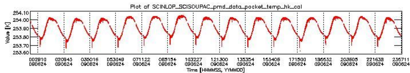
sciamachy_daily_report_level0_KSPT_L0_4303_N_20090624_3.PNG
