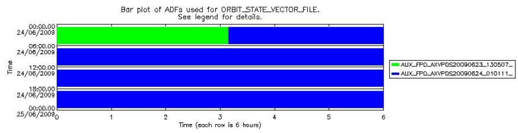
sciamachy_daily_report_level0_KSPT_L0_4303_N_20090624_7.PNG
