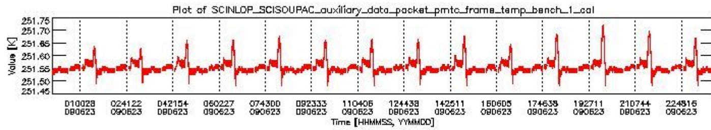
sciamachy_daily_report_level0_KSPT_L0_4303_N_20090623_0.PNG
