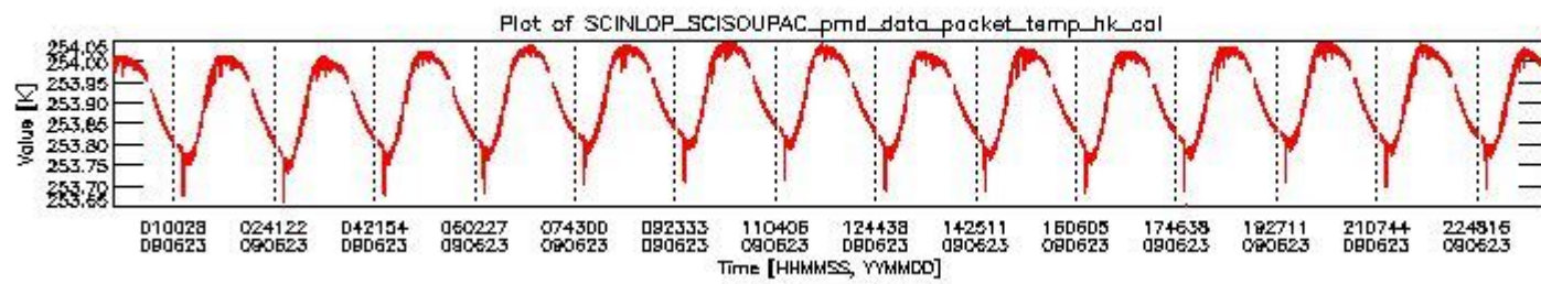
sciamachy_daily_report_level0_KSPT_L0_4303_N_20090623_3.PNG
