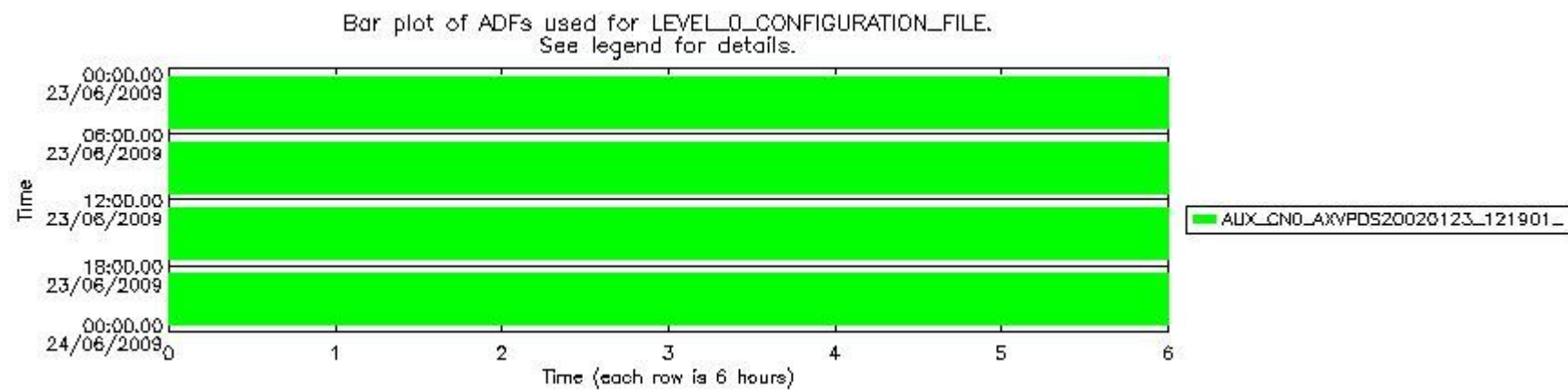
sciamachy_daily_report_level0_KSPT_L0_4303_N_20090623_6.PNG
