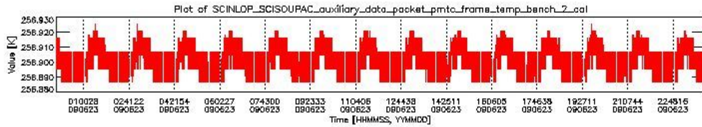
sciamachy_daily_report_level0_KSPT_L0_4303_N_20090623_1.PNG
