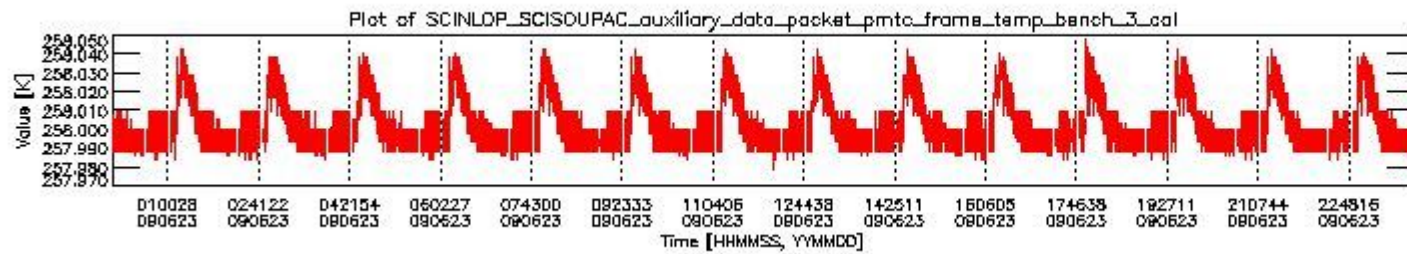
sciamachy_daily_report_level0_KSPT_L0_4303_N_20090623_2.PNG
