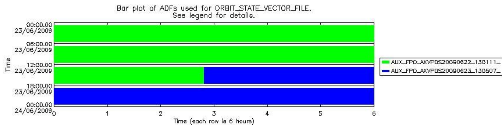
sciamachy_daily_report_level0_KSPT_L0_4303_N_20090623_7.PNG
