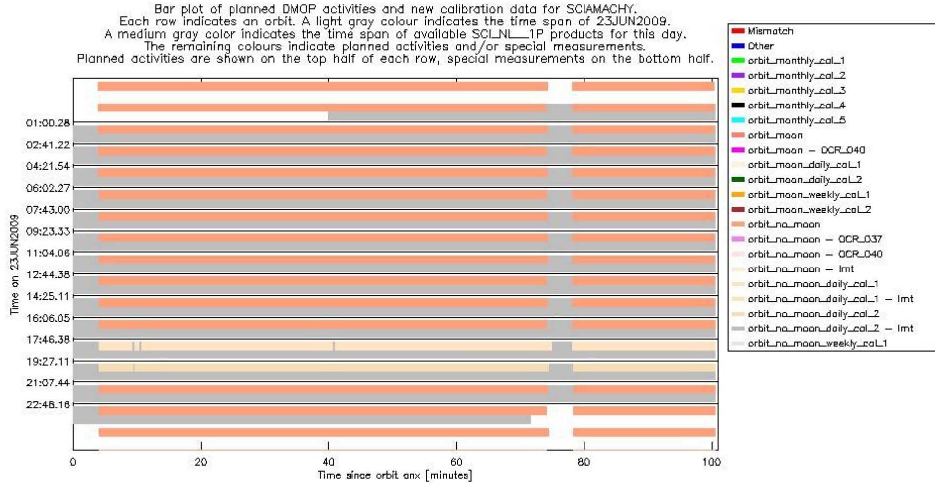
sciamachy_daily_report_level0_KSPT_L0_4303_N_20090623_5.PNG
