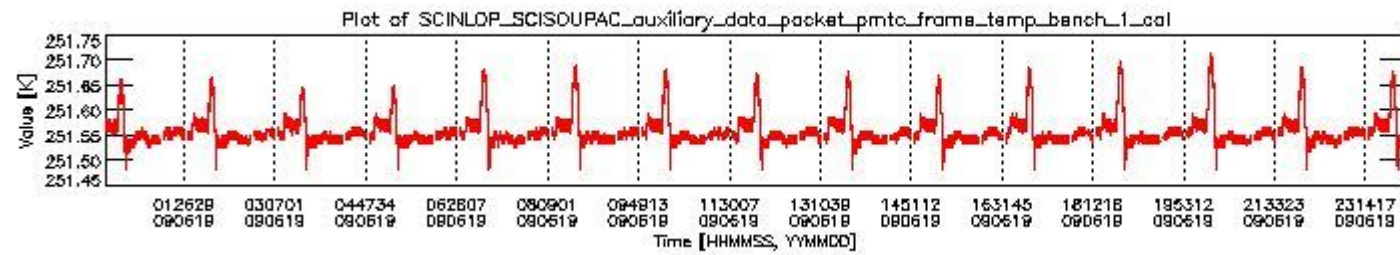
sciamachy_daily_report_level0_KSPT_L0_4303_N_20090619_0.PNG
