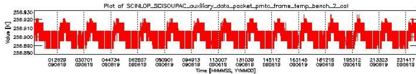
sciamachy_daily_report_level0_KSPT_L0_4303_N_20090619_1.PNG
