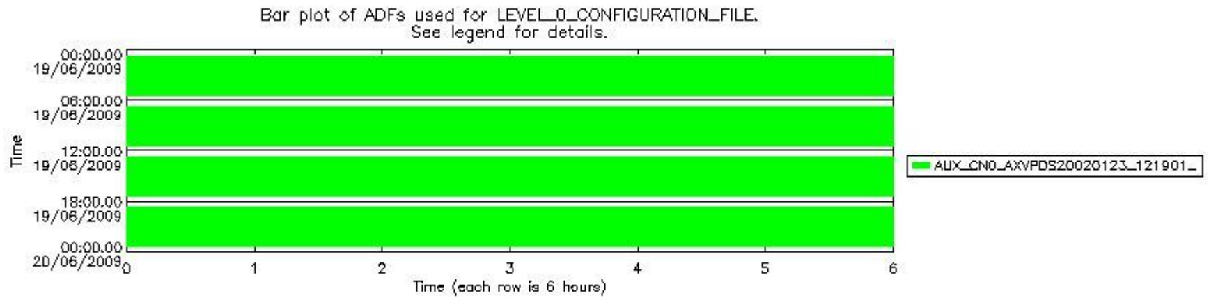
sciamachy_daily_report_level0_KSPT_L0_4303_N_20090619_6.PNG
