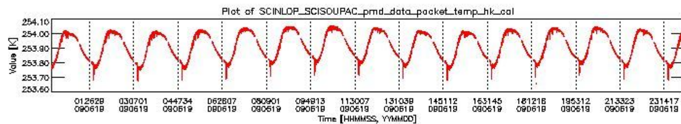
sciamachy_daily_report_level0_KSPT_L0_4303_N_20090619_3.PNG
