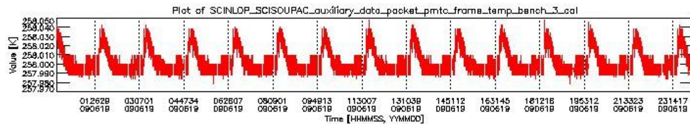
sciamachy_daily_report_level0_KSPT_L0_4303_N_20090619_2.PNG
