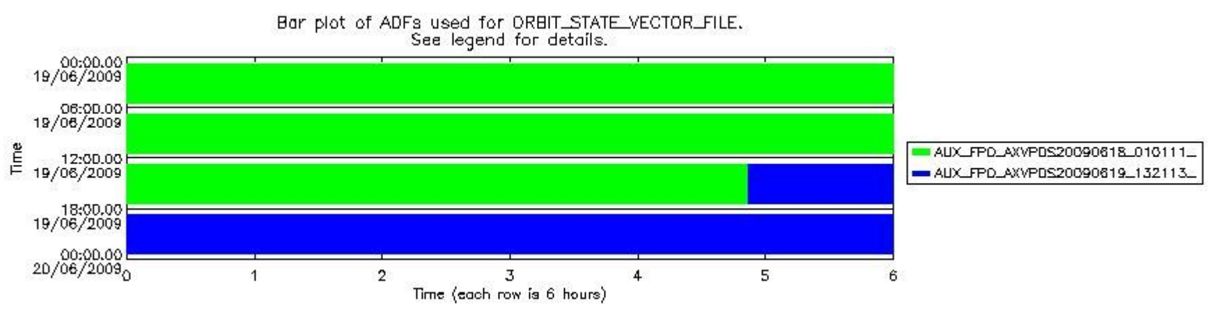
sciamachy_daily_report_level0_KSPT_L0_4303_N_20090619_7.PNG
