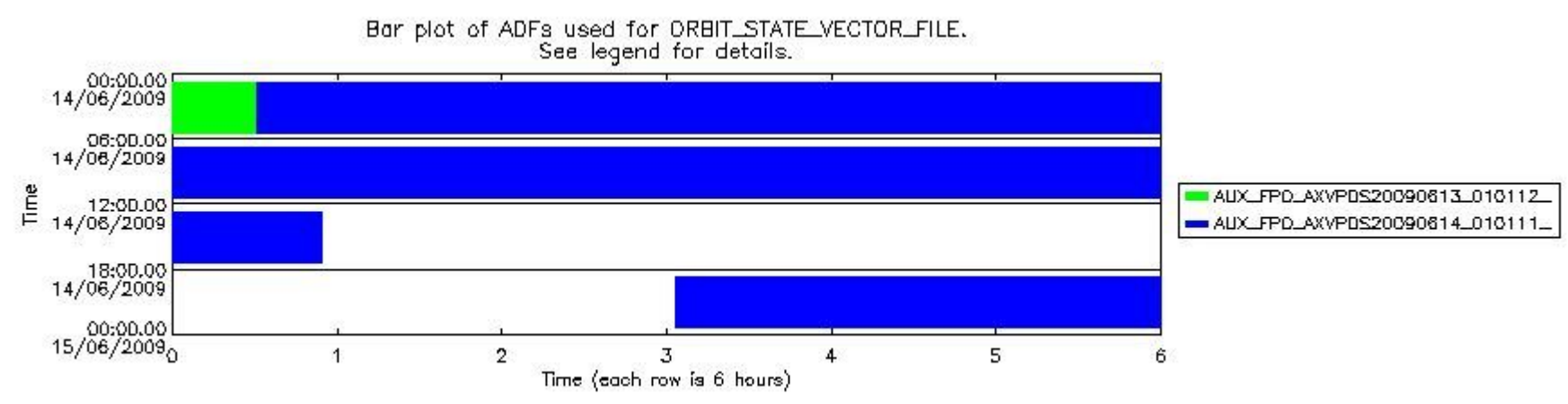
sciamachy_daily_report_level0_KSPT_L0_4303_N_20090614_8.PNG
