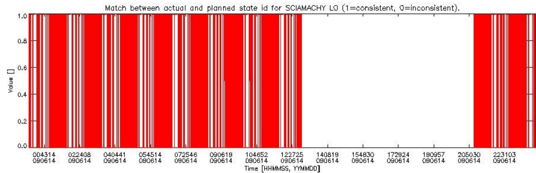
sciamachy_daily_report_level0_KSPT_L0_4303_N_20090614_5.PNG
