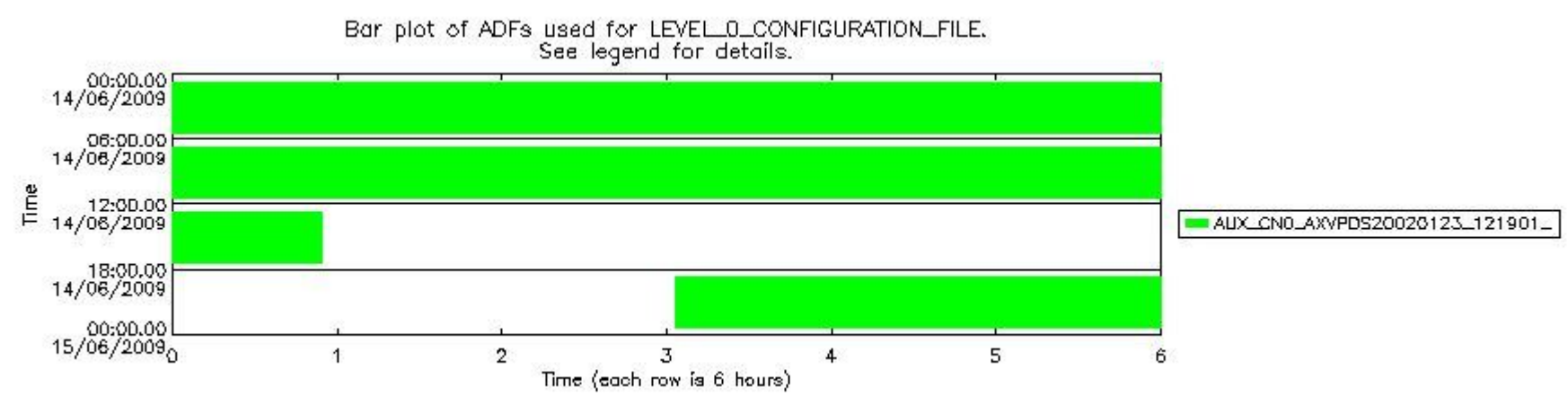
sciamachy_daily_report_level0_KSPT_L0_4303_N_20090614_7.PNG
