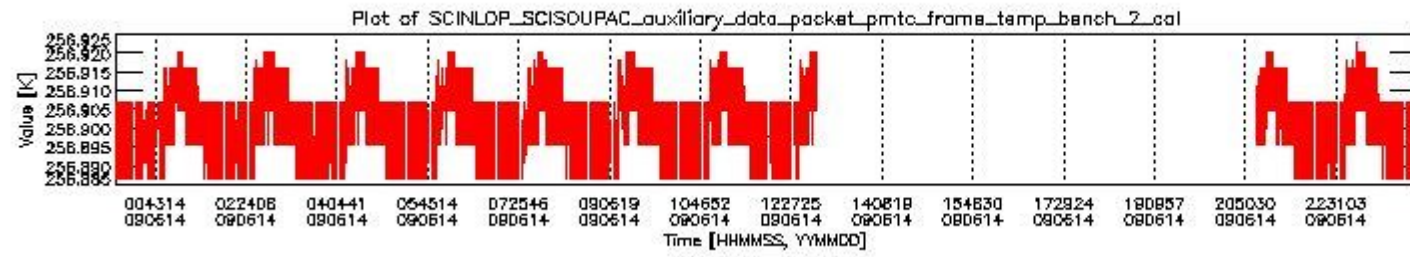
sciamachy_daily_report_level0_KSPT_L0_4303_N_20090614_1.PNG
