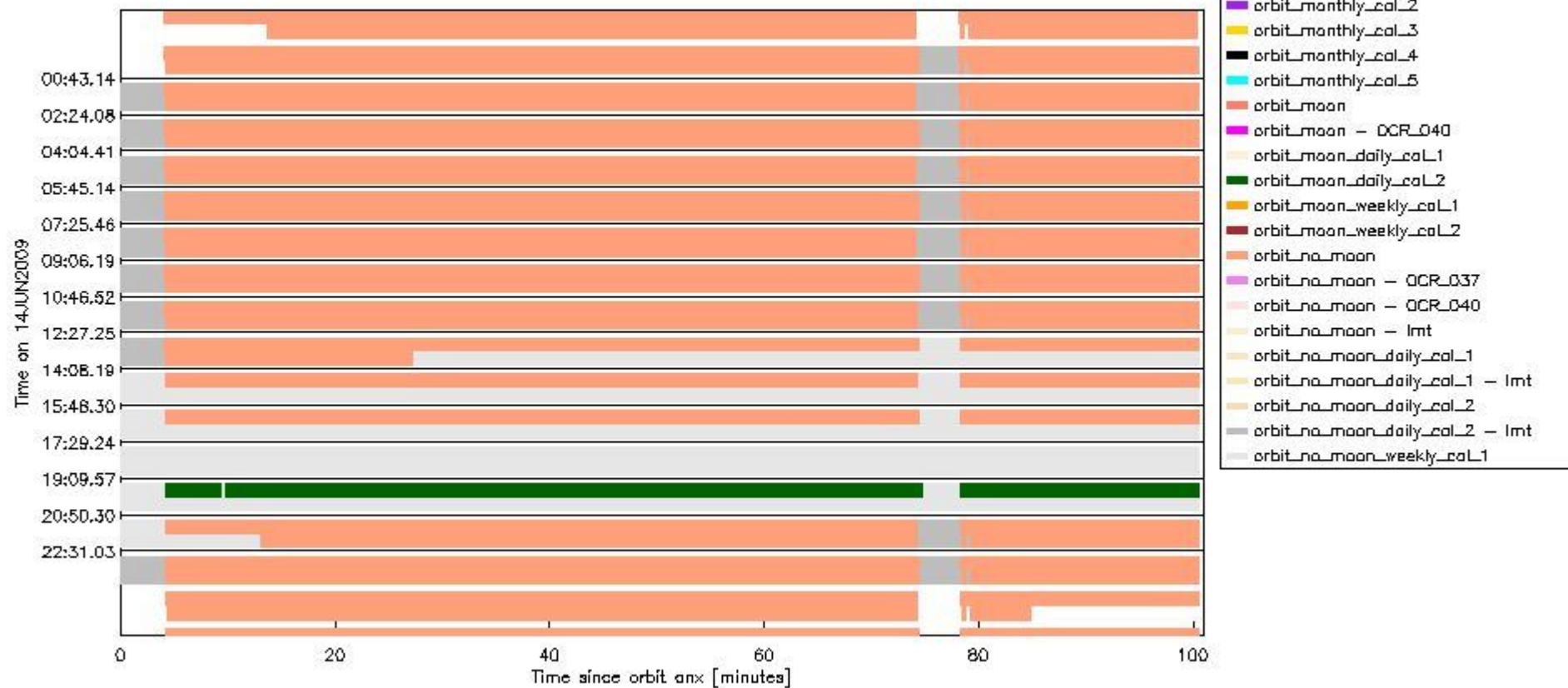
sciamachy_daily_report_level0_KSPT_L0_4303_N_20090614_6.PNG
