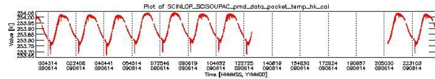
sciamachy_daily_report_level0_KSPT_L0_4303_N_20090614_3.PNG
