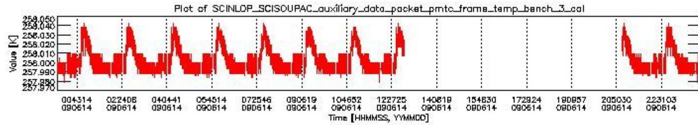
sciamachy_daily_report_level0_KSPT_L0_4303_N_20090614_2.PNG
