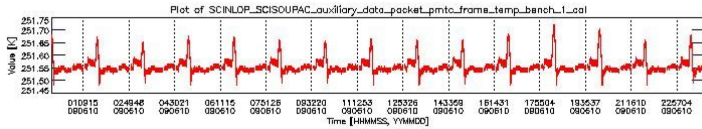
sciamachy_daily_report_level0_KSPT_L0_4303_N_20090610_0.PNG
