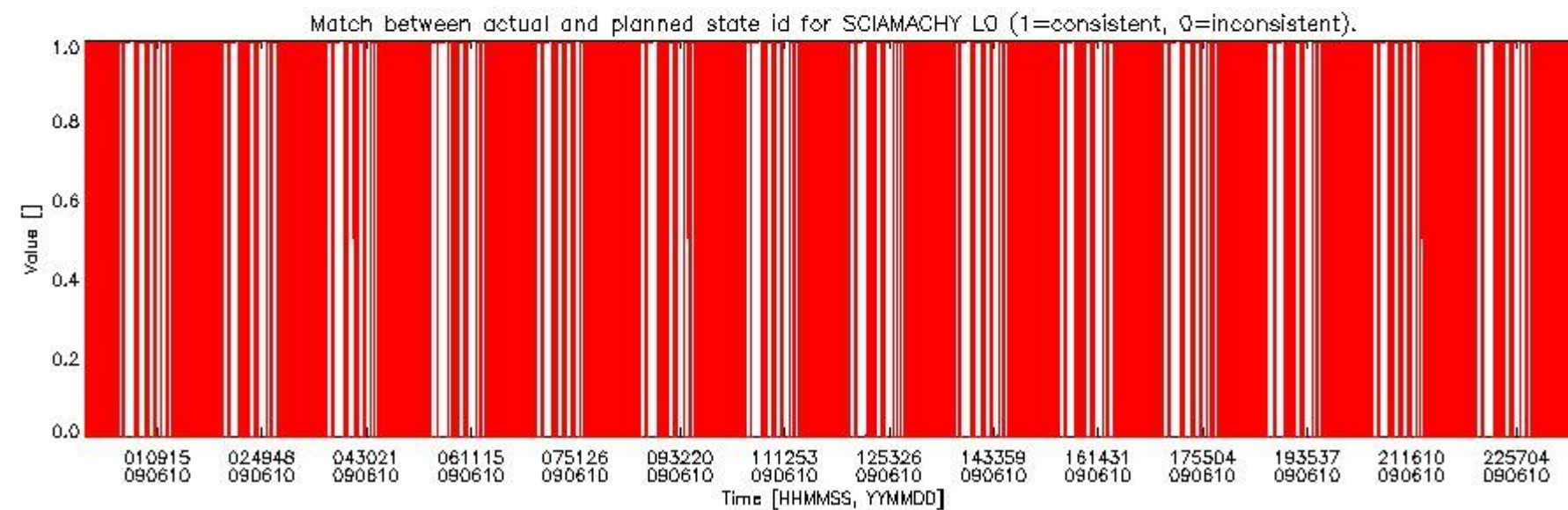
sciamachy_daily_report_level0_KSPT_L0_4303_N_20090610_5.PNG
