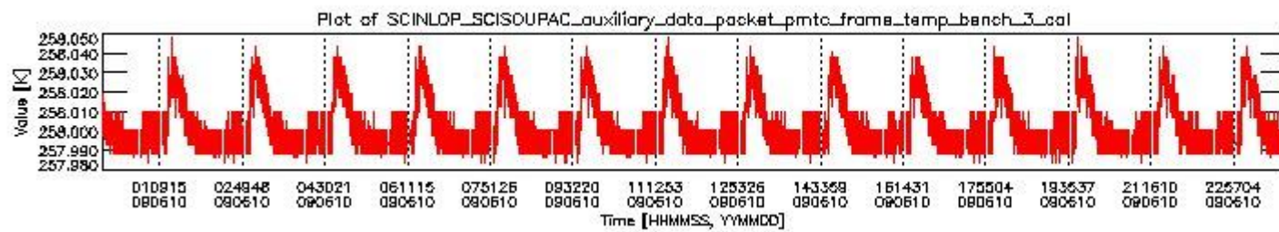
sciamachy_daily_report_level0_KSPT_L0_4303_N_20090610_2.PNG
