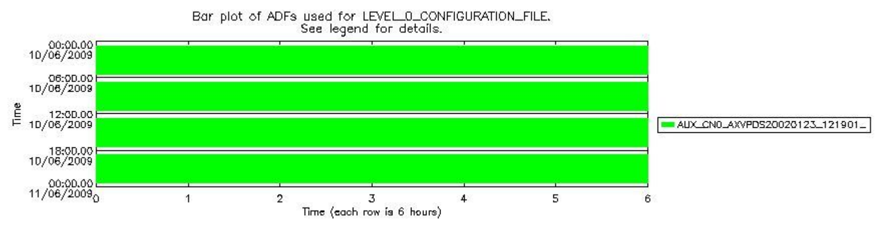
sciamachy_daily_report_level0_KSPT_L0_4303_N_20090610_7.PNG
