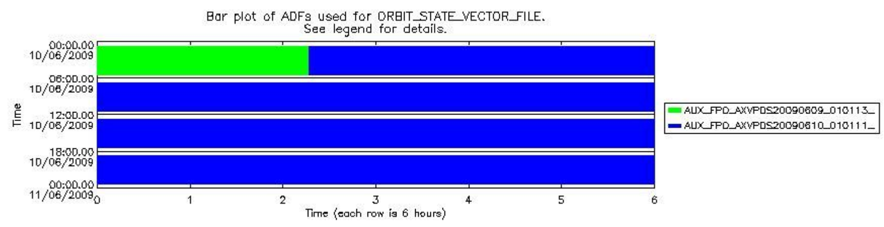
sciamachy_daily_report_level0_KSPT_L0_4303_N_20090610_8.PNG
