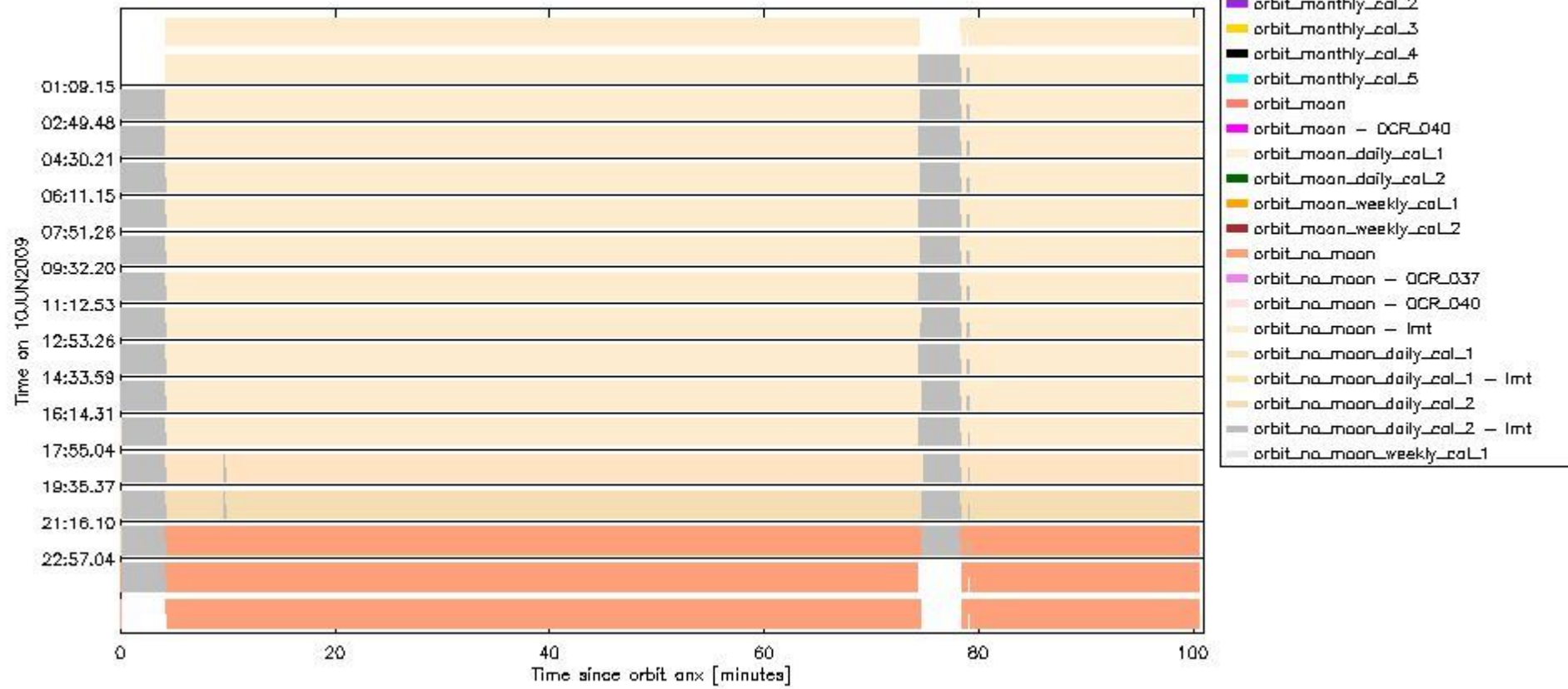
sciamachy_daily_report_level0_KSPT_L0_4303_N_20090610_6.PNG
