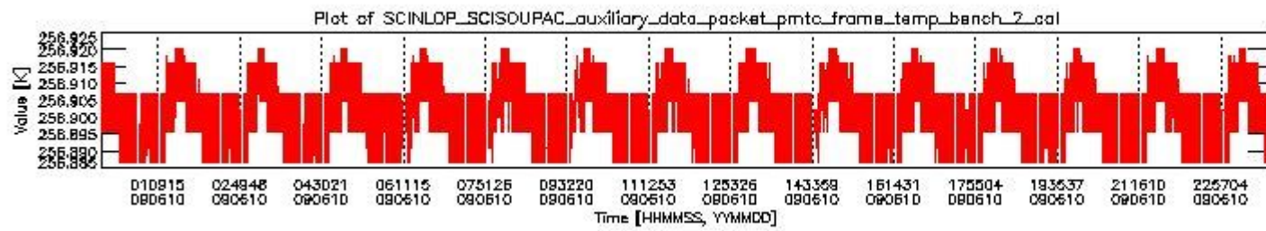
sciamachy_daily_report_level0_KSPT_L0_4303_N_20090610_1.PNG
