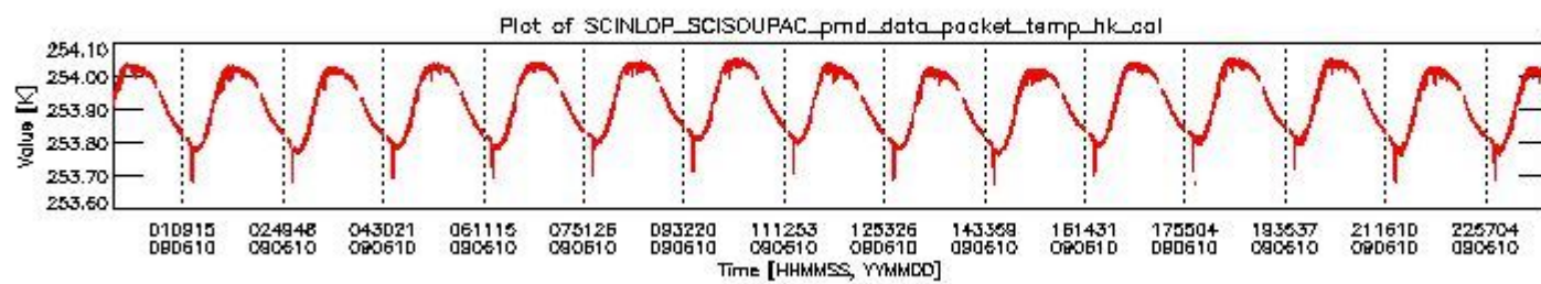
sciamachy_daily_report_level0_KSPT_L0_4303_N_20090610_3.PNG
